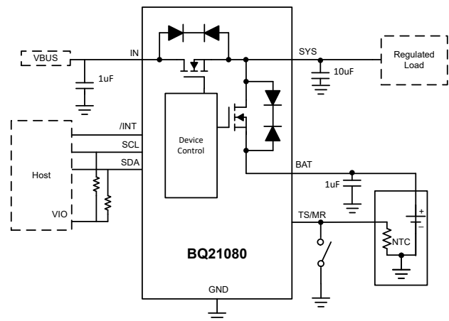
简化原理图
