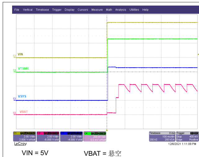
图 9-2. 在没有电池的情况下通过插入 IN 电源进行上电
