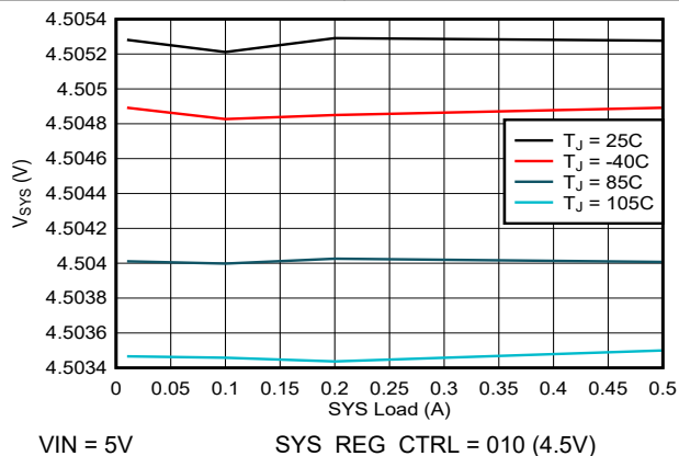
图 7-5. SYS 负载调节与温度间的关系
