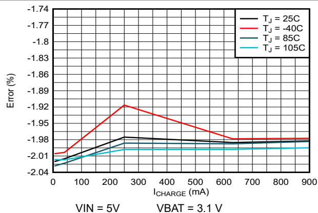
图 7-2. 充电电流精度与 ICHARGE 设置间的关系
