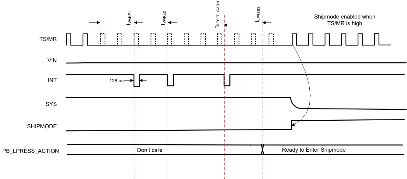
图 8-5. 按钮长按运输模式
