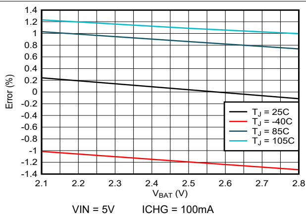
图 7-3. 预充电精度与电池电压间的关系
