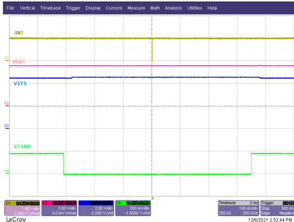
图 9-15. 存在 VIN 时的 Wake1 中断
