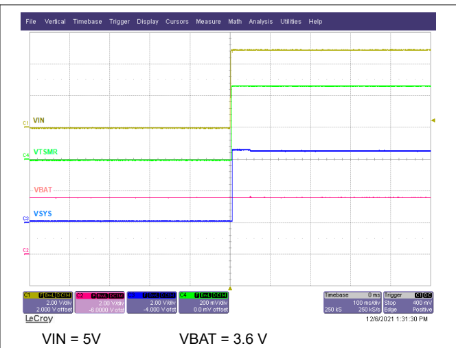
图 9-3. 通过插入 VIN 电源从关断模式上电
