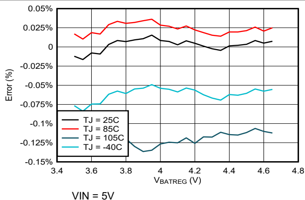
图 7-1. 电池调节电压精度与 VBATREG 设置间的关系
