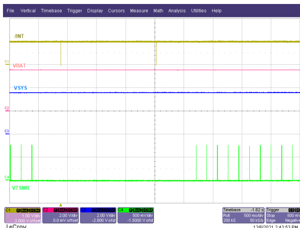
图 9-17. 存在 VIN 时的长按中断
