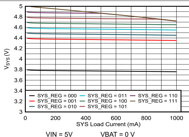
图 7-4. SYS 负载调节
