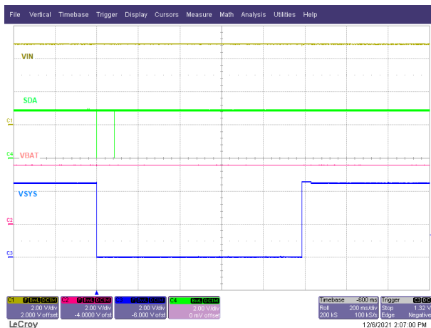
图 9-8. 通过 I 2 C 进行硬件复位
