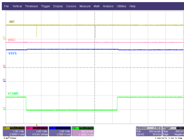
图 9-14. SYS 模式扫描
