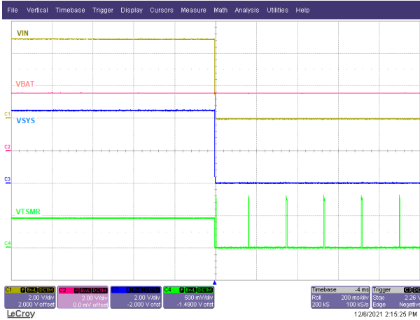
图 9-10. 移除 VIN 时进入运输模式
