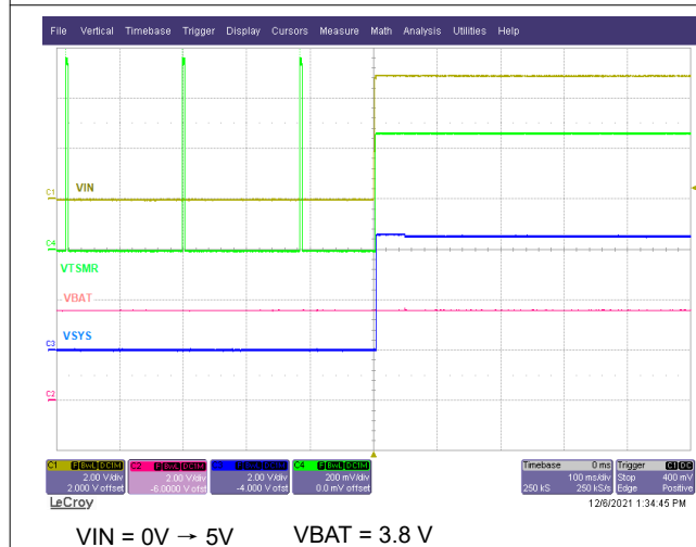
图 9-4. 通过插入 VIN 从运输模式上电
