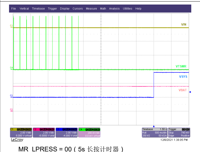
图 9-5. 通过按下 /TSMR 按钮从运输模式上电
