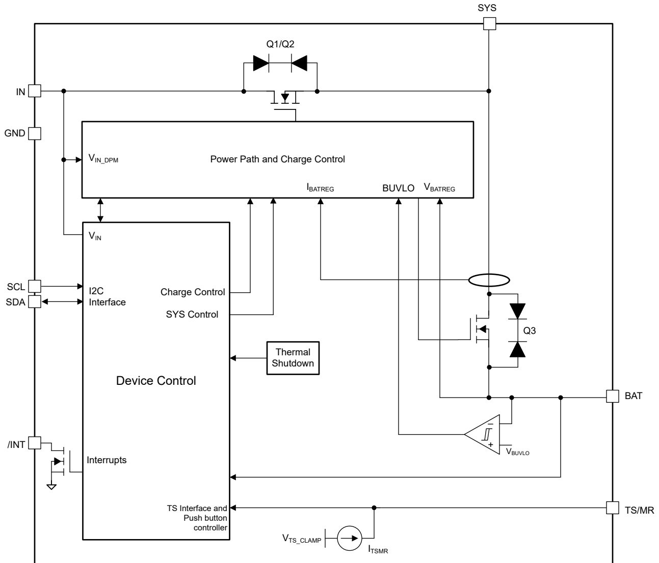
图 8-3. 功能方框图
