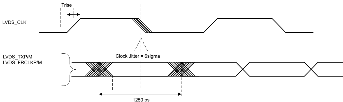
图 7-14. 计时参数
