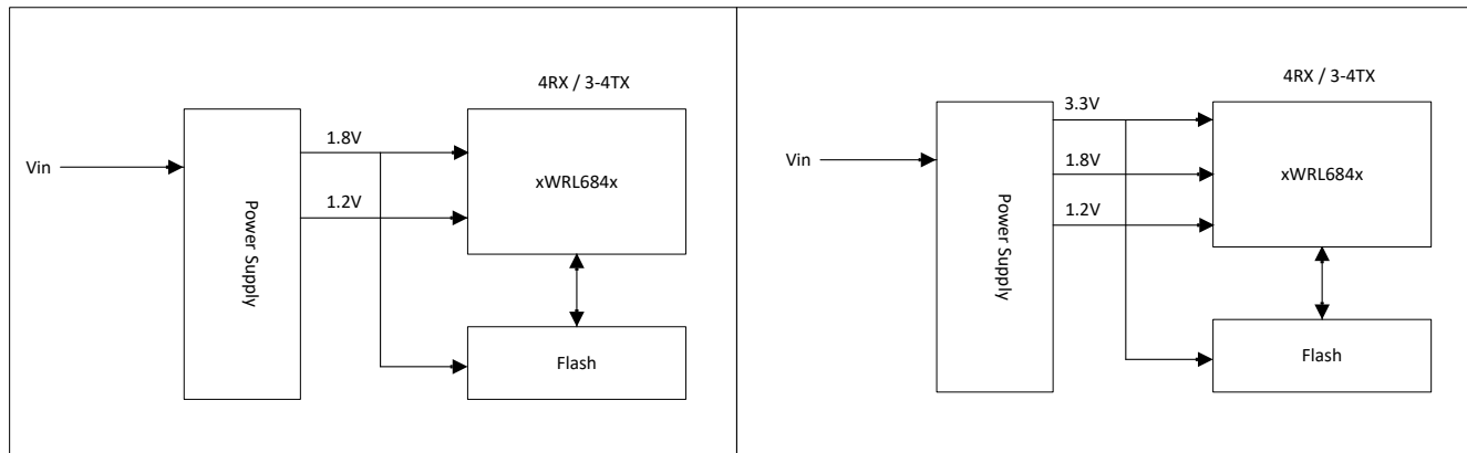
图 7-2. I/O 拓扑（左图：1.8V I/O 拓扑，右图：3.3V I/O 拓扑）
