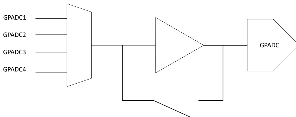
图 8-7. GPADC 路径
