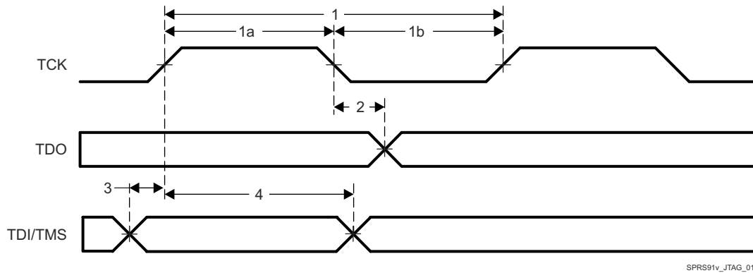
图 7-18. JTAG 时序
