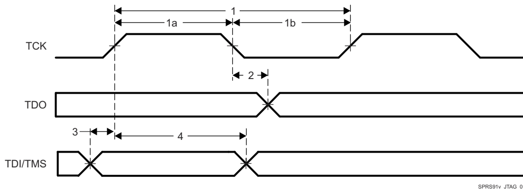
图 8-22. JTAG Timing
