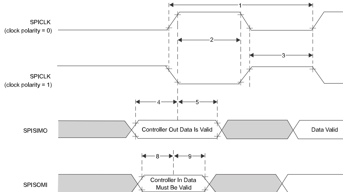
图 7-9. SPI 控制器模式外部时序 (时钟相位 = 1)
