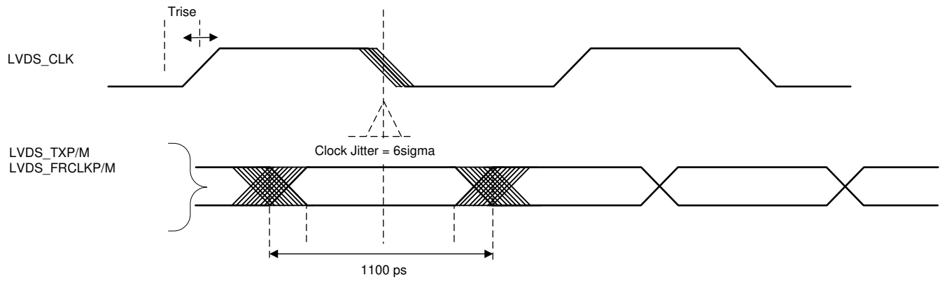
图 8-14. Timing Parameters
