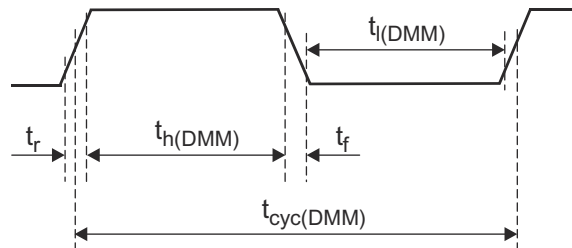
图 8-20. DMMCLK Timing
