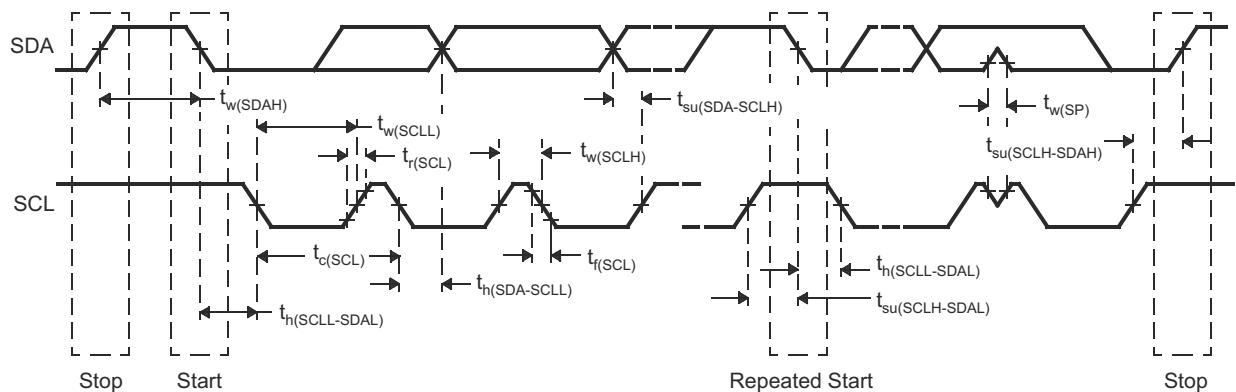
图 7-23. I2C 时序图
