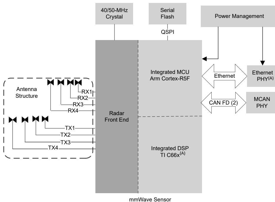
图 2-1. 适用于汽车应用的自主雷达传感器
