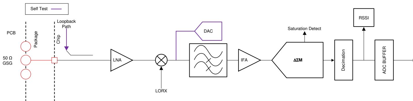
图 8-4. 接收子系统 (每通道)
