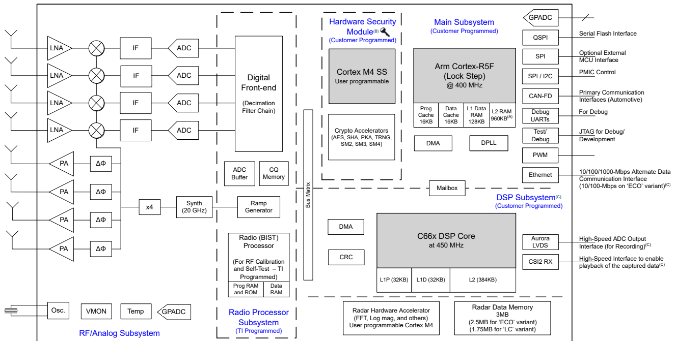
图 8-1. 功能方框图
