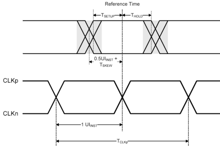
图 7-24. HS 发送模式下的时钟和数据时序
