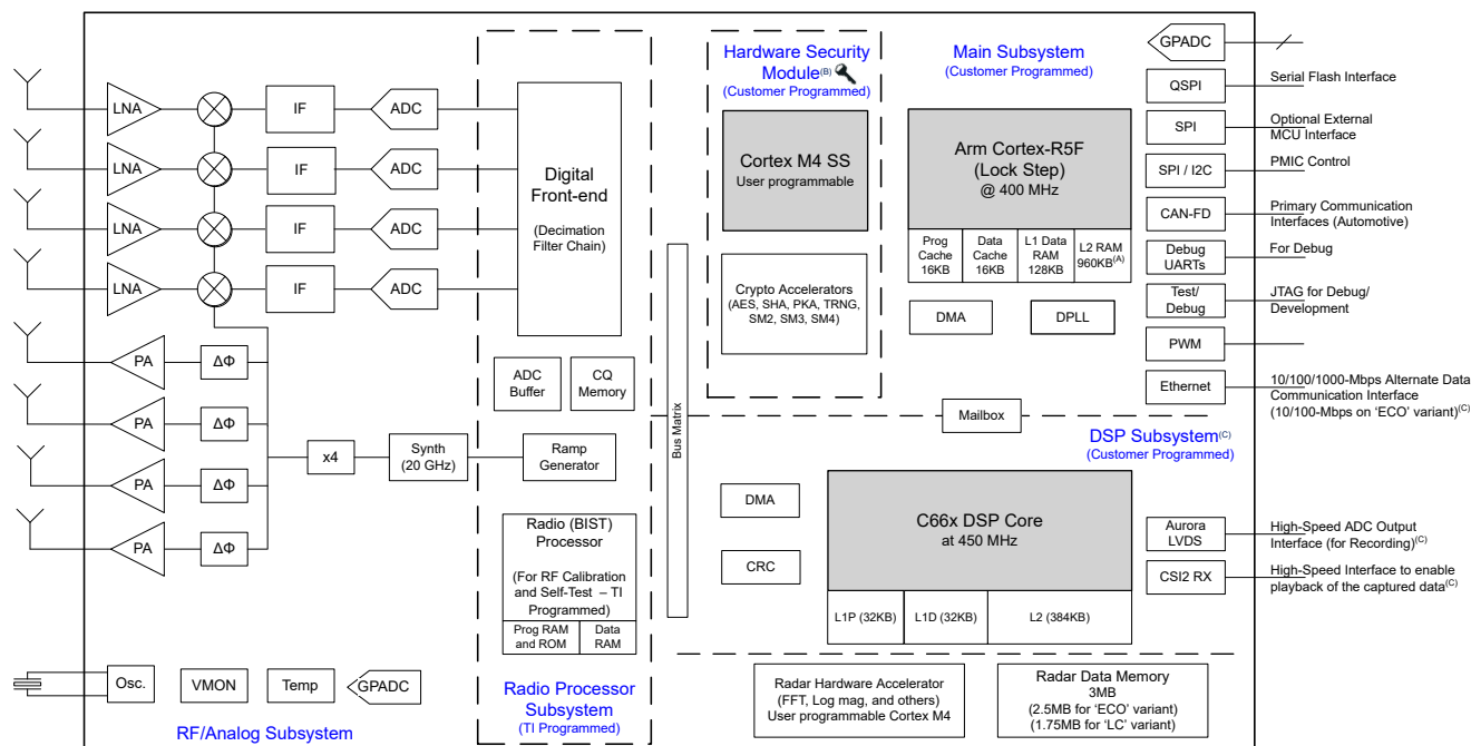
图 3-1. 功能方框图
