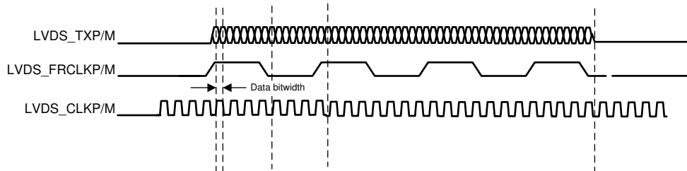
图 7-21. LVDS 接口通道配置和相关时序
