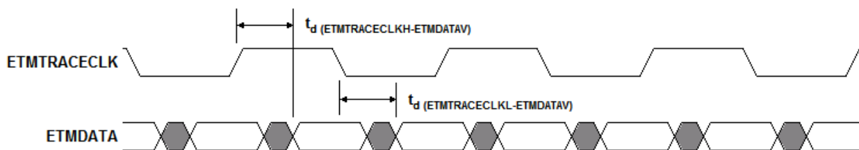
图 7-27. ETMDATA 时序
