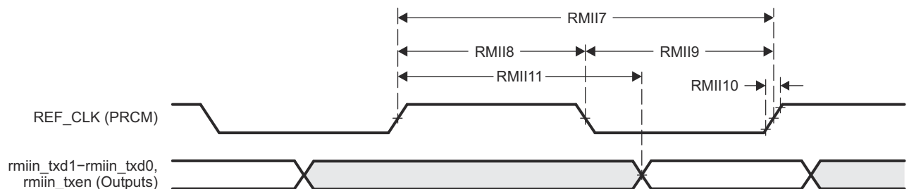
图 7-14. MAC 发送接口时序，RMII n 运行模式
