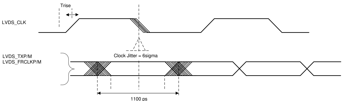
图 7-22. 计时参数
