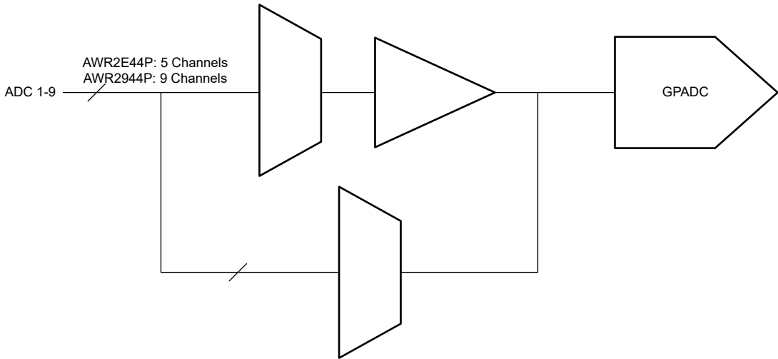
图 8-6. GPADC 路径
