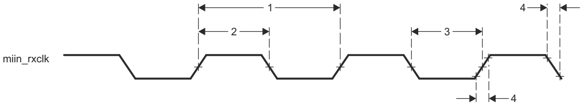
图 7-19. 时钟时序 (MAC 接收) — MII 运行模式
