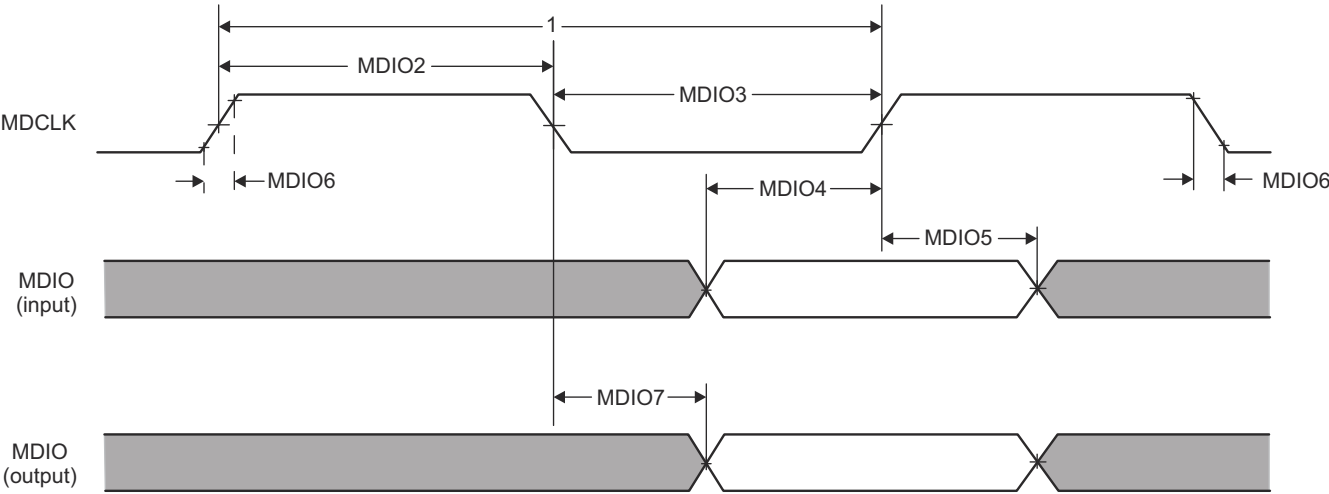
图 7-20. MAC MDIO 图表
