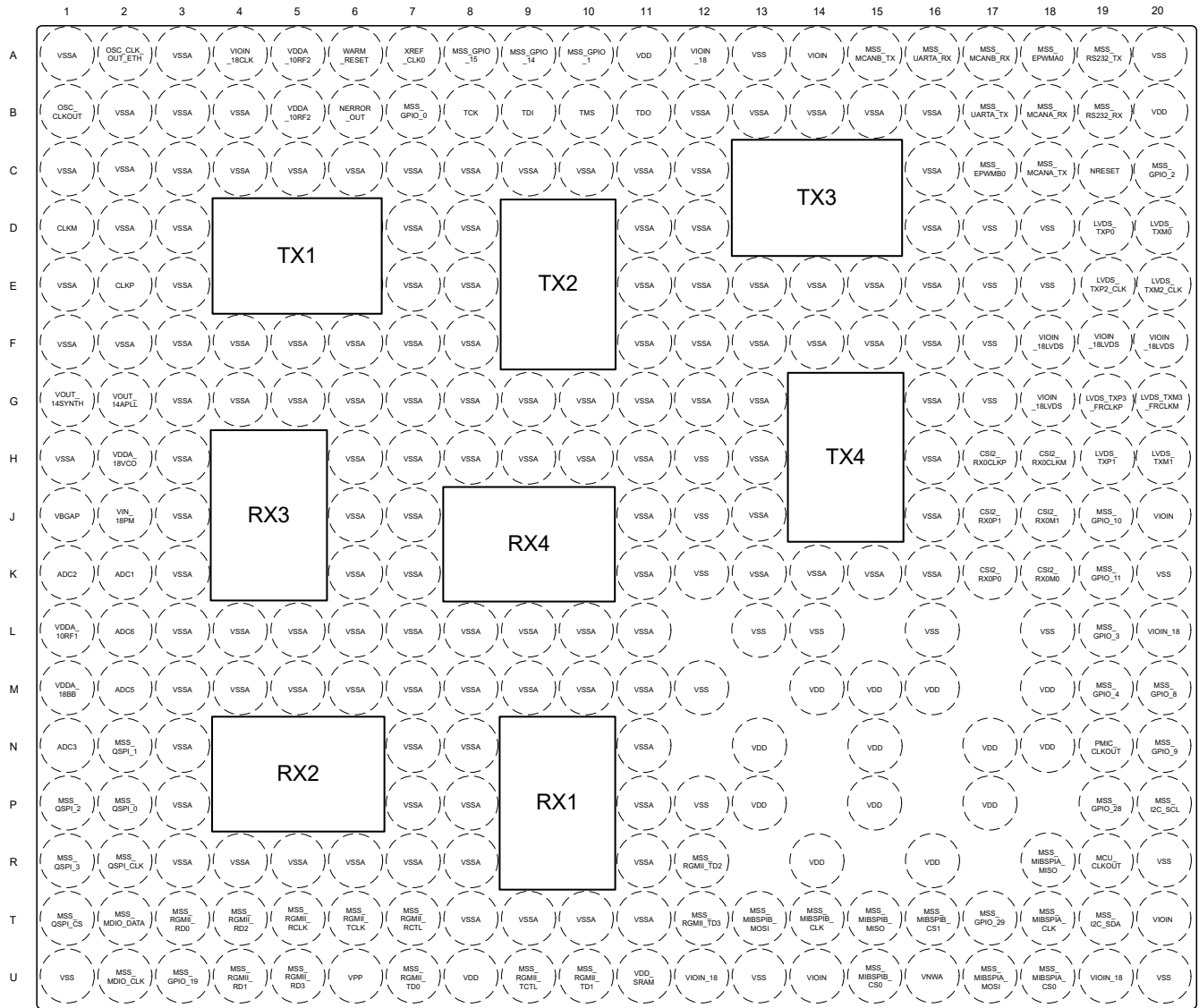
图 6-2. 引脚图 - AWR2E44P/AWR2E44-ECO/AWR2E44LC
