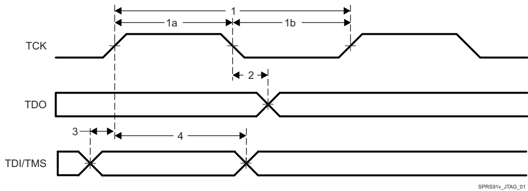
图 7-25. JTAG 时序
