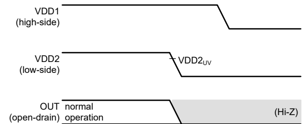
图 6-10. VDD2 和 VDD1 先后关闭
