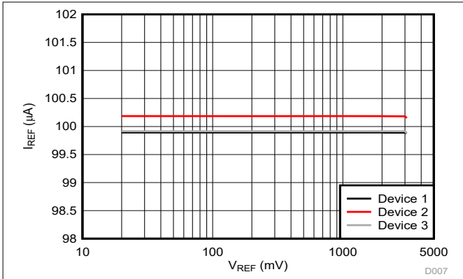
图 5-39. 基准电流与基准电压间的关系
