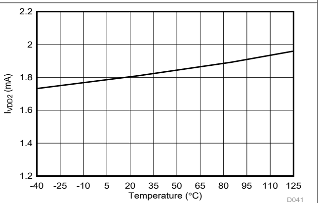
图 5-42. 高侧电源电流与温度间的关系
