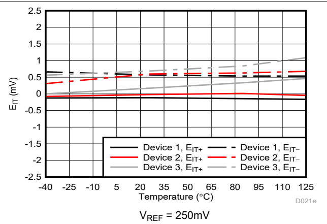
图 5-12. Cmp0 跳变阈值误差与温度间的关系
