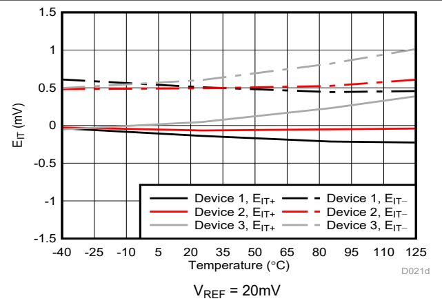
图 5-6. Cmp0 跳变阈值误差与温度间的关系
