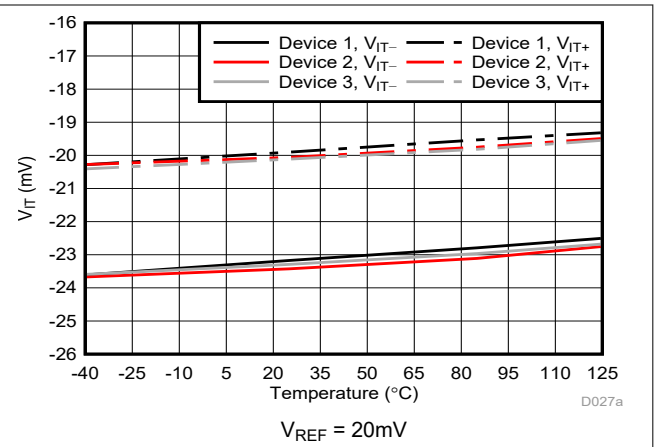
图 5-22. Cmp1 跳变阈值与温度间的关系
