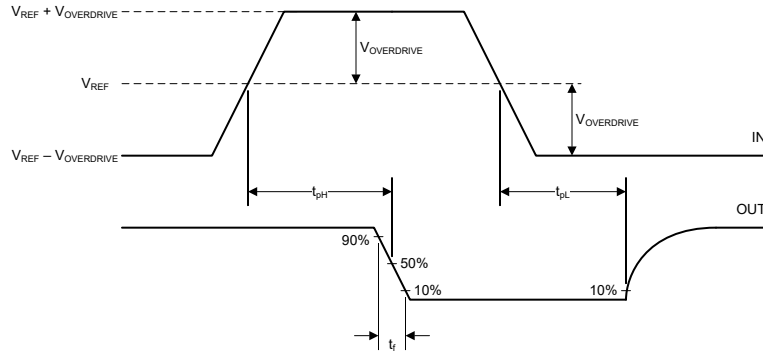
图 5-1. 上升、下降和延迟时间定义 (LATCH = 低电平)
