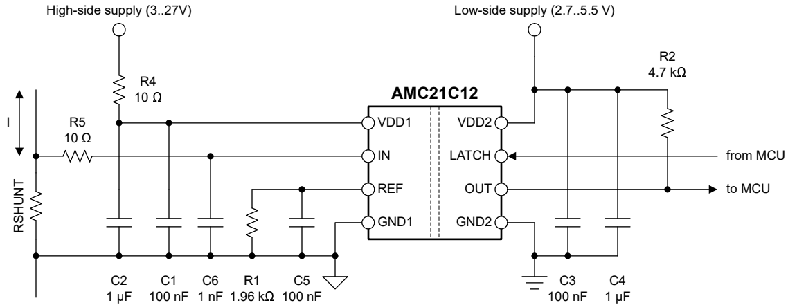
图 7-6. 去耦 AMC21C12
