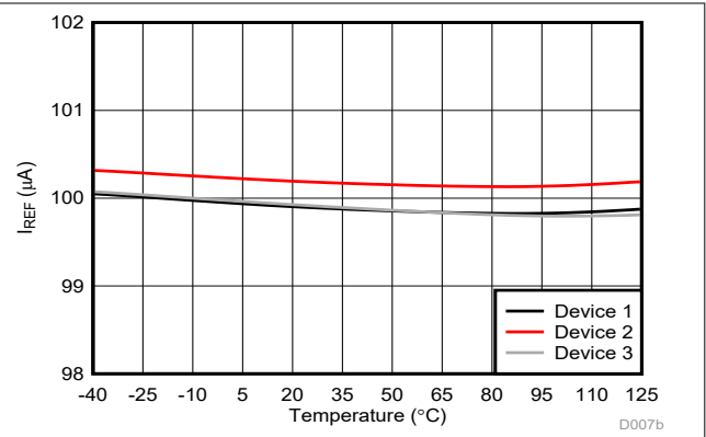
图 5-40. 基准电流与温度间的关系
