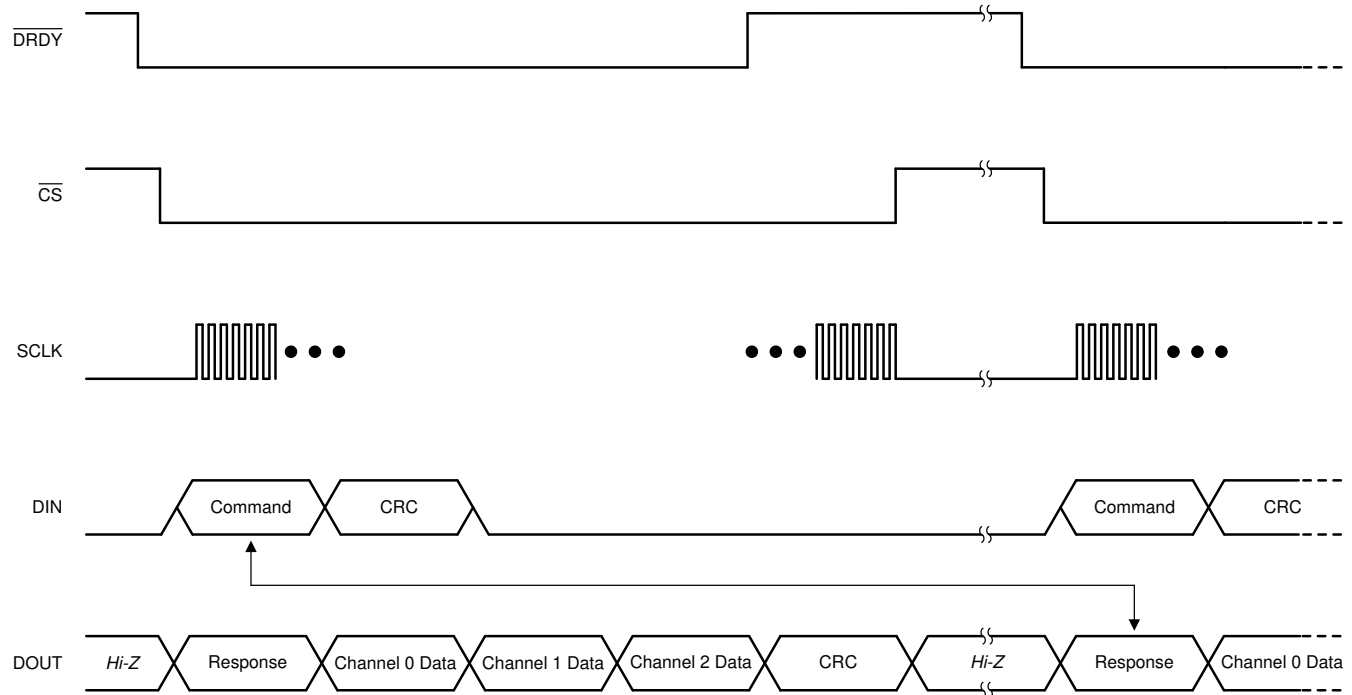
图 8-24. 典型通信帧
