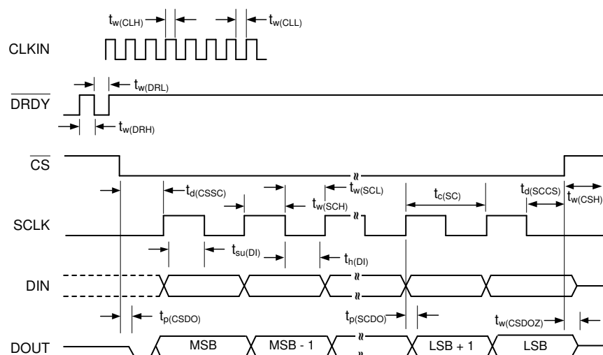
图 6-1. SPI 时序图
