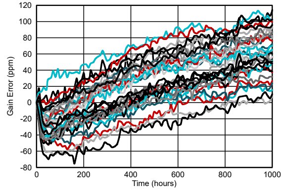
30 个单元, 85°C
