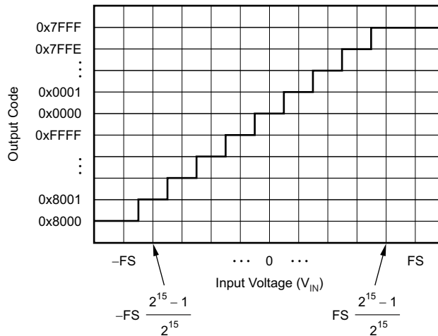
图 8-25. 代码转换图
