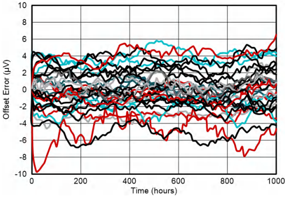
30 个单元, 85°C
