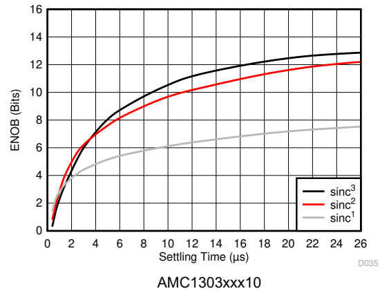
图 8-5. 测得的有效位数与建立时间间的关系
