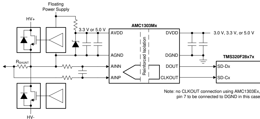
应用原理图
