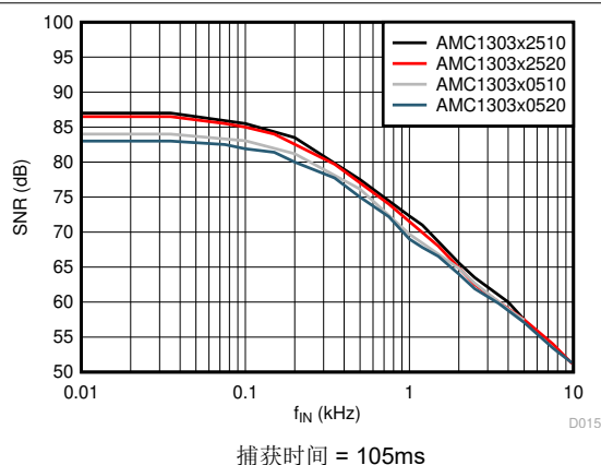
图 6-18. 信噪比与输入信号频率间的关系
