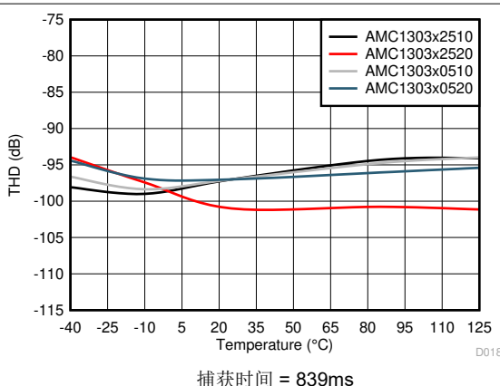
图 6-22. 总谐波失真与温度间的关系
