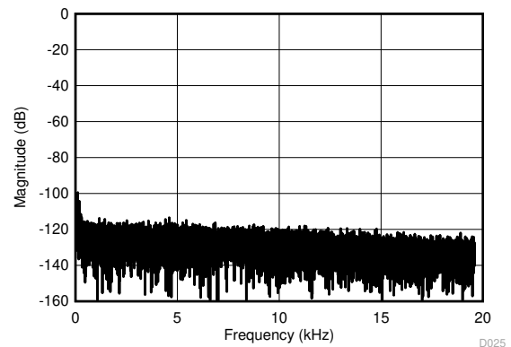
图 6-31. 35Hz 输入信号时的频谱
