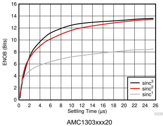
图 8-4. 测得的有效位数与建立时间间的关系
