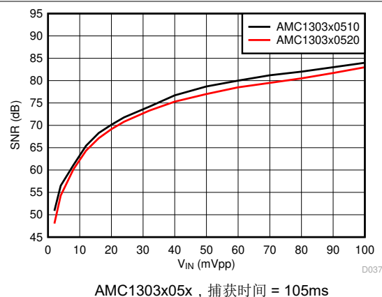
图 6-20. 信噪比与输入信号幅度间的关系
