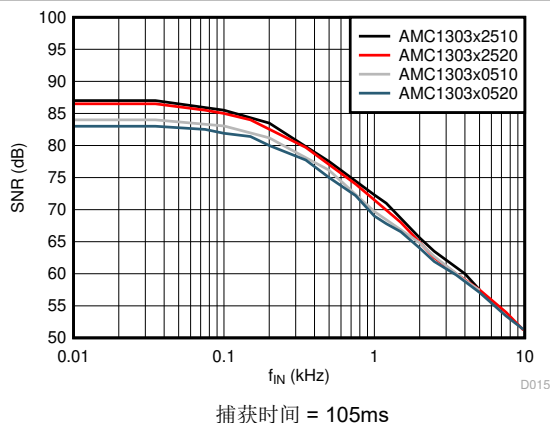
图 6-18. 信噪比与输入信号频率间的关系
