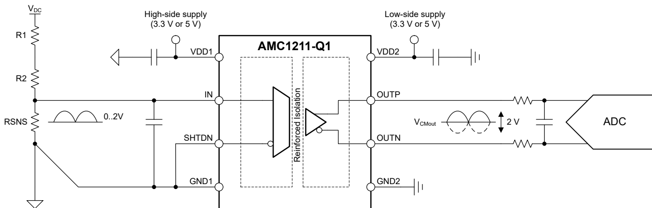
简化原理图
