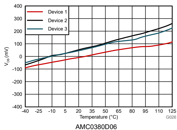
图 6-12. 输入失调电压与温度间的关系
