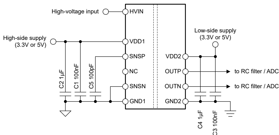
图 8-5. AMC0380D 去耦
