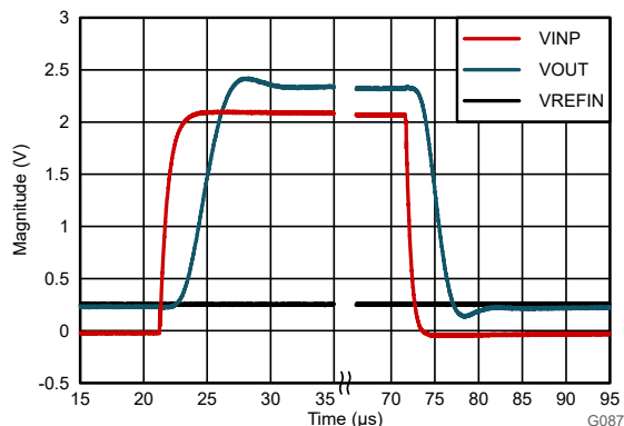
图 8-4. AMC0x11S 的阶跃响应
