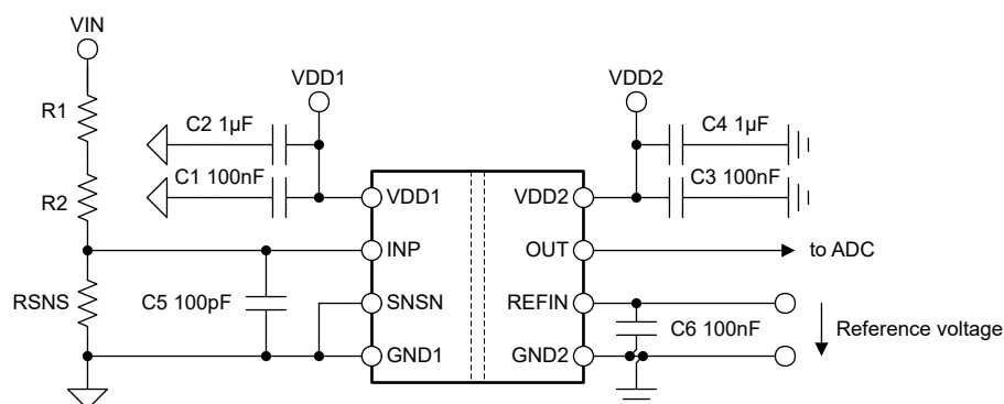
图 8-5. AMC0x11S 去耦
