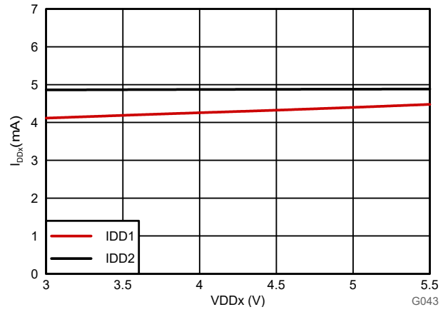
图 6-13. 电源电流与电源电压间的关系
