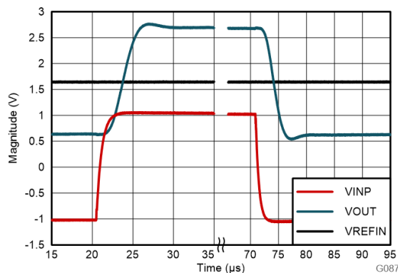
图 8-4. AMC0x30S-Q1 的阶跃响应
