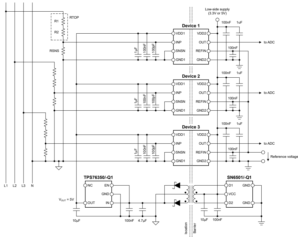
图 8-1. 在典型应用中使用 AMC0x30S
