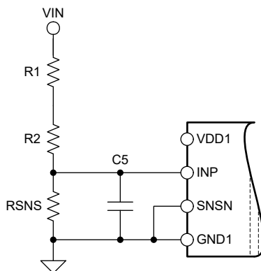
图 8-2. 输入滤波器
