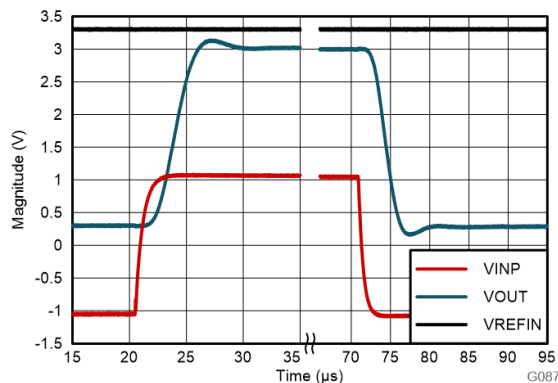
图 8-4. AMC0x30R 的阶跃响应
