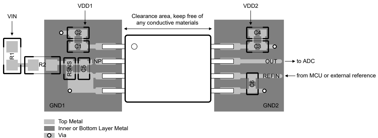
图 8-6. AMC0x11S-Q1 的建议布局
