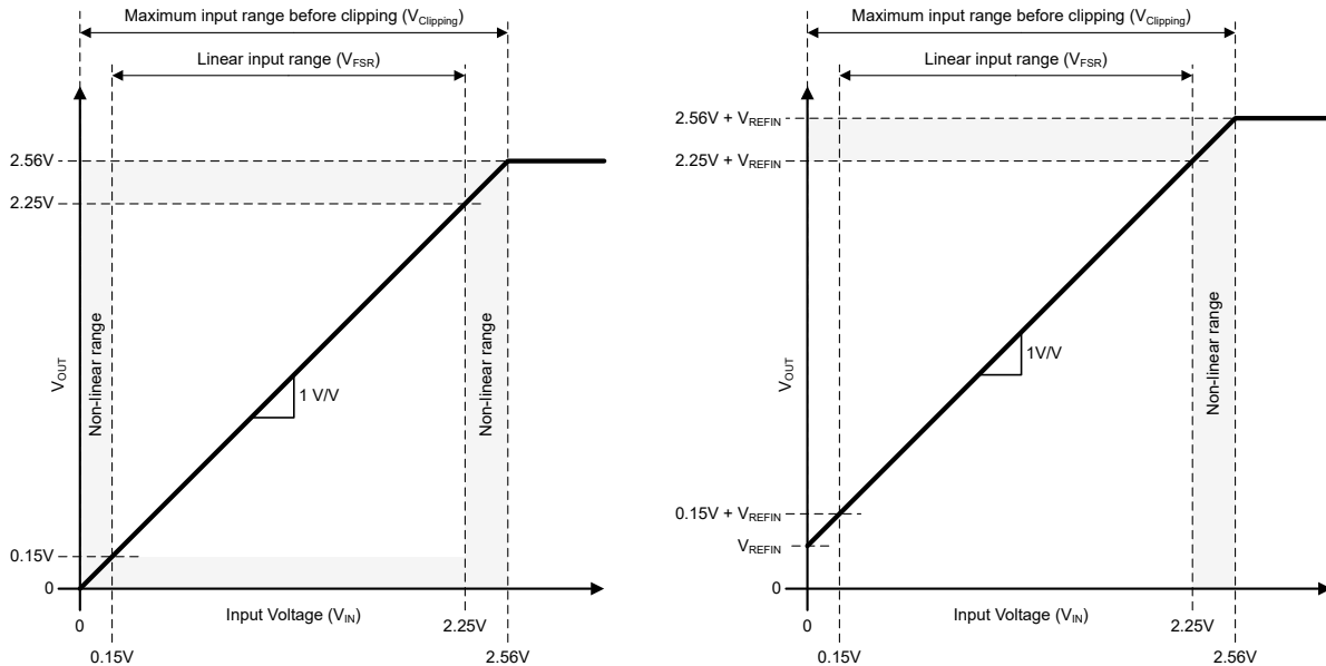
图 7-2. AMC0x11S-Q1 的输入到输出传送曲线 左：REFIN 短接至 GND2。右： V_{\text{REFIN}} = 150\text{mV}
