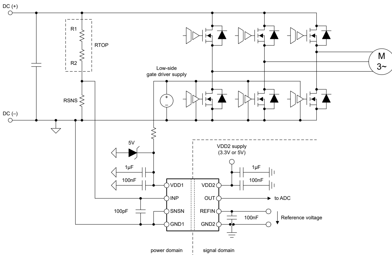
图 8-1. 在典型应用中使用 AMC0x11S-Q1
