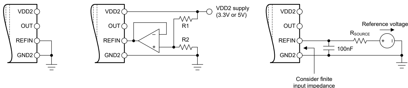
图 8-3. 连接 REFIN 引脚
