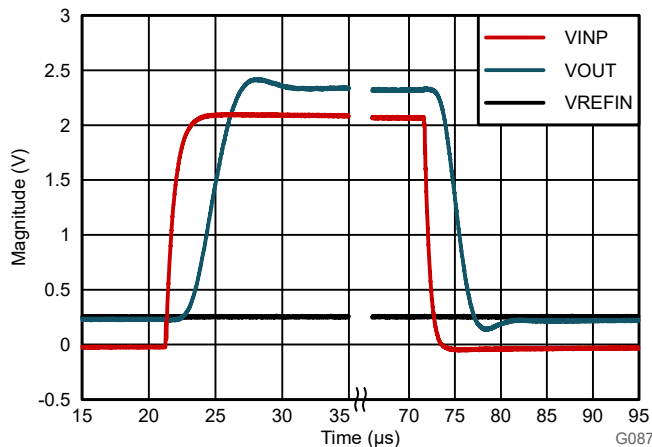
图 8-4. AMC0x11S-Q1 的阶跃响应
