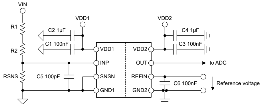
图 8-5. AMC0x11R 去耦
