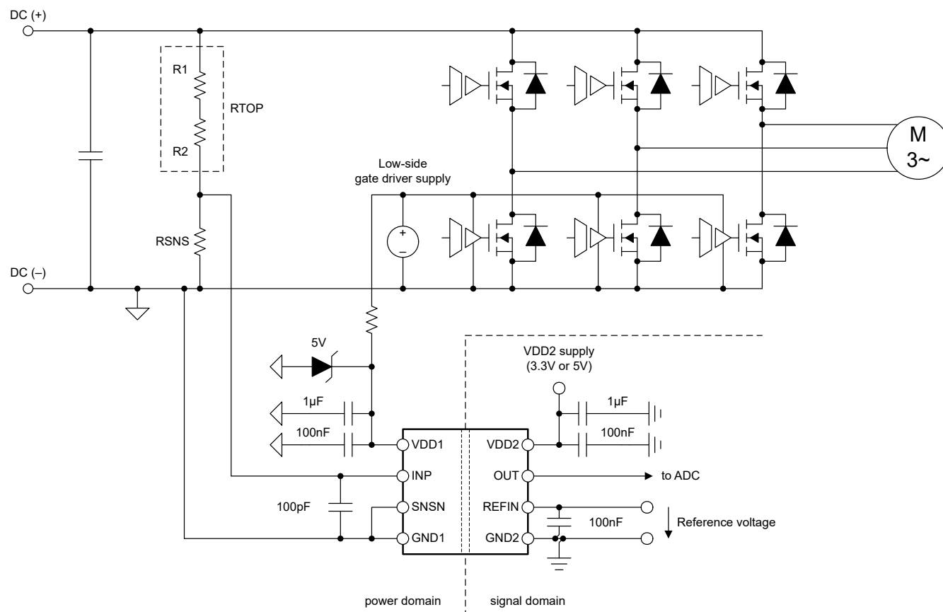
图 8-1. 在典型应用中使用 AMC0x11R
