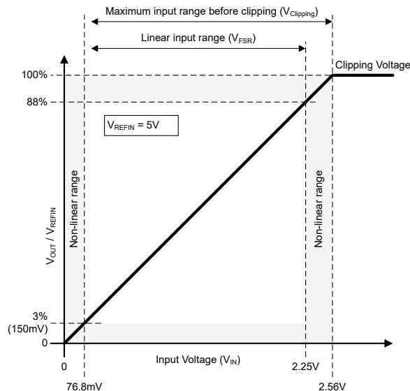
图 7-2. AMC0x11R 的输入到输出传送曲线
