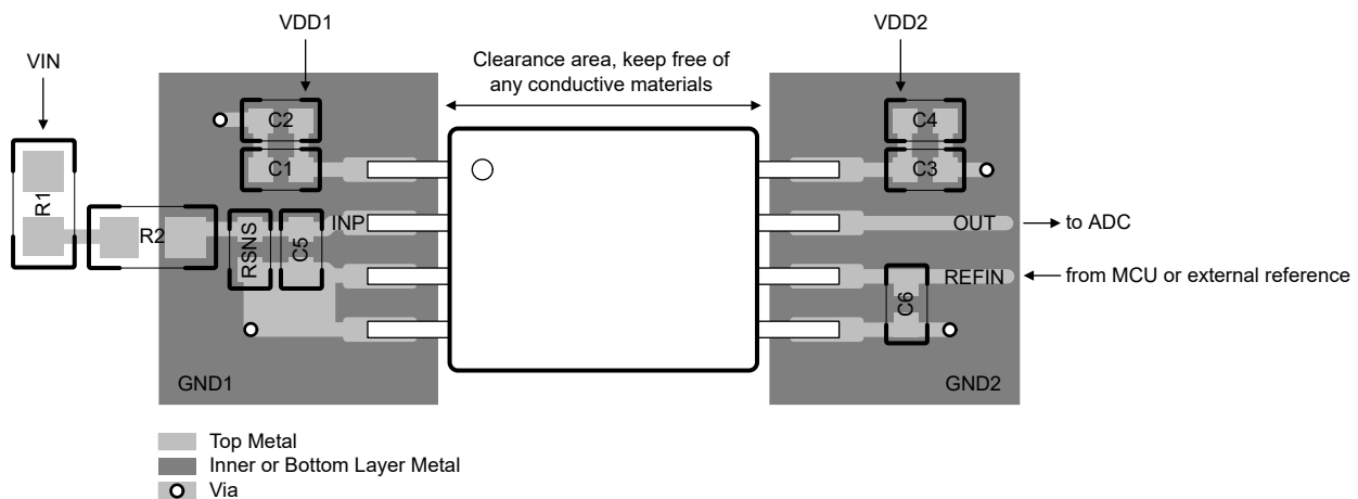
图 8-6. AMC0x11R 的建议布局
