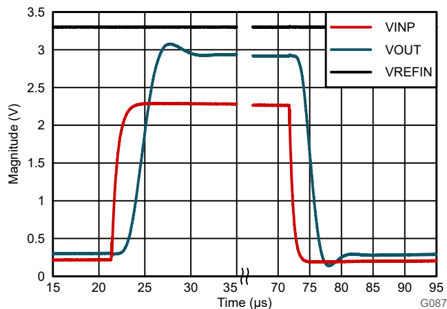
图 8-4. AMC0x11R 的阶跃响应
