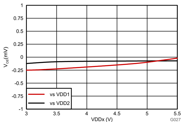
图 6-6. 输入失调电压与电源电压间的关系
