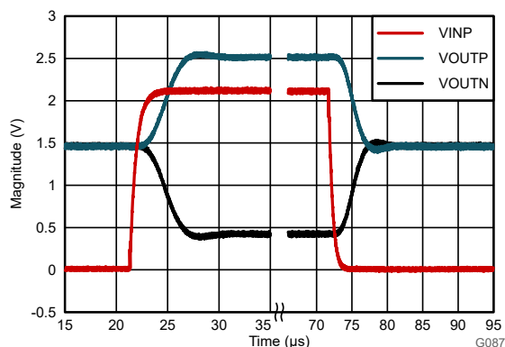
图 8-4. AMC0x11D 的阶跃响应
