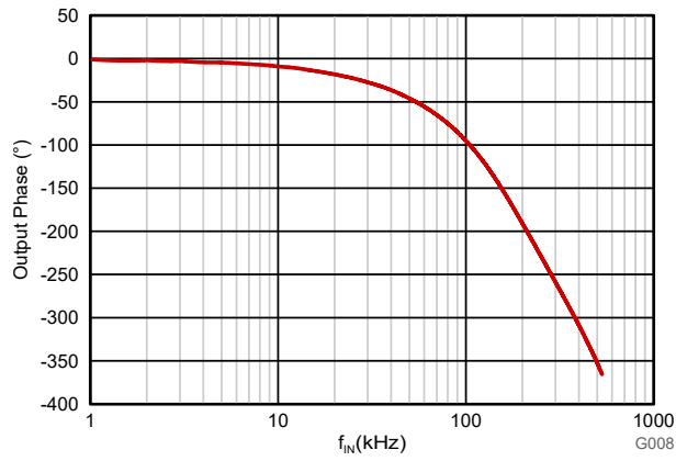
图 6-12. 输出相位与输入频率间的关系
