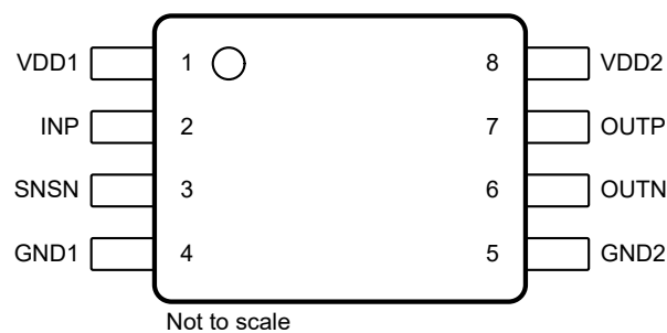
图 5-1. DWV 和 D 封装，8 引脚 SOIC (顶视图)
