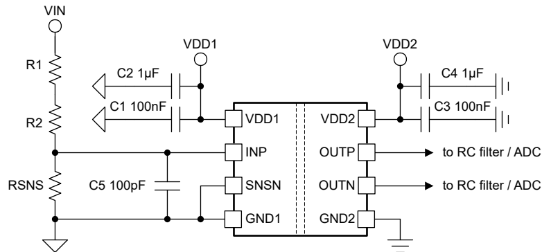
图 8-5. AMC0x11D 去耦
