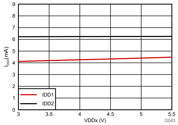
图 6-13. 电源电流与电源电压间的关系
