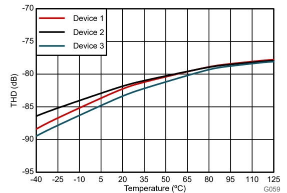
图 6-21. 非线性度与温度间的关系
