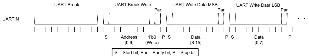
图 7-21. UARTIN Break Write Data Format
