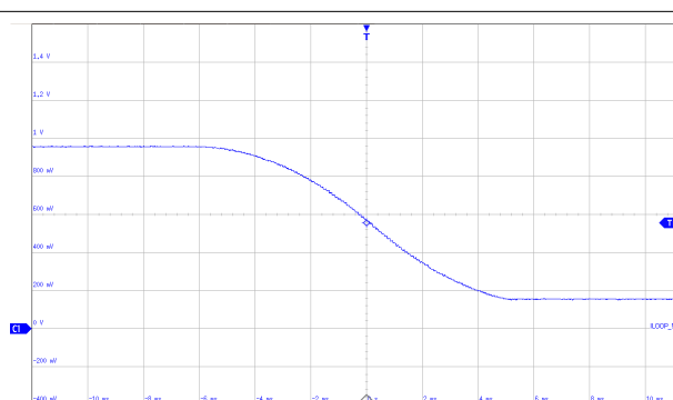
图 7-6. Sinusoidal Slew Rate: Falling
