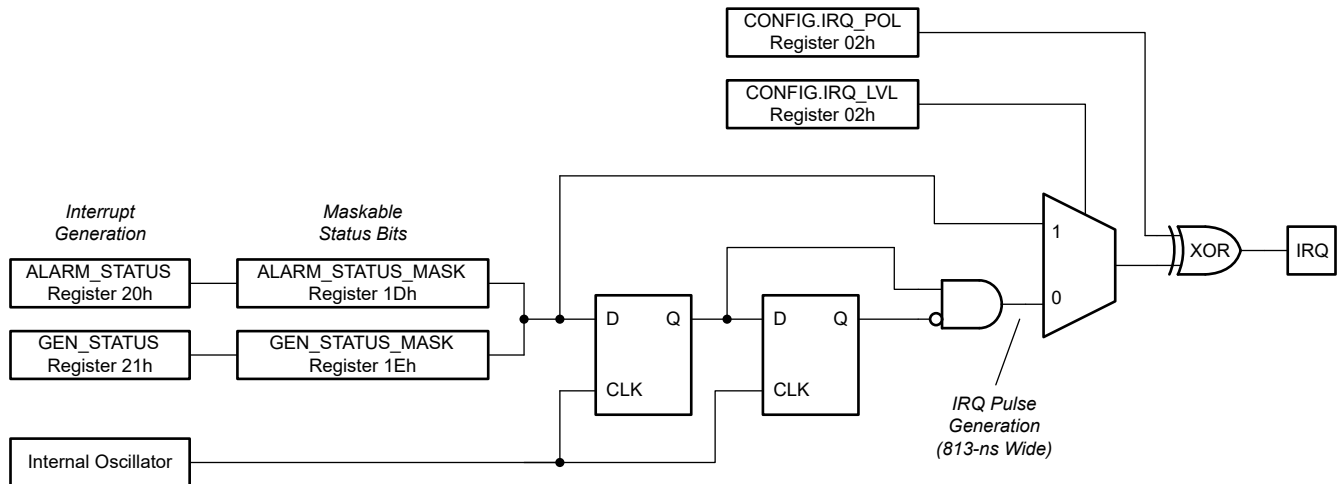
图 7-15. IRQ Block Diagram
