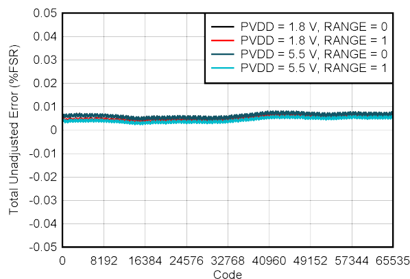
图 6-9. DAC TUE vs Digital Input Code
