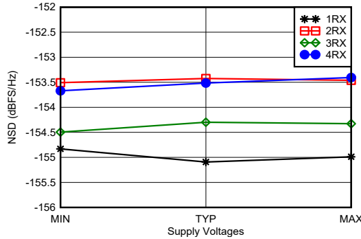
使用 3.6GHz 匹配时，单音幅度为 -20dBFS，偏移频率为 12.5MHz，所有电源均处于 MIN、TYP 或 MAX 推荐工作电压 图 7-385. 3.6GHz 条件下 RX 噪声频谱密度与电源电压和通道间的关系
