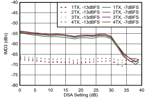
图 7-215. 8.11 GHz 条件下 TX IMD3 与 DSA 设置间的关系
