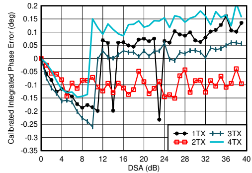
图 7-89. 2.6GHz 条件下 TX 校准差分相位误差与 DSA 设置和通道间的关系
