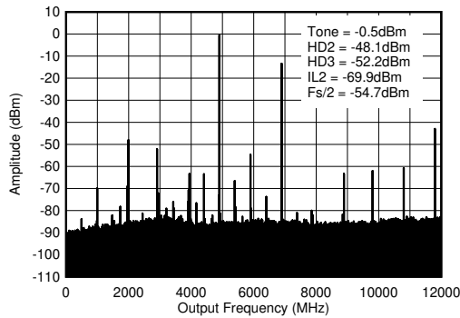
f_{\text{DAC}} = 11796.48\text{MSPS} , 交错模式, 4.9GHz 匹配, 包括 PCB 和电缆损耗。 \text{ILn} = f_s/n \pm f_{\text{OUT}} 。
