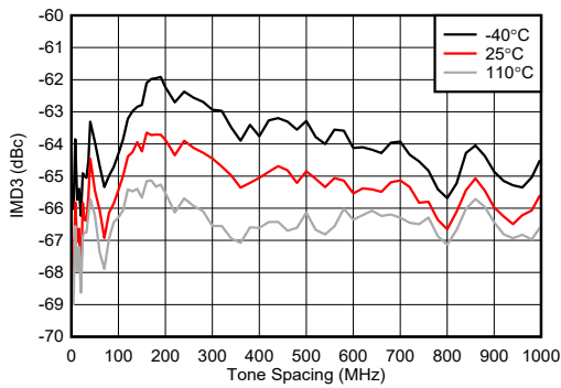
图 7-255. 9.61GHz 条件下 TX IMD3 与频率间隔间的关系
