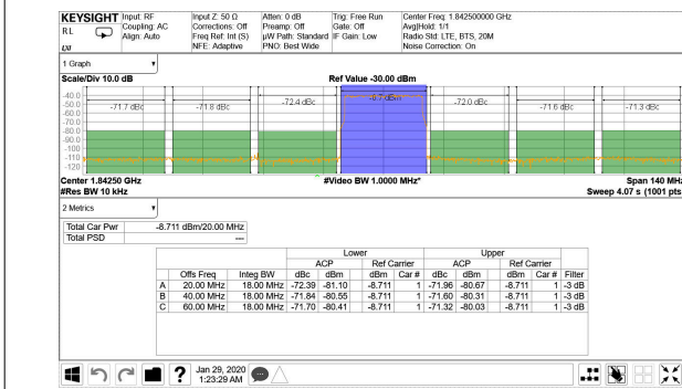
图 7-68. 1.8425GHz 条件下的 TX 20MHz LTE 输出频谱
