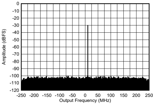
图 7-464. 9.61GHz 条件下 RX 单音输出 FFT
