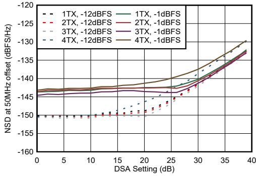
50MHz 偏移
