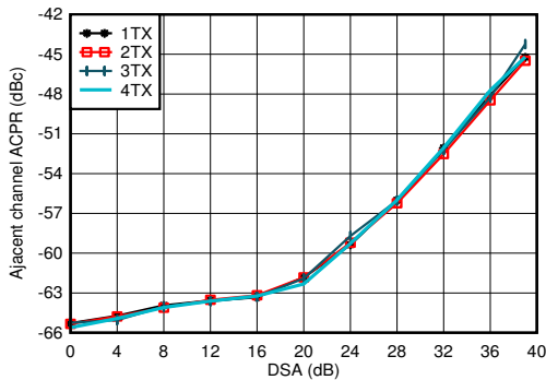
图 7-110. 2.6GHz 条件下 TX 100MHz NR ACPR 与 DSA 间的关系
