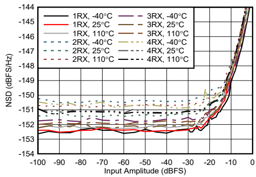
图 7-454. 9.6GHz 条件下 RX NSD 与数字振幅间的关系
