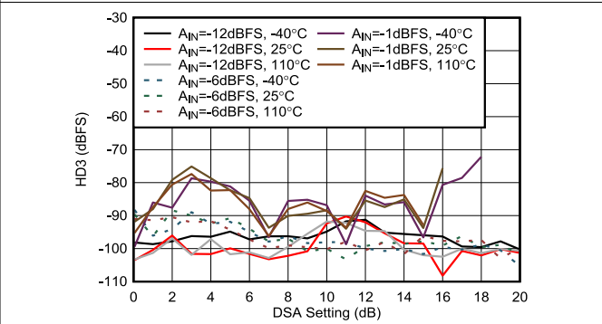
图 7-432. 8.1 GHz 条件下 RX HD3 与 DSA 设置间的关系
