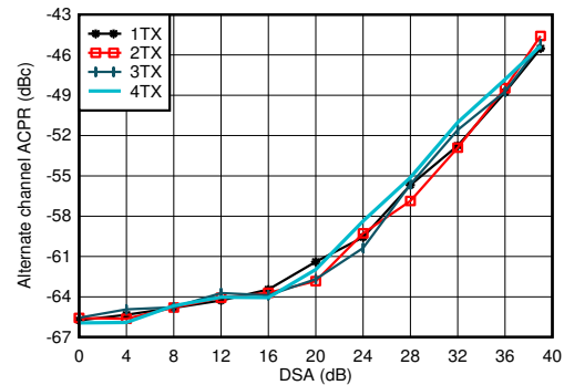
图 7-109. 2.6GHz 条件下 TX 20MHz LTE alt-ACPR 与 DSA 间的关系
