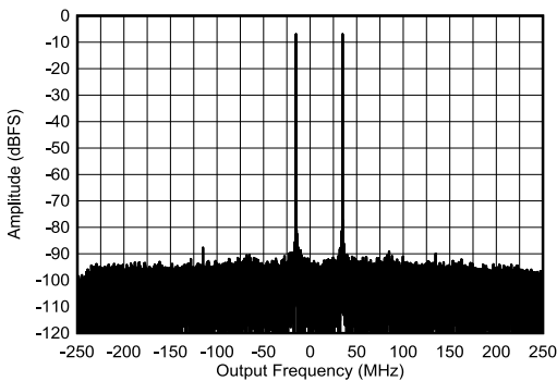
图 7-466. 9.61GHz 条件下 RX 单音输出 FFT
