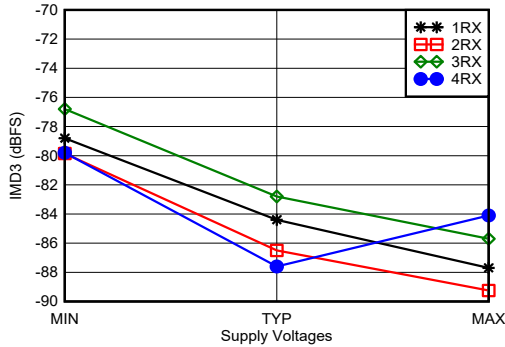
使用 3.6GHz 匹配时，单音幅度为 -7dBFS，频率间隔为 20MHz，所有电源均处于 MIN、TYP 或 MAX 推荐工作电压 图 7-383. 3.6GHz 条件下 RX IMD3 与电源电压和通道间的关系
