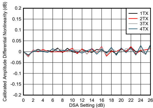
图 7-233. TX DSA 校准振幅微分非线性
