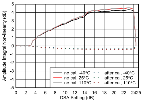
图 7-419. 8.11GHz 条件下 RX 振幅积分非线性
