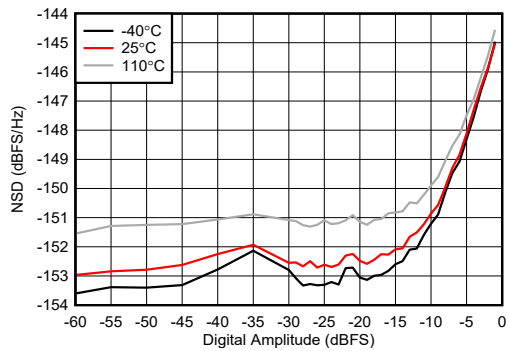
图 7-257. 9.61GHz 条件下 TX NSD 与数字振幅间的关系
