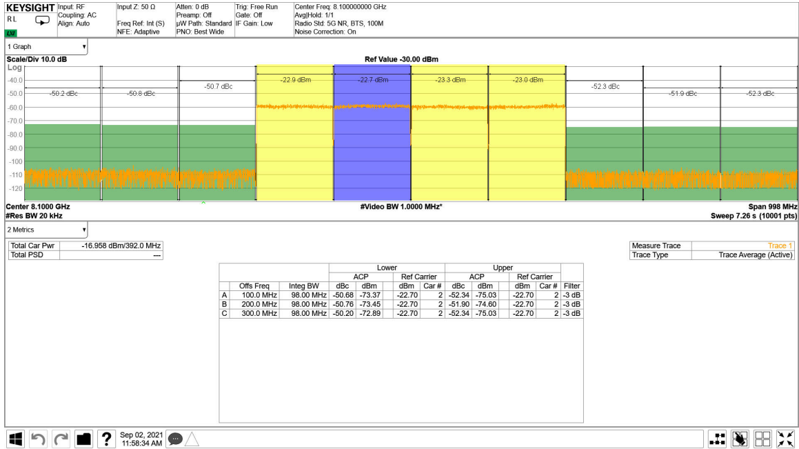
图 7-227. 8.1GHz 条件下 TX 4x100MHz NR 输出频谱
