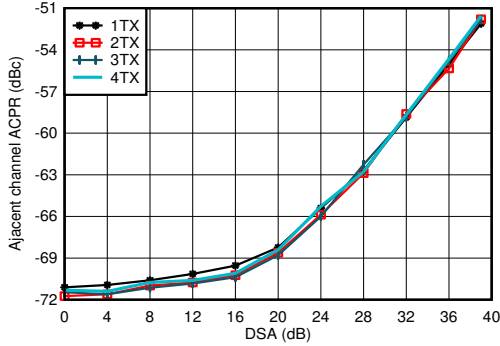
图 7-108. 2.6GHz 条件下 TX 20MHz LTE ACPR 与 DSA 间的关系
