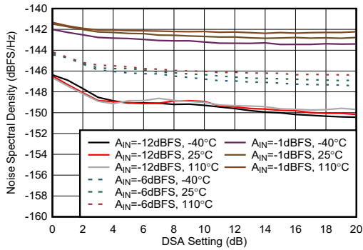
图 7-456. 9.6 GHz 条件下 RX NSD 与 DSA 设置间的关系
