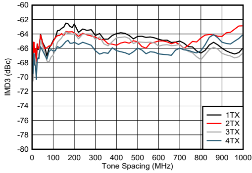
图 7-253. 9.61GHz 条件下 TX IMD3 与频率间隔间的关系
