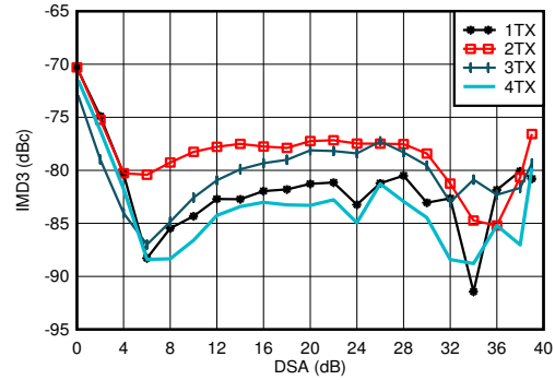
f_{\text{DAC}} = 11796.48\text{MSPS} , 交错模式, f_{\text{CENTER}} = 1.8\text{GHz} , 在 1.8 GHz 条件下匹配, 单音幅度为 -13\text{dBFS}
