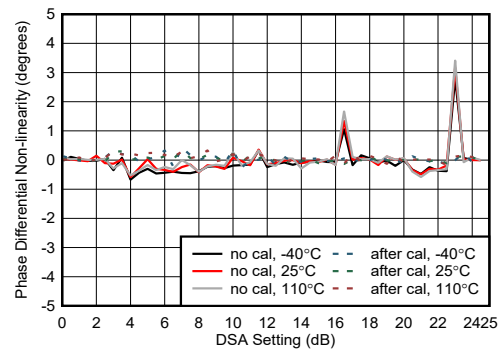
图 7-420. 8.11GHz 条件下 RX 相位微分非线性
