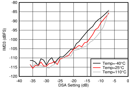
图 7-371. 3.6GHz 条件下 RX IMD3 与输入电平和温度间的关系
