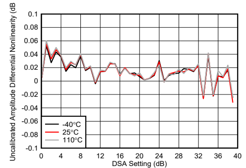
图 7-189. 8.11GHz 条件下 TX DSA 未校准振幅微分非线性
