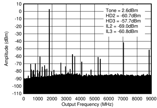
图 7-75. 1.8GHz (0 - f_{\text{DAC}} ) 条件下的 TX 单频 (-12dBFS) 输出频谱
