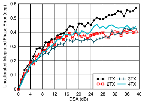
图 7-126. 3.5GHz 条件下 TX 未校准积分相位误差与 DSA 设置和通道间的关系
