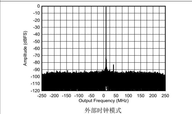
图 7-434. 8.1GHz 条件下 RX 单音输出 FFT, -1dBFS
