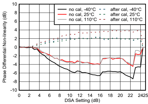
图 7-421. 8.11GHz 条件下 RX 相位微分非线性
