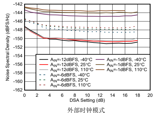
图 7-428. 8.11 GHz 条件下 RX NSD 与 DSA 设置间的关系
