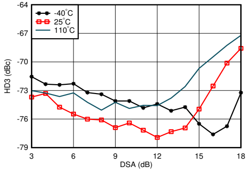
图 7-377. 3.6GHz 条件下 RX HD3 与 DSA 设置和温度间的关系
