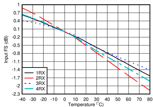
使用 4.9GHz 匹配时，为每个通道标准化为 25°C 时的满量程 图 7-387. 4.9GHz 条件下 RX 输入满量程与温度和通道间的关系
