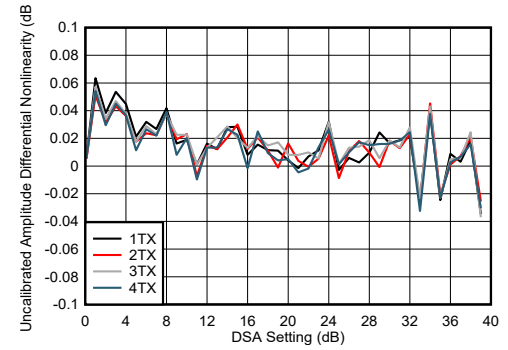
图 7-177. 8.11GHz 条件下 TX DSA 未校准振幅微分非线性
