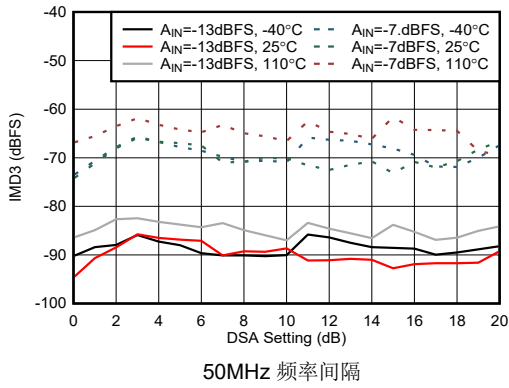
图 7-452. 9.6 GHz 条件下 RX IMD3 与 DSA 设置间的关系
