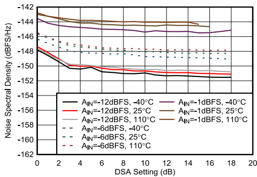
图 7-427. 8.11 GHz 条件下 RX NSD 与 DSA 设置间的关系
