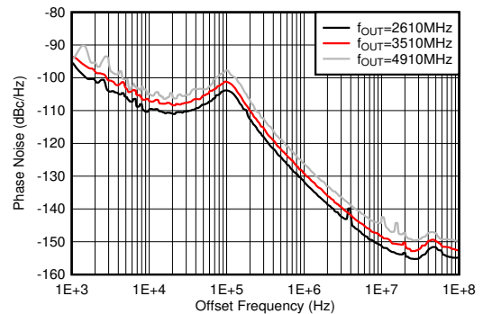
图 7-475. 25°C 条件下 12GHz VCO 相位噪声与偏移频率和 f_{\text{OUT}} 间的关系
