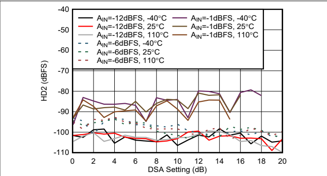
图 7-430. 8.1 GHz 条件下 RX HD2 与 DSA 设置间的关系
