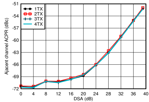
图 7-69. 1.8425GHz 条件下 TX 20MHz LTE ACPR 与数字电平间的关系
