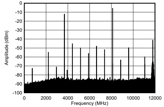
图 7-203. 8.1GHz 条件下 TX 单音输出频谱
