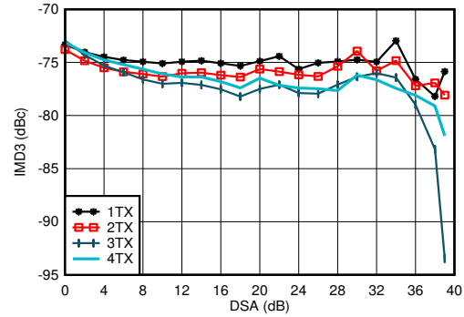
图 7-97. 2.6GHz 条件下 TX IMD3 与 DSA 设置间的关系
