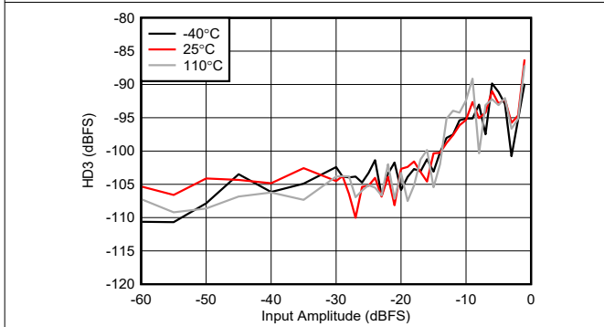
图 7-431. 8.1GHz 条件下 RX HD3 与数字振幅间的关系
