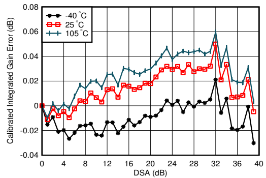
图 7-85. 2.6GHz 条件下 TX 校准差分增益误差与 DSA 设置和温度间的关系
