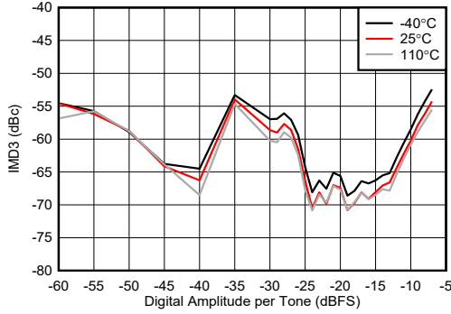
图 7-214. 8.11GHz 条件下 TX IMD3 与数字振幅间的关系
