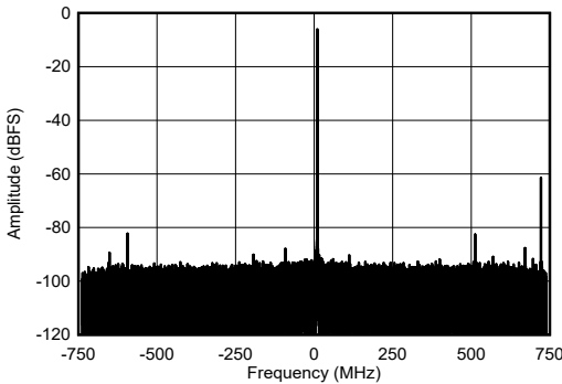
图 7-462. 9.61GHz 条件下 RX 单音输出 FFT
