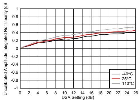
图 7-238. TX DSA 未校准振幅积分非线性
