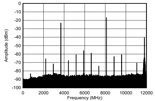
图 7-205. 8.1GHz 条件下 TX 单音输出频谱
