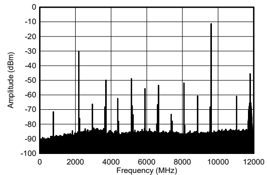
图 7-262. 9.61GHz 和 -1dBFS (宽带) 条件下 TX 单音频谱
