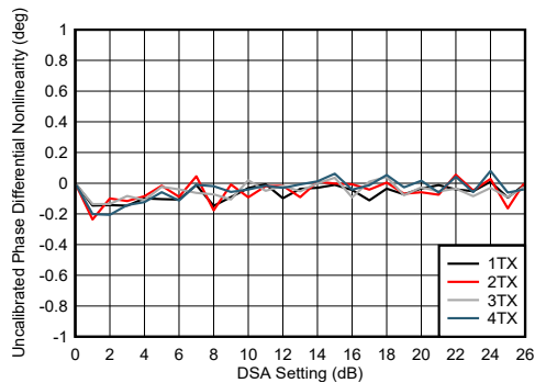
图 7-240. TX DSA 未校准相位微分非线性
