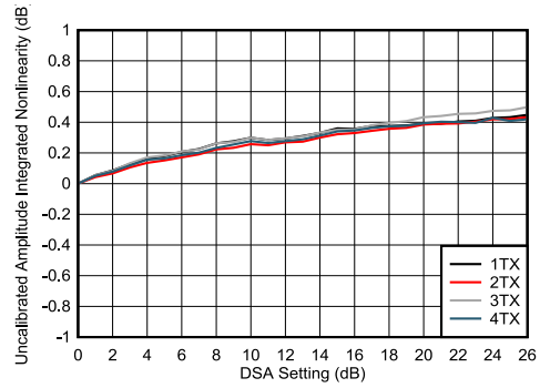
图 7-236. TX DSA 未校准振幅积分非线性
