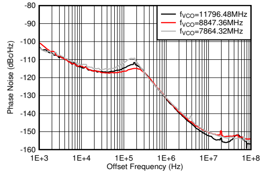
图 7-473. f_{\text{OUT}} = 2610\text{MHz} 时相位噪声与偏移频率和 f_{\text{VCO}} 间的关系
