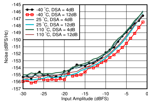
图 7-399. 4.9GHz 条件下 RX 噪声频谱密度与输入振幅和温度间的关系
