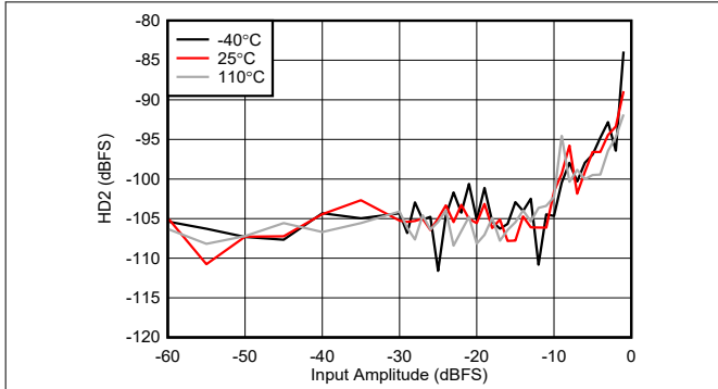
图 7-429. 8.1GHz 条件下 RX HD2 与数字振幅间的关系
