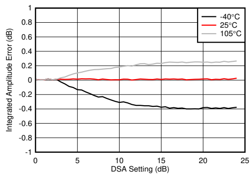
图 7-362. 3.6GHz 条件下 RX 校准差分振幅误差与 DSA 设置间的关系
