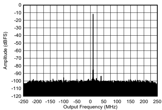
图 7-435. 8.1GHz 条件下 RX 单音输出 FFT, -3dBFS
