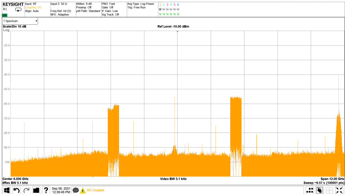
图 7-228. 8.1GHz 条件下 TX 4x100MHz NR 输出频谱
