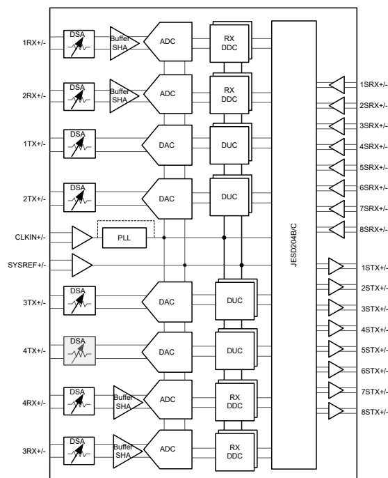
功能模块图
