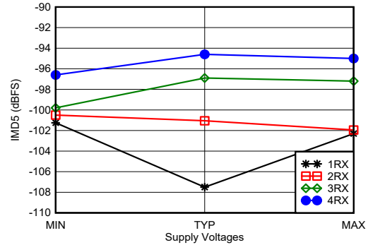
使用 3.6GHz 匹配时，单音幅度为 -7dBFS，频率间隔为 20MHz，所有电源均处于 MIN、TYP 或 MAX 推荐工作电压 图 7-384. 3.6GHz 条件下 RX IMD5 与电源电压和通道间的关系
