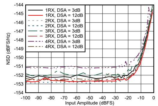
图 7-426. 8.11GHz 条件下 RX NSD 与数字振幅间的关系
