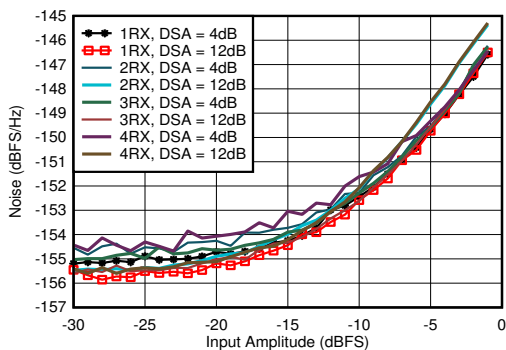
图 7-323. 1.75GHz 条件下 RX 噪声频谱密度与输入幅度和通道间的关系
