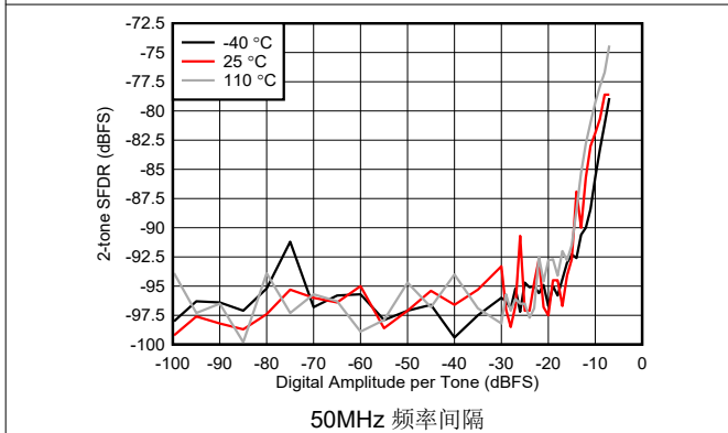
图 7-433. 8.1GHz 条件下 RX 双音 SFDR 与数字振幅间的关系
