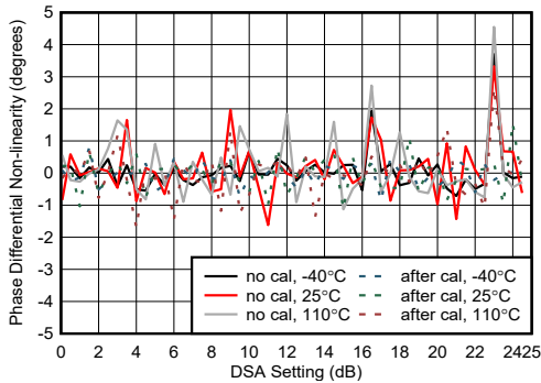
图 7-448. 9.6GHz 条件下 RX 相位微分非线性
