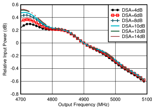
通过匹配，为每个 DSA 设置标准化为 4.9 GHz 下的功率 图 7-386. RX 带内增益平坦度， f_{\text{IN}} = 4900\text{MHz}
