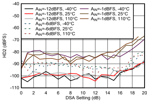
图 4-463. 9.6GHz 条件下 RX HD2 与 DSA 设置间的关系
