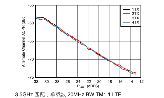
图 4-143. 3.5GHz 条件下 TX 20MHz LTE alt-ACPR 与数字电平间的关系
