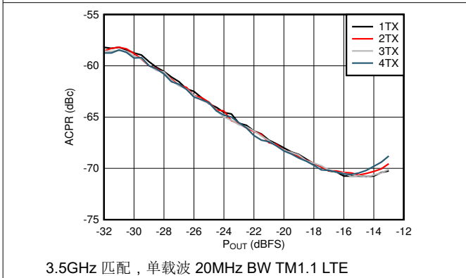
图 4-142. 3.5GHz 条件下 TX 20MHz LTE ACPR 与数字电平间的关系
