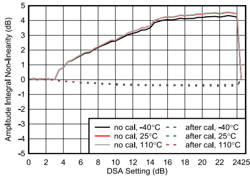
图 4-426. 8.11GHz 条件下 RX 振幅积分非线性
