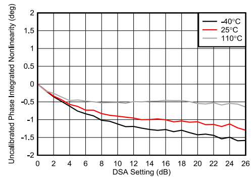
图 4-250. TX DSA 未校准相位积分非线性
