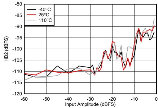
图 4-462. 9.6GHz 条件下 RX HD2 与数字电平间的关系
