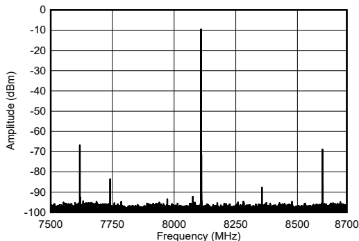
图 4-204. 8.11GHz 条件下 TX 单音输出频谱
