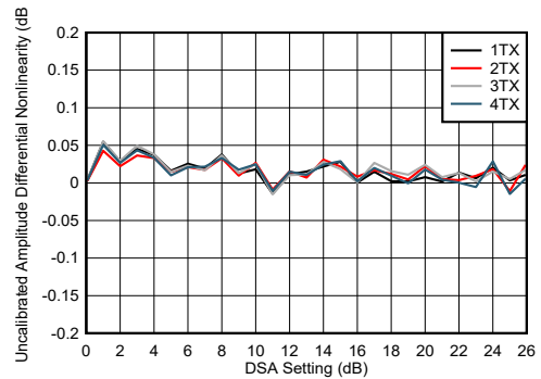
图 4-236. TX DSA 未校准振幅微分非线性
