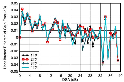
f_{\text{DAC}} = 11796.48\text{MSPS} , 交错模式, 在 4.9GHz 下匹配 差分增益误差 = P_{\text{OUT}}(\text{DSA 设置} - 1) - P_{\text{OUT}}(\text{DSA 设置}) + 1
