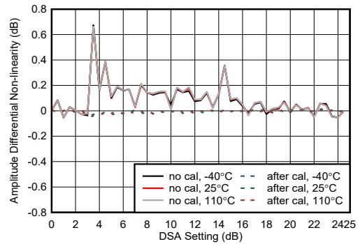
图 4-425. 8.11GHz 条件下 RX 振幅微分非线性
