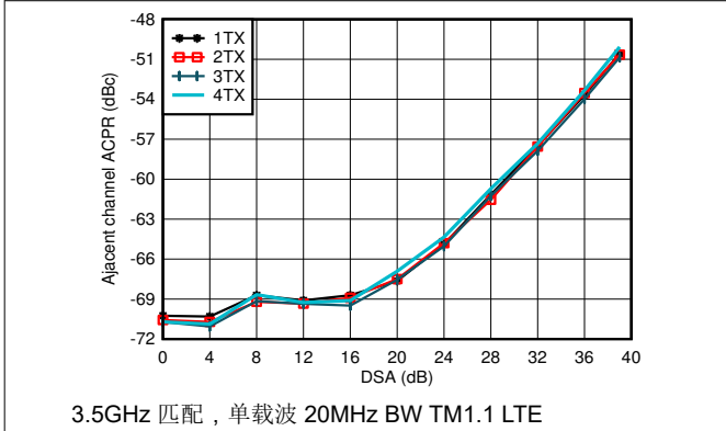
图 4-140. 3.5GHz 条件下的 TX 20MHz LTE ACPR 与 DSA 设置间的关系
