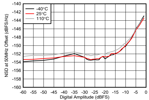
50MHz 偏移下
