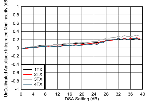
图 4-191. 8.11GHz 条件下 TX DSA 未校准振幅积分非线性
