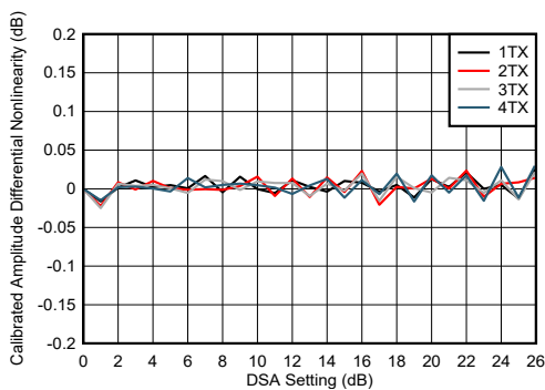
图 4-237. TX DSA 已校准振幅微分非线性
