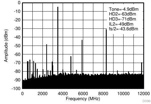
图 4-147. 3.5GHz (0- f_{\text{DAC}} ) 条件下的 TX 单频 (-6dBFS) 输出频谱
