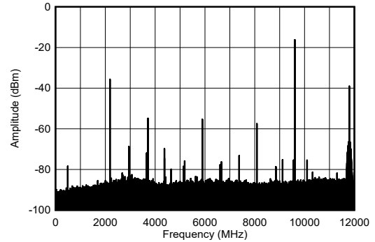
图 4-270. 9.61GHz 和 -12dBFS (宽带) 条件下的 TX 单音频谱
