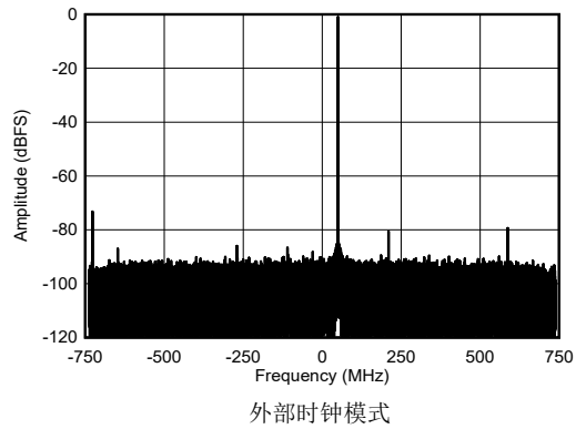
图 4-441. 8.11GHz 条件下 RX 单频输出 FFT, -1dBFS
