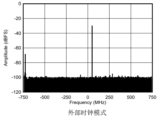
图 4-443. 8.11GHz 条件下 RX 单频输出 FFT, -30dBFS
