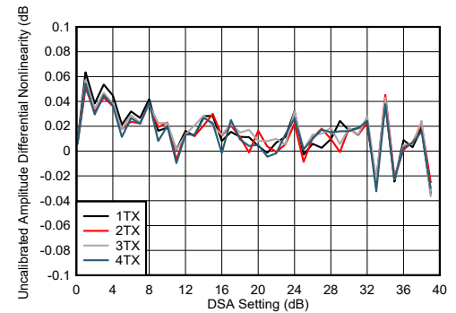
图 4-187. 8.11GHz 条件下 TX DSA 未校准振幅微分非线性
