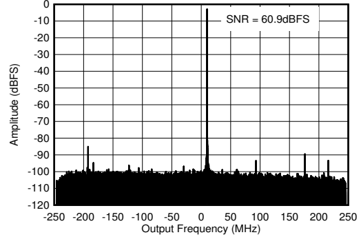
图 4-327. 1.75GHz 条件下的 RX 输出 FFT
