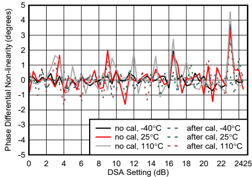
图 4-453. 9.6GHz 条件下 RX 相位微分非线性
