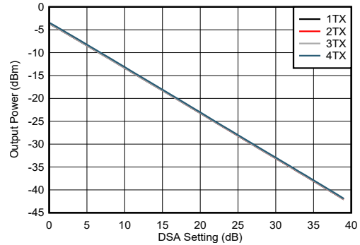
图 4-185. 8.11GHz 条件下 TX 输出功率与 DSA 设置间的关系
