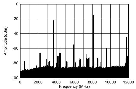
图 4-209. 8.11GHz 条件下 TX 双音输出频谱
