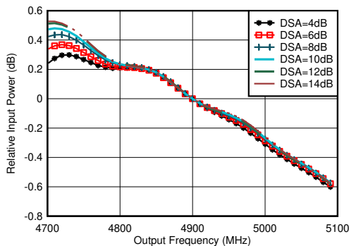
图 4-393. RX 带内增益平坦度， f_{IN} = 4900\text{MHz}
