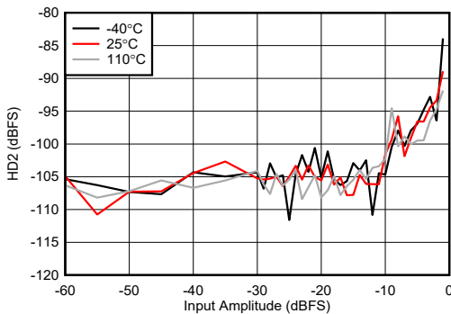
图 4-436. 8.11GHz 条件下 RX HD2 与数字振幅间的关系
