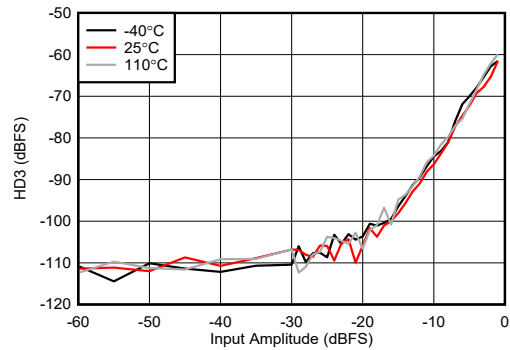
图 4-464. 9.6GHz 条件下 RX HD3 与数字电平间的关系
