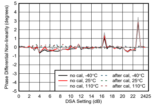
图 4-427. 8.11GHz 条件下 RX 相位微分非线性
