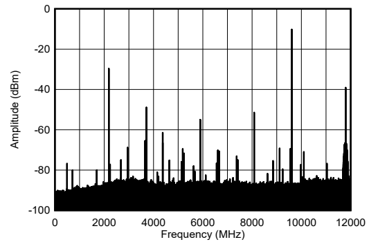
图 4-266. 9.61GHz 和 -1dBFS (宽带) 条件下的 TX 单音频谱
