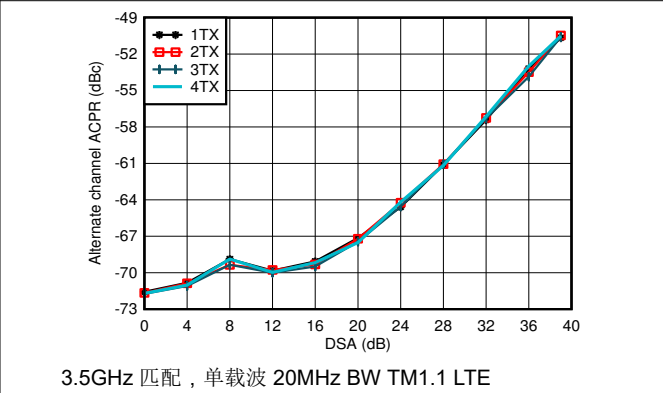
图 4-141. 3.5GHz 条件下的 TX 20MHz LTE alt-ACPR 与 DSA 设置间的关系
