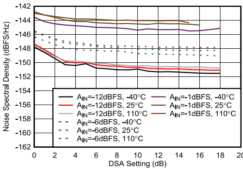
图 4-434. 8.11 GHz 条件下 RX NSD 与 DSA 设置间的关系
