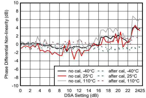
图 4-454. 9.6GHz 条件下 RX 相位积分非线性
