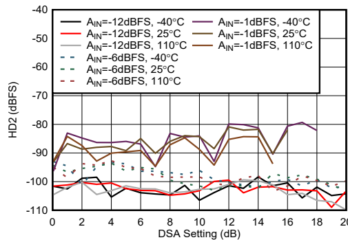
图 4-437. 8.11GHz 条件下 RX HD2 与 DSA 设置间的关系
