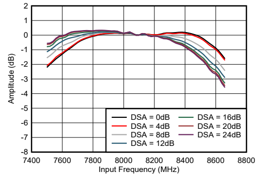
图 4-423. RX 振幅与频率和 DSA 设置间的关系
