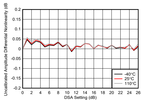
图 4-238. TX DSA 未校准振幅微分非线性
