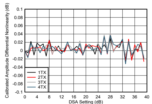
图 4-188. 8.11GHz 条件下 TX DSA 已校准振幅微分非线性
