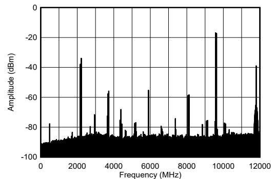
图 4-274. 9.61GHz 和 -13dBFS (宽带) 条件下的 TX 双音频谱
