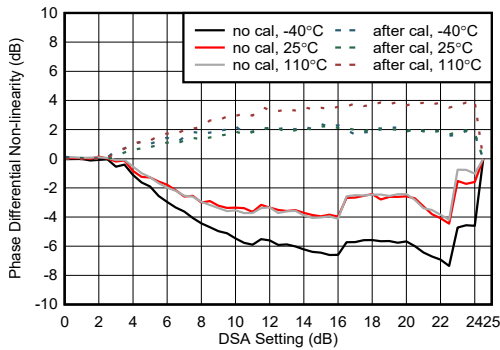
图 4-428. 8.11GHz 条件下 RX 相位微分非线性
