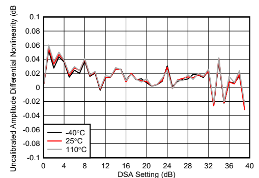
图 4-189. 8.11GHz 条件下 TX DSA 未校准振幅微分非线性
