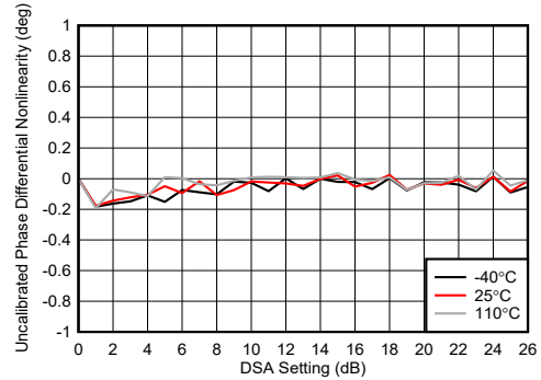
图 4-246. TX DSA 未校准相位微分非线性
