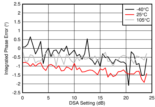
图 4-373. 3.6GHz 条件下 RX 校准差分相位误差与 DSA 设置间的关系
