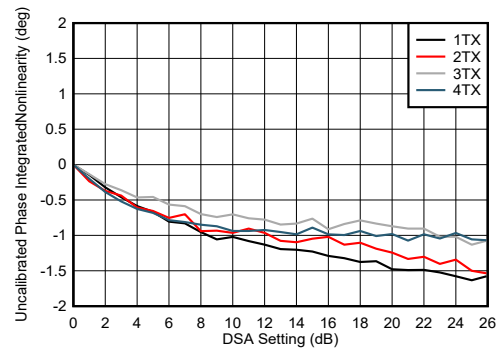
图 4-248. TX DSA 未校准相位积分非线性
