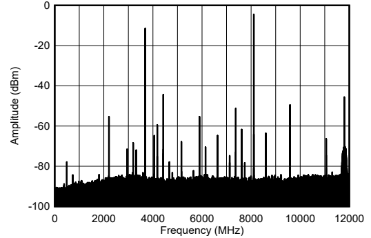
图 4-203. 8.11GHz 条件下 TX 单音输出频谱
