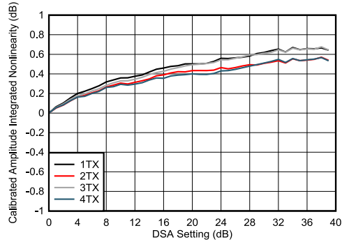
图 4-192. 8.11GHz 条件下 TX DSA 已校准振幅积分非线性
