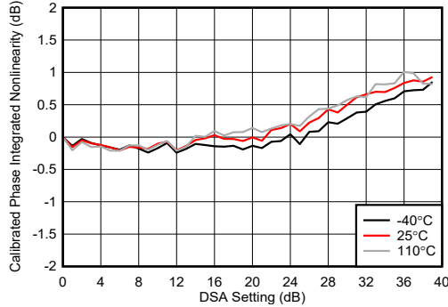
图 4-202. 8.11GHz 条件下 TX DSA 已校准相位积分非线性
