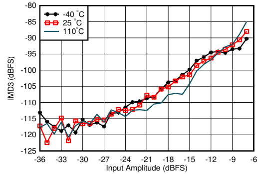
使用 1.8GHz 匹配时，频率间隔 = 20MHz，DSA = 12dB
