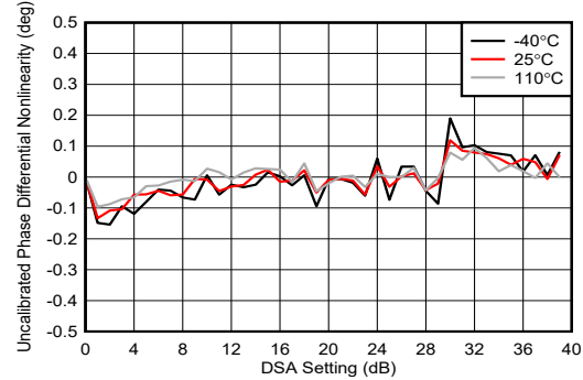
图 4-197. 8.11GHz 条件下 TX DSA 未校准相位微分非线性
