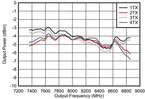
图 4-184. 8.11GHz 条件下 TX 输出功率与频率间的关系
