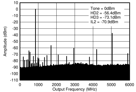
f_{\text{DAC}} = 5898.2\text{MSPS} , 交错模式, 0.8GHz 匹配, 包括 PCB 和电缆损耗 \text{IL}_n = f_s/n \pm f_{\text{OUT}}
