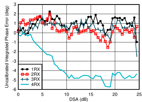
图 4-400. 4.9GHz 条件下 RX 未校准差分相位误差与 DSA 设置间的关系
