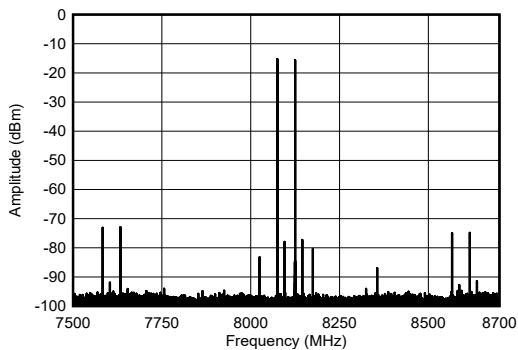
图 4-210. 8.11GHz 条件下 TX 双音输出频谱
