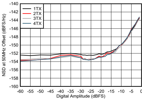
50MHz 偏移下
