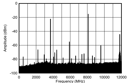
图 4-205. 8.11GHz 条件下 TX 单音输出频谱
