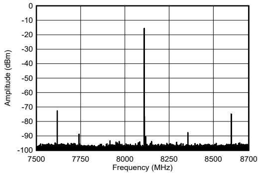
图 4-208. 8.11GHz 条件下 TX 单音输出频谱
