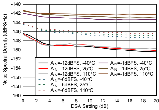
图 4-461. 9.6 GHz 条件下 RX NSD 与 DSA 设置间的关系
