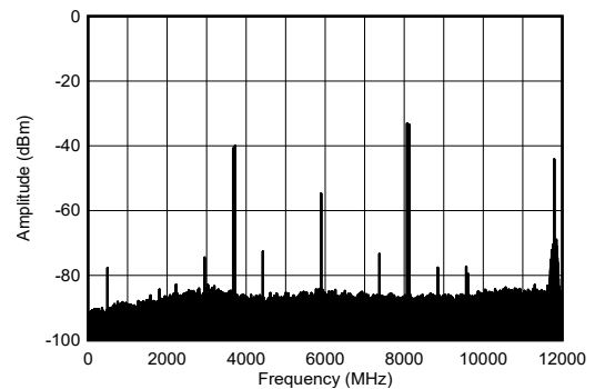
图 4-211. 8.11GHz 条件下 TX 双音输出频谱
