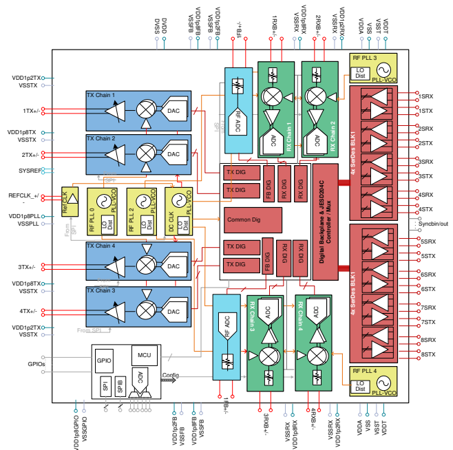
AFE7700 方框图
