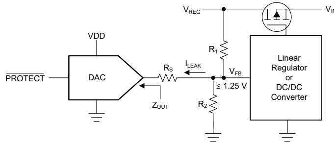
图 6-13. 高阻抗（高阻态）输出和 \overline{\text{PROTECT}} 输入
