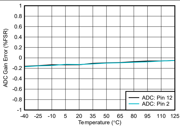
图 5-57. ADC 增益误差与温度间的关系
