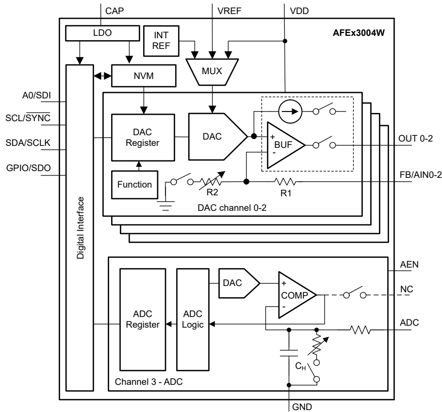
图 6-3. 启用的 ADC 器件功能图
