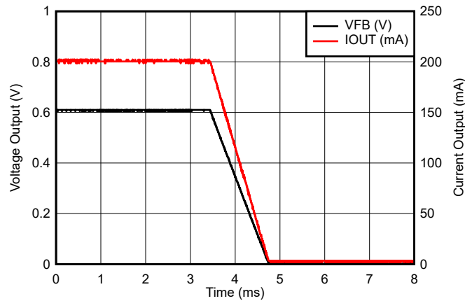
图 8-2. IOUT 和 VFB 导通至关断转换
