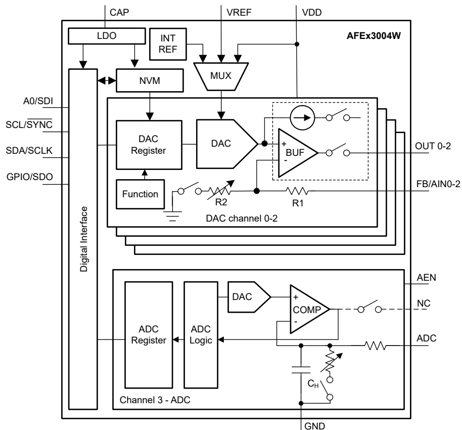
图 6-2. 启用的 ADC 器件功能图
