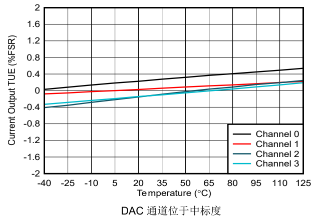
图 5-38. 电流输出 TUE 与温度间的关系
