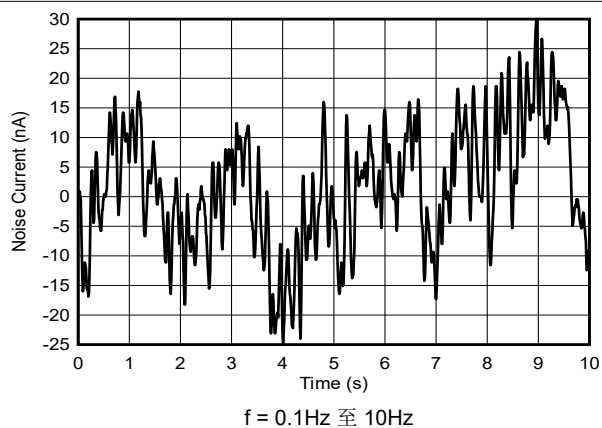
图 5-50. 电流输出闪烁噪声
