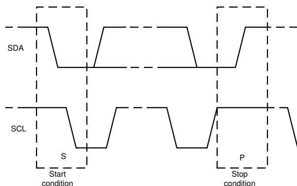
图 6-24. 启动和停止条件
