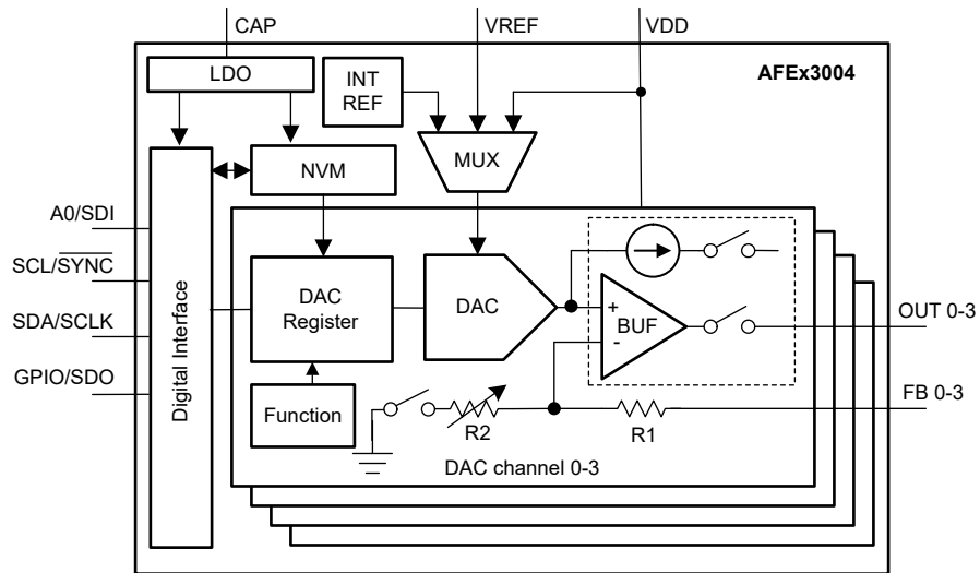
图 6-1. 已禁用 ADC 器件功能图
