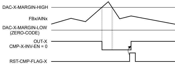
图 6-9. 具有低电平有效输出的闭锁比较器
