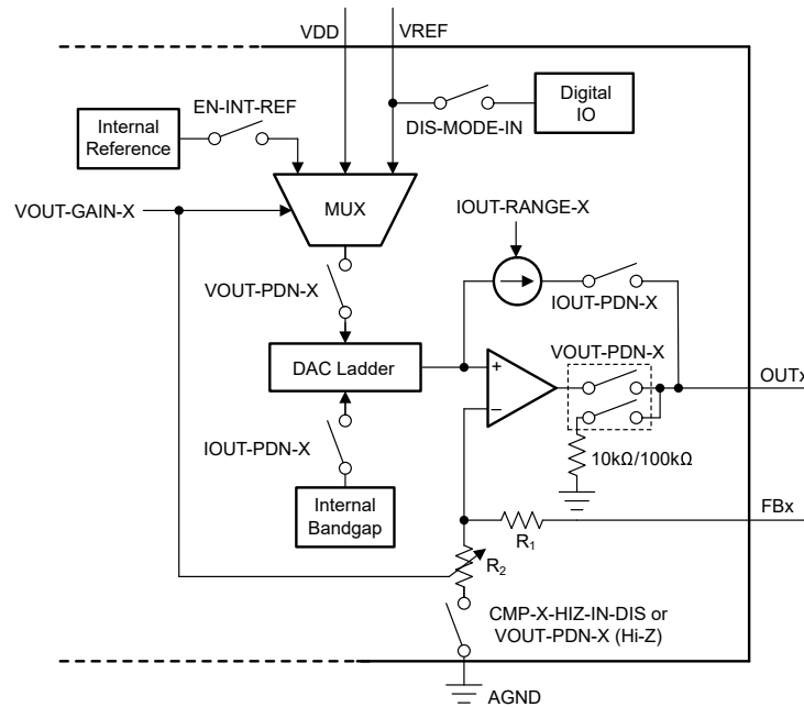
图 6-4. 电压基准选择与断电逻辑
