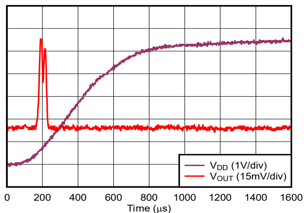
图 5-23. 电压输出上电干扰
