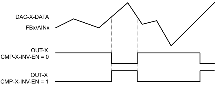
图 6-7. 可编程比较器操作
