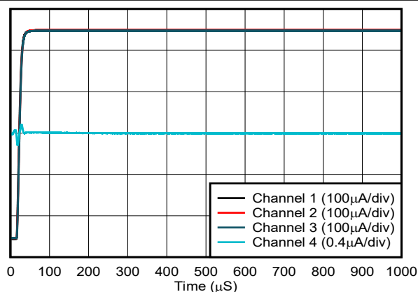
图 5-45. 电流输出上电干扰
