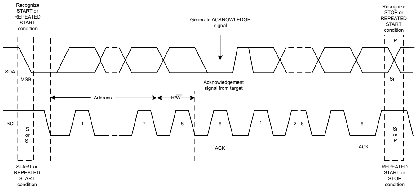
图 6-26. I 2 C 总线协议
