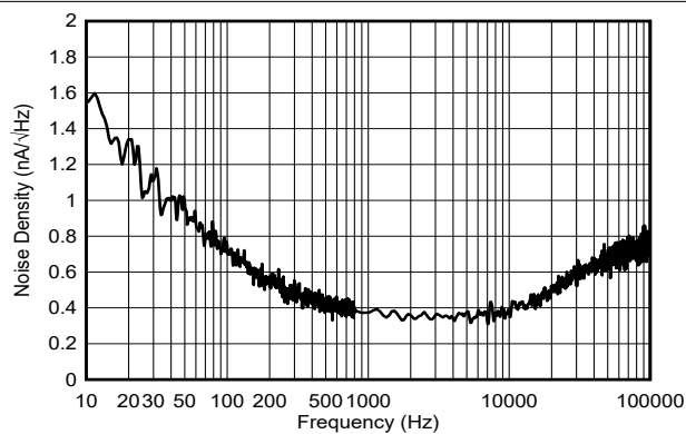
图 5-49. 电流输出噪声密度
