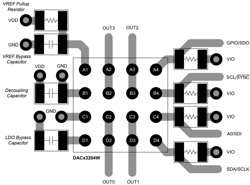
图 8-3. 布局示例
