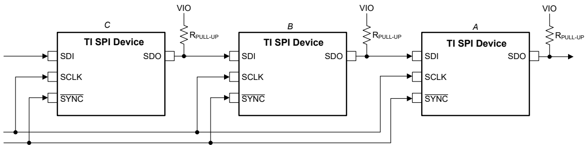
图 6-21. SPI 菊花链连接
