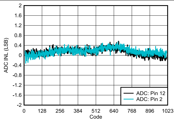
图 5-51. ADC INL 与数字输出代码间的关系
