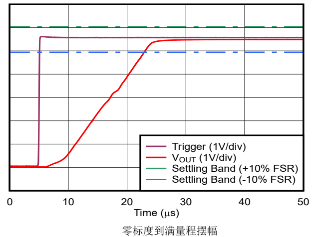
图 5-21. 电压输出稳定时间：上升沿
