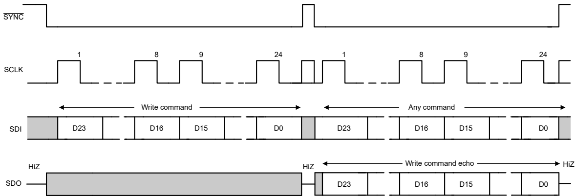
图 6-19. SPI 写入周期
