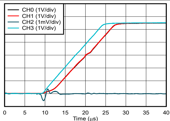
图 5-23. 电压输出上电干扰
