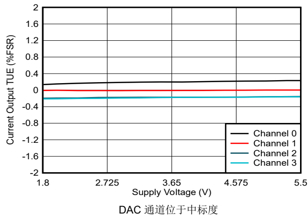
图 5-39. 电流输出 TUE 与电源电压间的关系
