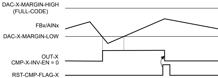
图 6-10. 具有高电平有效输出的锁存比较器
