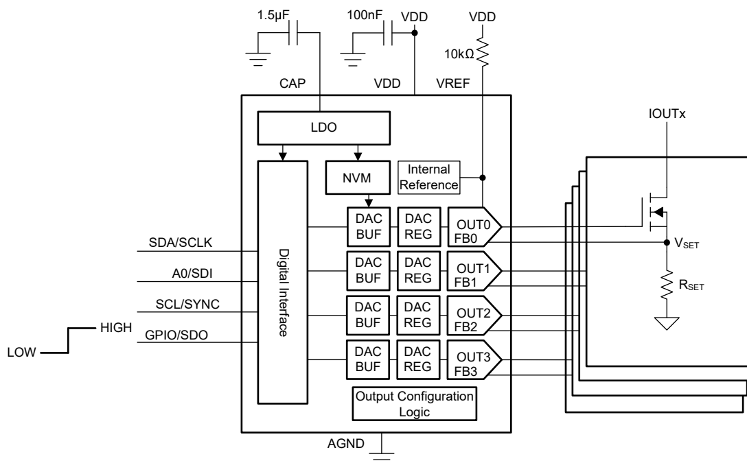
图 8-1. 电流源
