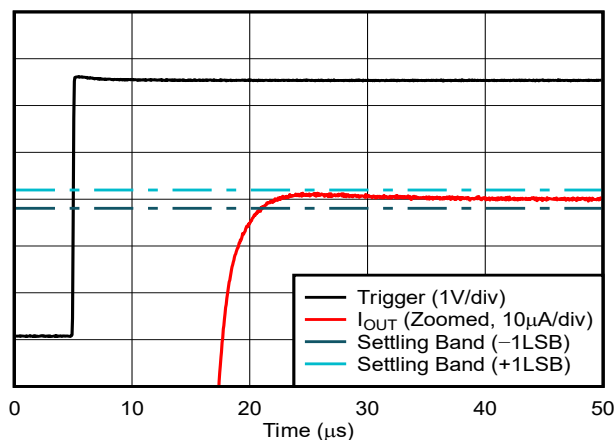
图 5-43. 输出电流稳定时间：上升沿（ \frac{1}{4} 至 \frac{3}{4} 标度）
