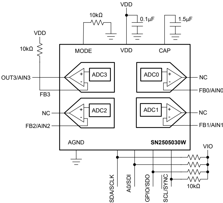
图 6-5. ADC 接口
