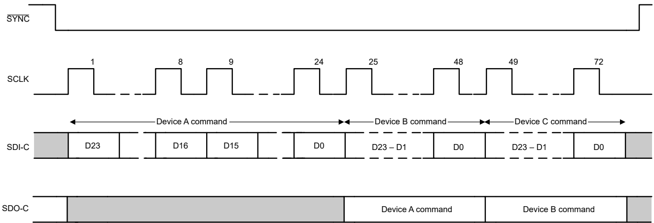
图 6-22. SPI 菊花链写入周期
