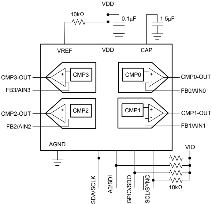
图 6-6. 比较器接口
