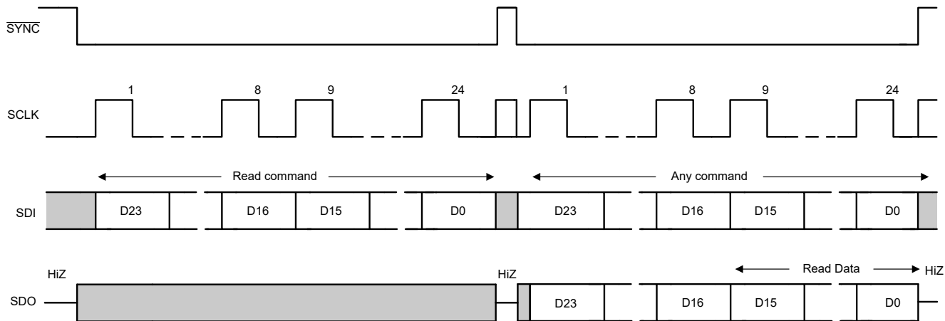
图 6-20. SPI 读取周期
