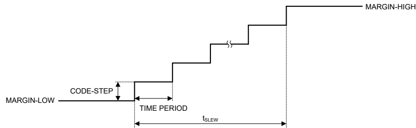
图 6-12. 可编程压摆率控制
