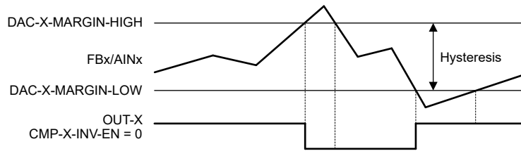
图 6-8. 不带锁存输出的可编程迟滞
