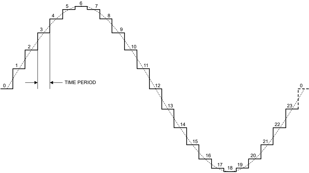
图 6-17. 正弦波生成
