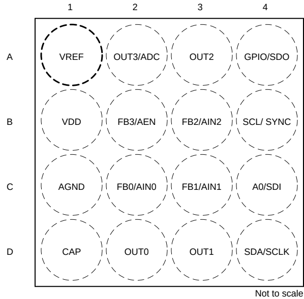
图 4-1. YBH 封装，16 引脚 DSBGA ( 俯视图 )
