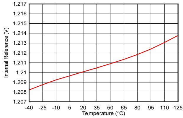
图 5-61. 内部基准与温度间的关系
