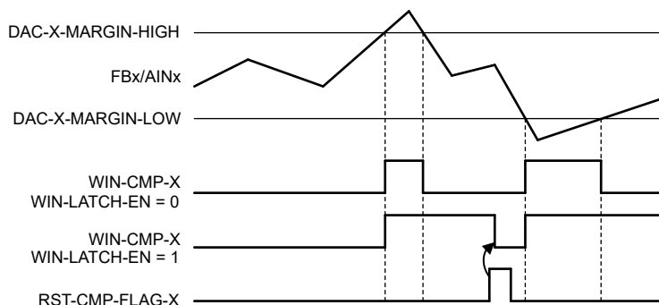
图 6-11. 窗口比较器操作
