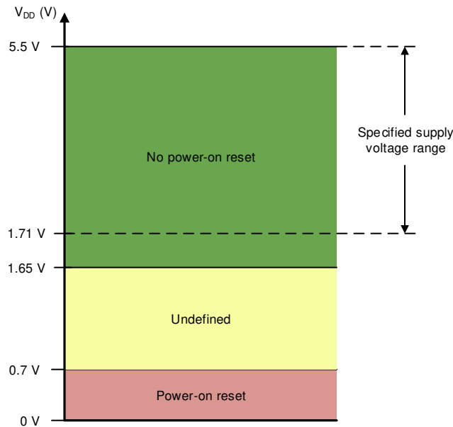
图 6-18. V_{DD} POR 电路的阈值电平
