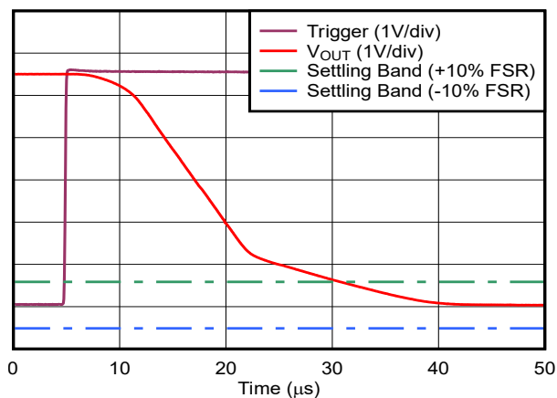
图 5-22. 电压输出稳定时间：下降沿
