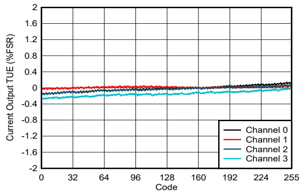
图 5-37. 电流输出 TUE 与数字输入代码间的关系
