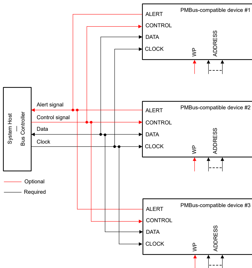
图 6-14. PMBus 连接
