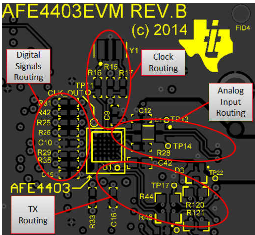
图 11-1. Example Layout
