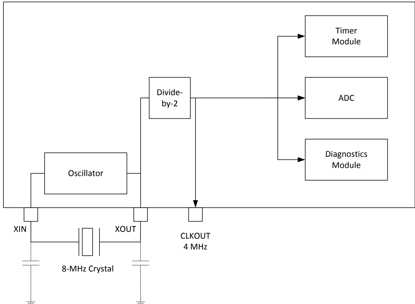
图 8-7. AFE Clocking
