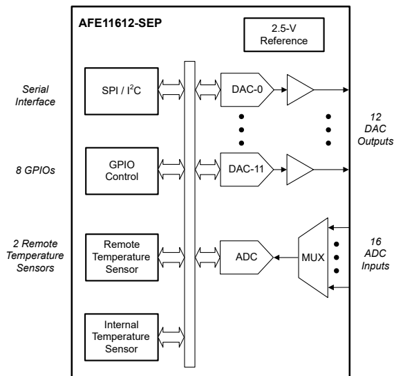
简化原理图
