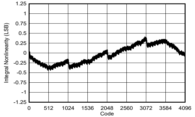
图 6-7. Integral Linearity Error vs Code
