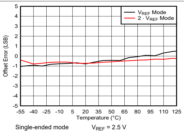
图 6-37. Offset vs Temperature
