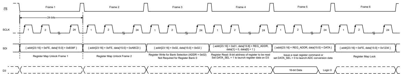
图 7-18. 寄存器读取
