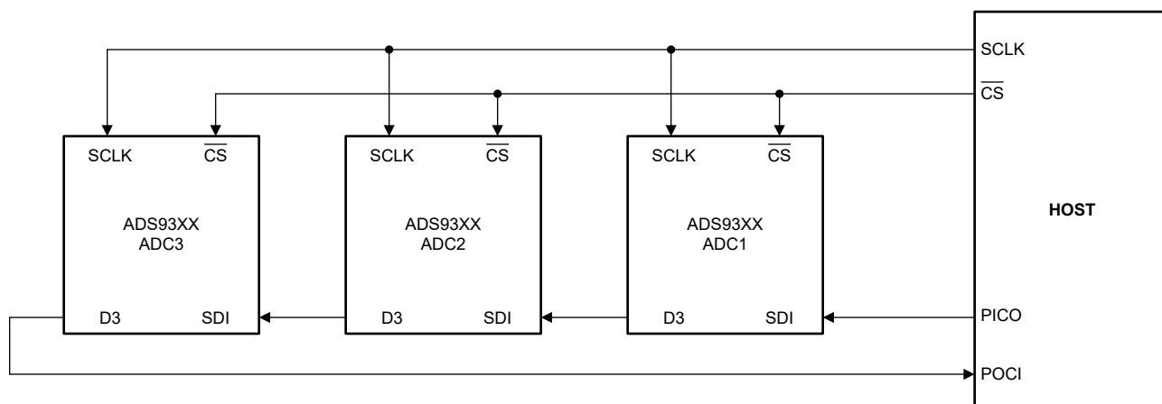
图 7-14. 菊花链连接
