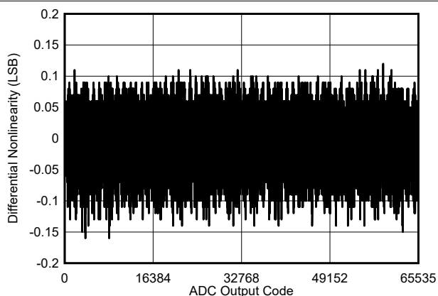
图 6-6. 典型 DNL
