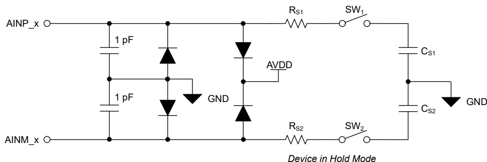
图 7-1. 模拟输入
