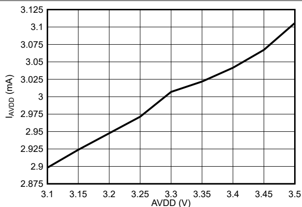
图 6-29. 2.5V 基准下 AVDD 电流与 AVDD 电压间的关系
