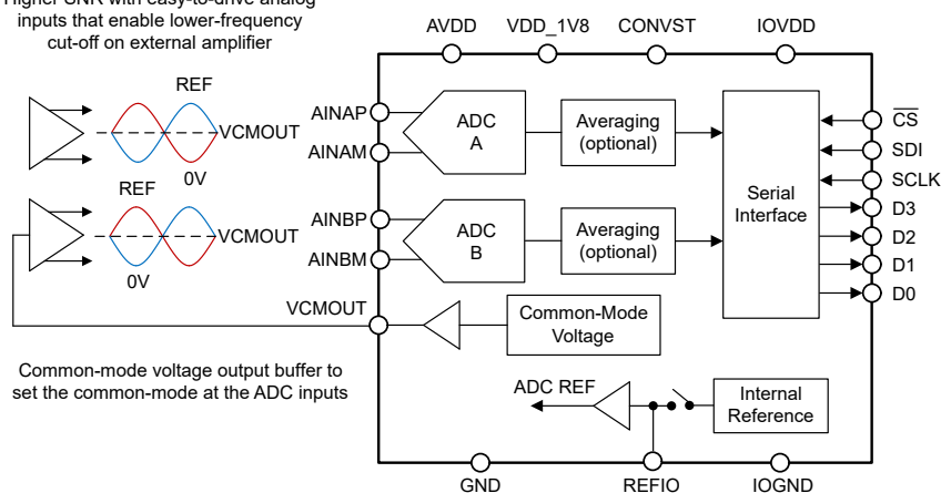
器件方框图
