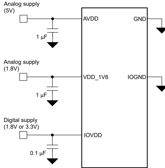
图 10-2. 电源去耦
