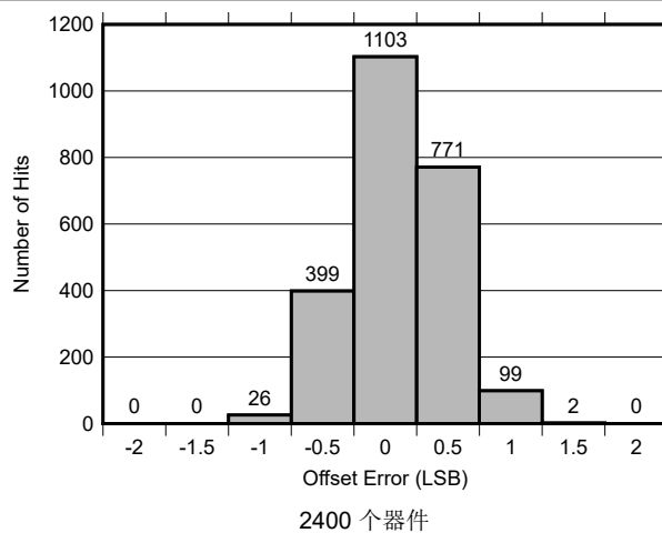
图 6-8. 典型偏移误差分布 (LSB)
