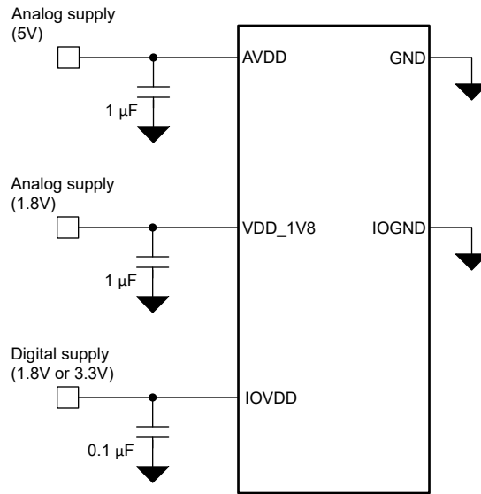
图 10-2. 电源去耦
