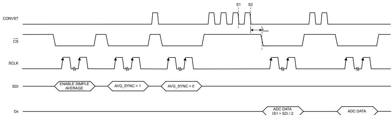
图 7-11. 非连续 CONVST 模式下简单平均启用时序 (2 样本均值)
