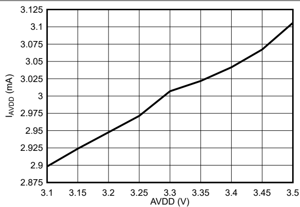
图 6-29. 2.5V 基准下 AVDD 电流与 AVDD 电压间的关系
