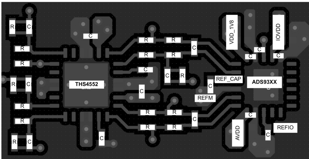
图 10-3. 示例布局
