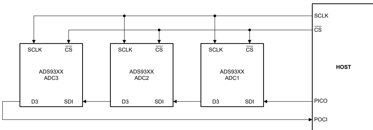
图 7-14. 菊花链连接
