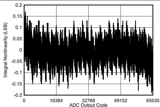
图 6-5. 典型 INL
