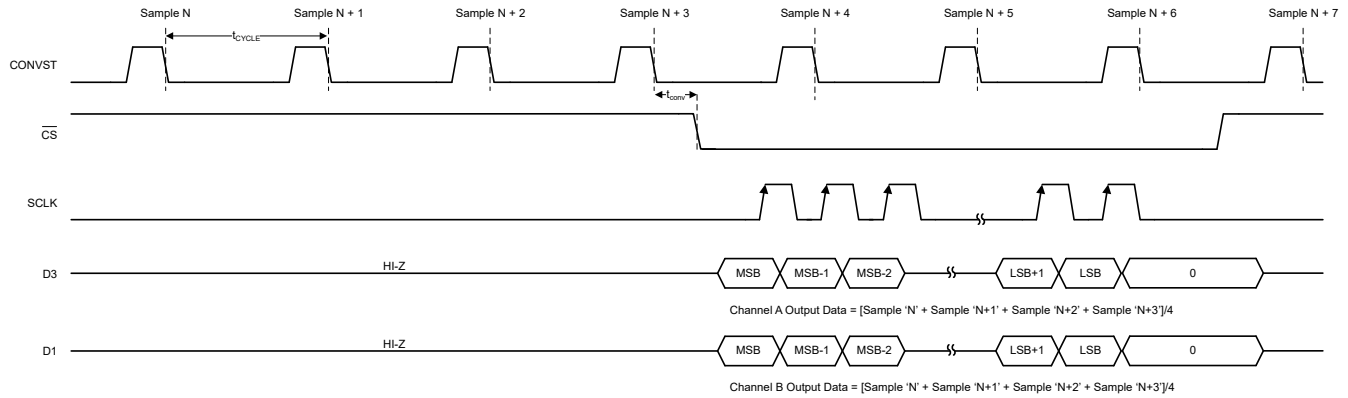
图 7-10. 在双通道数据接口模式下简单平均 4 个样本的 ADC 输出示例
