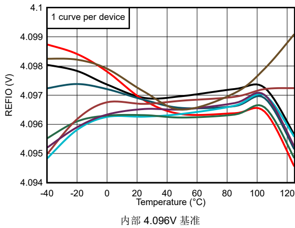
图 6-35. 4.096V 基准下 REFIO 电压与温度间的关系
