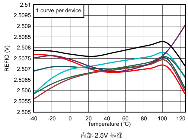
图 6-36. 2.5V 基准下 REFIO 电压与温度间的关系
