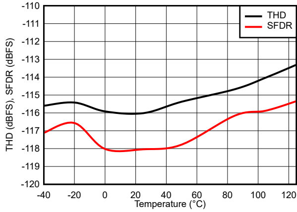
图 6-23. THD 和 SFDR 与温度间的关系
