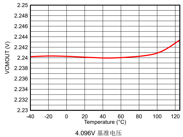
图 6-38. 4.096V 基准下 VCMOUT 电压与温度间的关系
