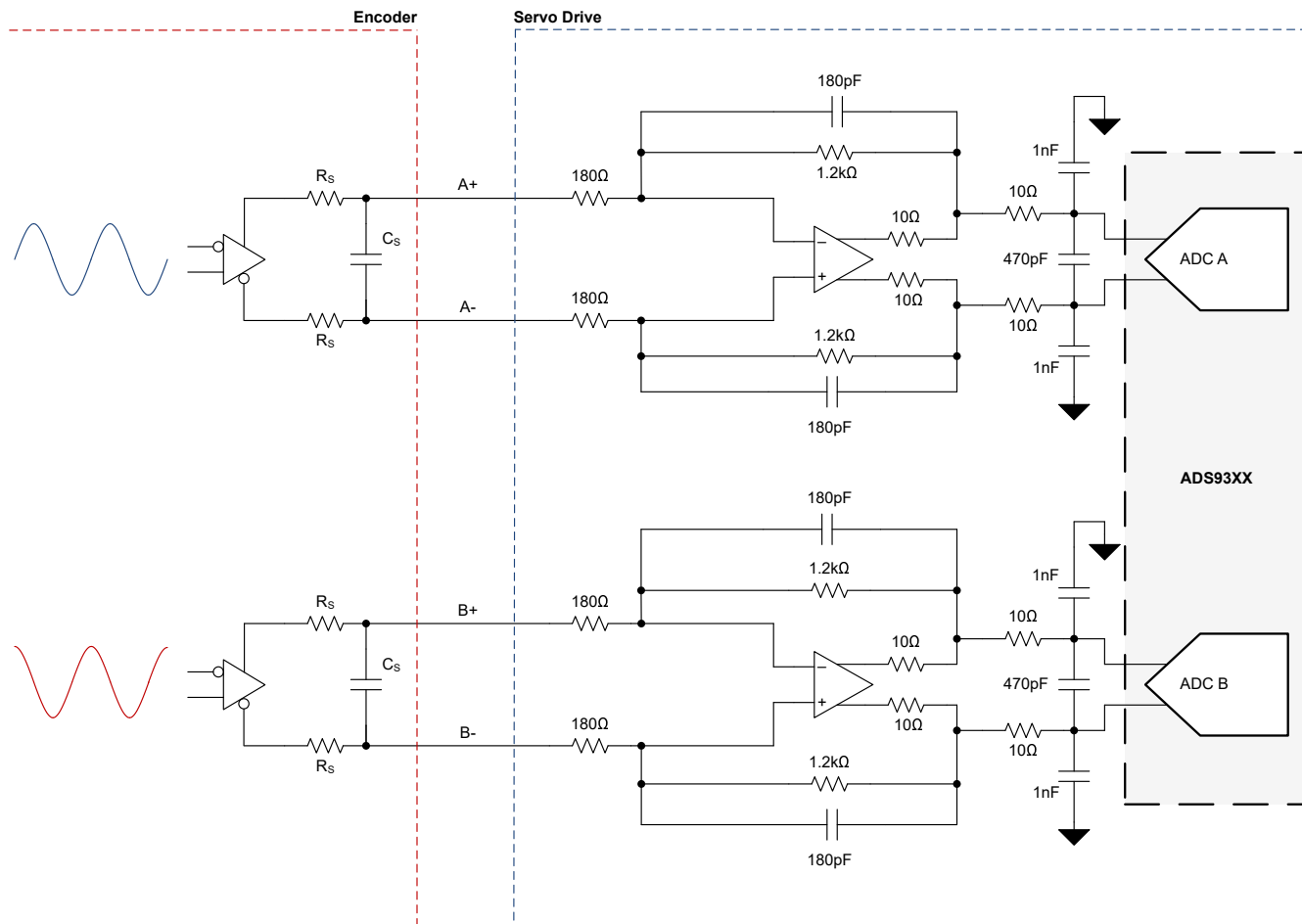
图 10-1. 具有 500kHz 输入信号带宽的正弦-余弦编码器接口电路
