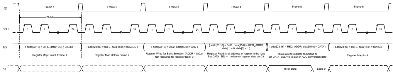
图 7-18. 寄存器读取
