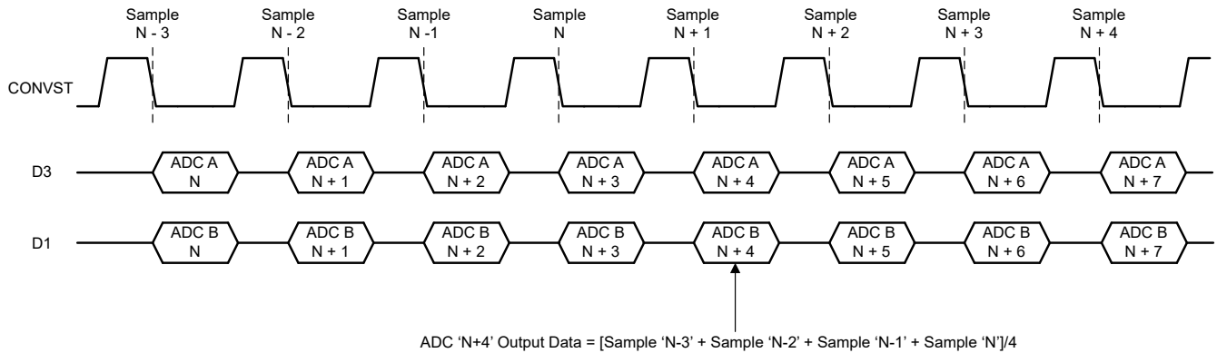
图 7-12. 移动平均 4 个样本的 ADC 输出示例
