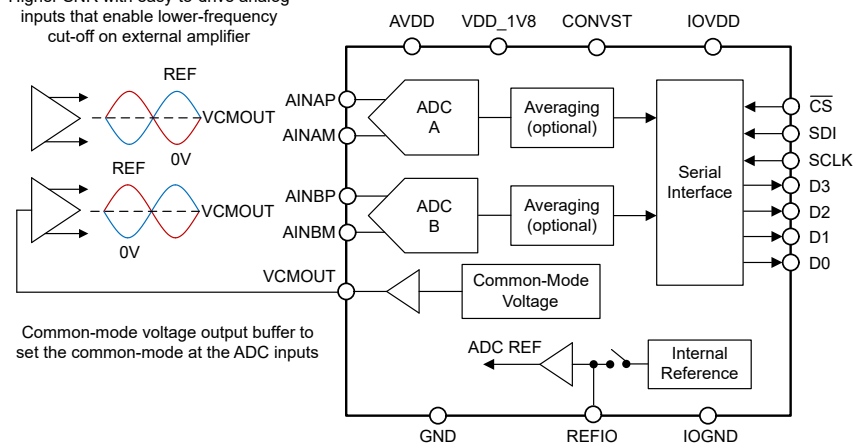
器件方框图
