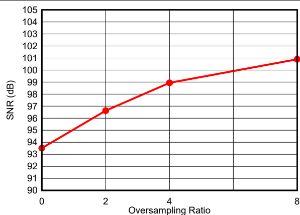
图 6-17. SNR 与移动平均过采样率间的关系
