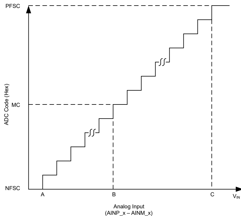
图 7-7. 传输特性
