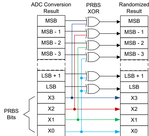
图 7-13. 使用 4 位 PRBS 的 XOR 操作
