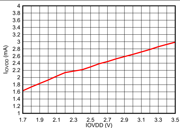
图 6-30. IOVDD 电流与 IOVDD 电压间的关系
