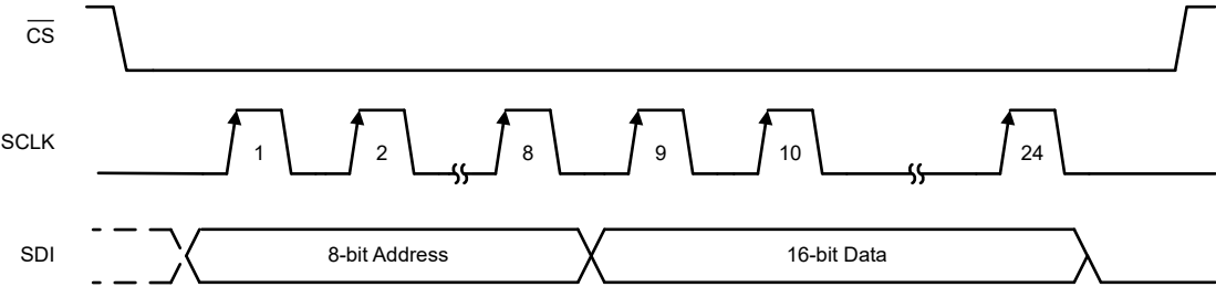
图 7-17. 寄存器写入帧
