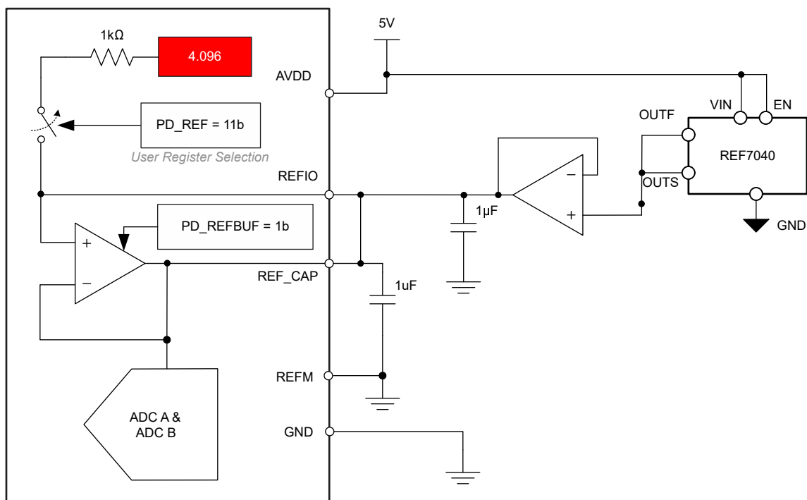
图 7-6. 采用外部基准缓冲器的外部基准
