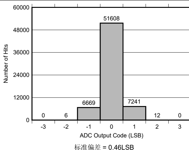
图 6-18. 直流输入直方图
