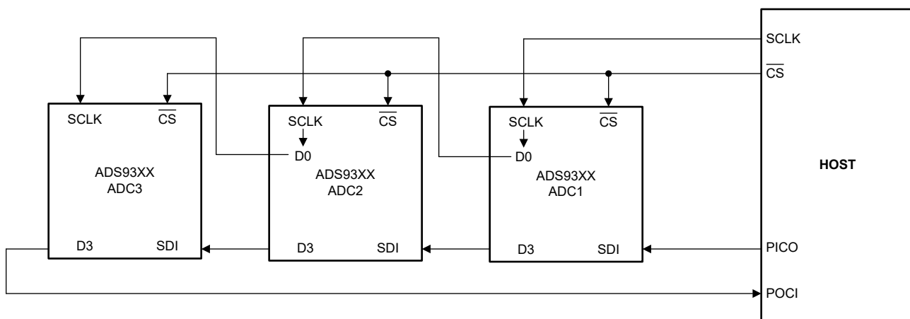
图 7-16. 启用菊花时钟模式时的菊花链连接
