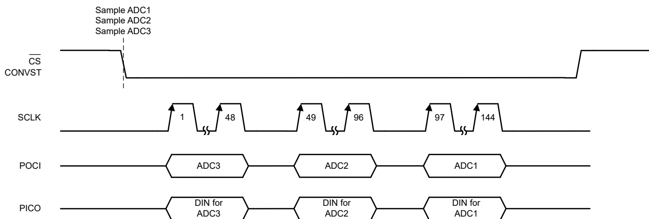
图 7-15. 简化的菊花链时序
