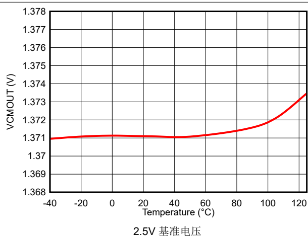
图 6-39. 2.5V 基准下 VCMOUT 电压与温度间的关系
