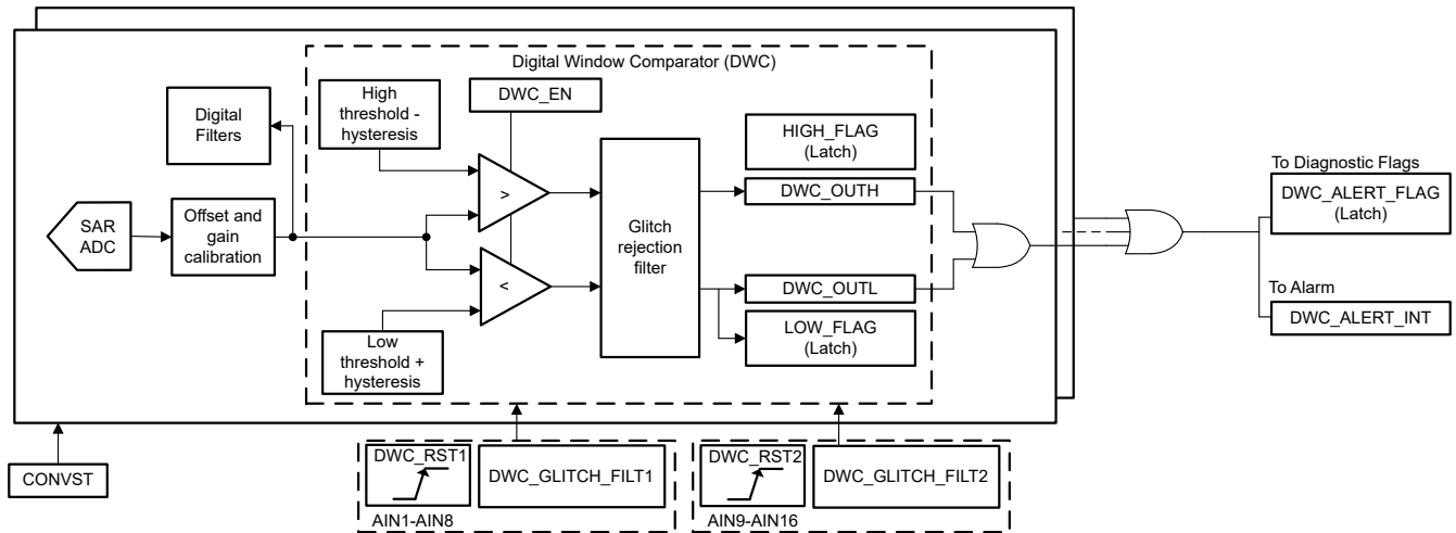
图 7-23. 数字窗口比较器功能方框图
