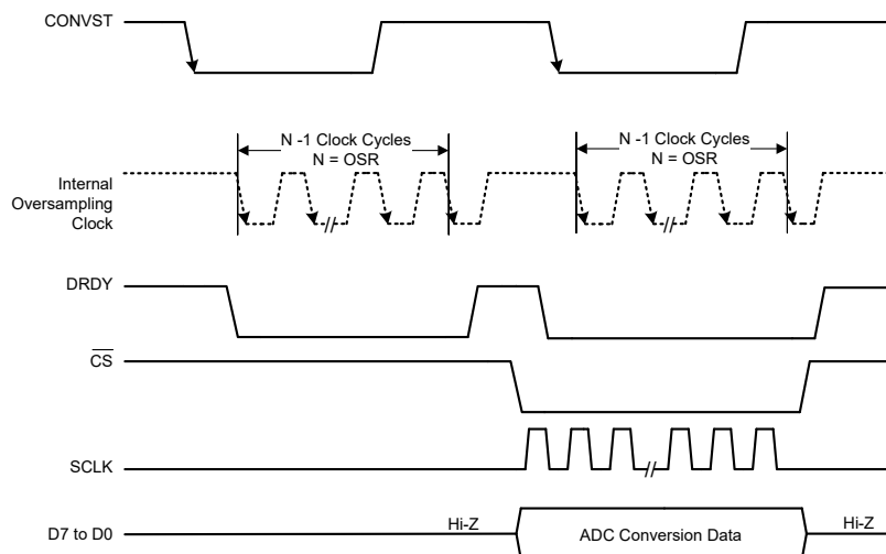
图 7-16. 内部过采样时钟
