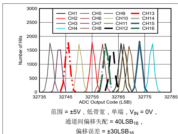
图 7-10. ADC 校准前的偏移误差
