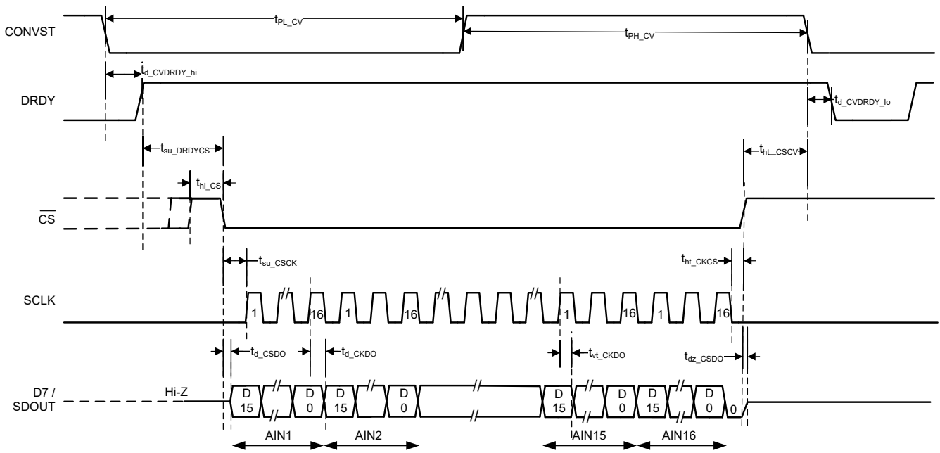
图 6-5. ADC 转换数据读取时序：1 通道
