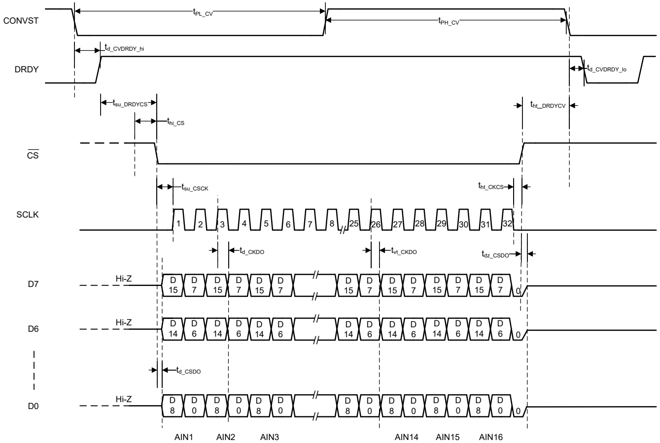
图 6-2. ADC 转换数据读取时序：8 通道（默认操作）
