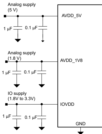
图 9-3. 电源去耦
