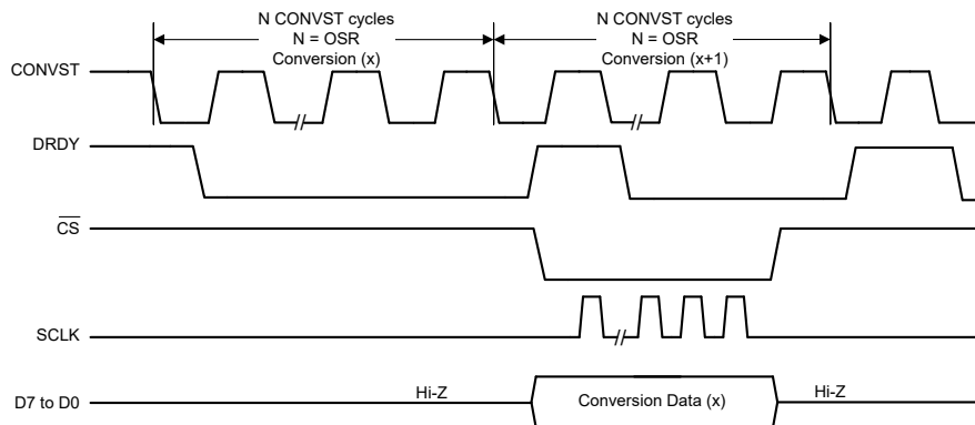
图 7-15. 外部过采样时钟
