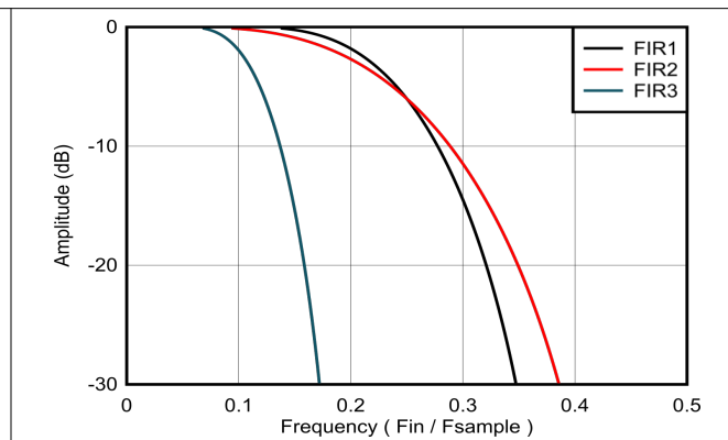
图 7-20. FIR1、FIR2 和 FIR3 滤波器频率响应，通带详细信息
