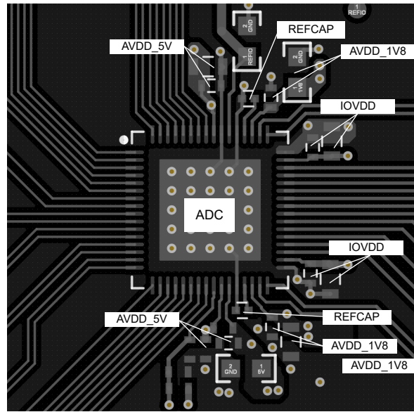
图 9-4. 示例布局
