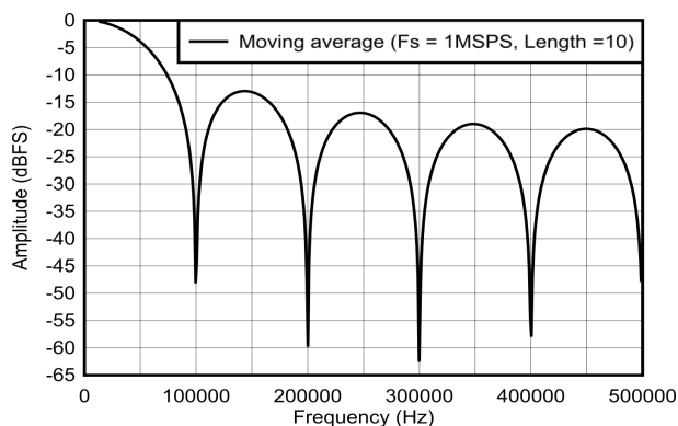
图 7-17. 移动平均值的频率响应 (长度 = 10)
