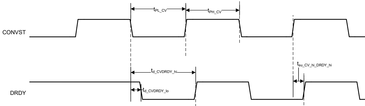
图 6-6. CONVST 和 DRDY，外部时钟过采样
