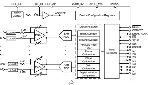
器件方框图
