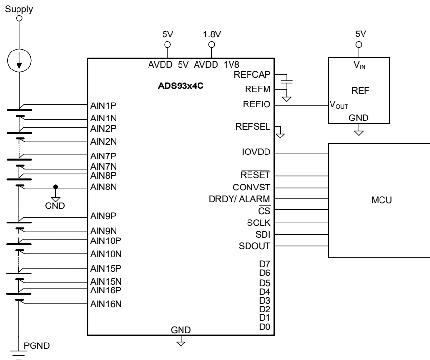
图 9-1. 使用 ADS9324C 进行 16 节串联电池电芯电压监控
