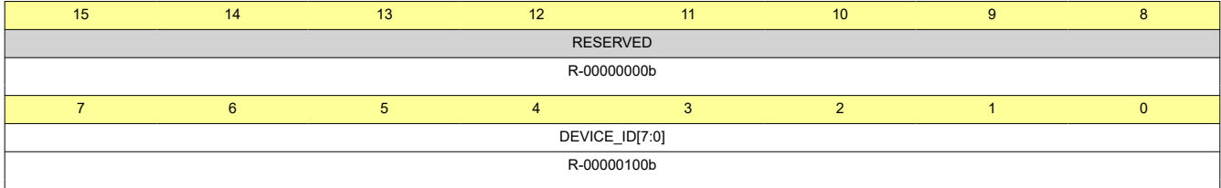
图 8-18. DEVICE_ID 寄存器
