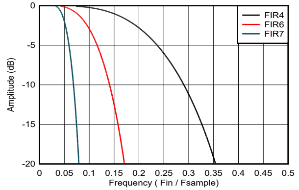
图 7-22. FIR4、FIR6 和 FIR7 滤波器频率响应，通带详细信息
