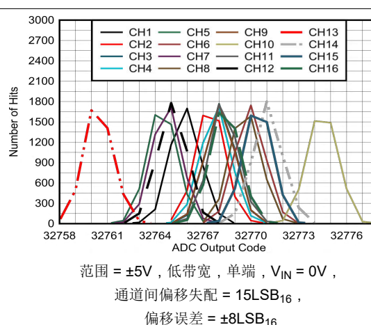
图 7-11. ADC 校准后的偏移误差
