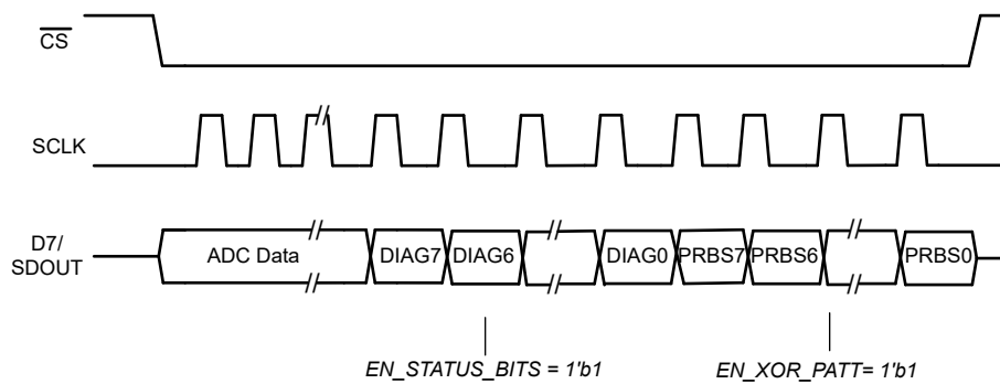
图 7-35. ADC 输出帧，1 通道模式
