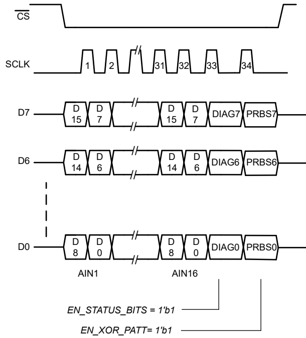
图 7-32. ADC 输出帧，8 通道模式
