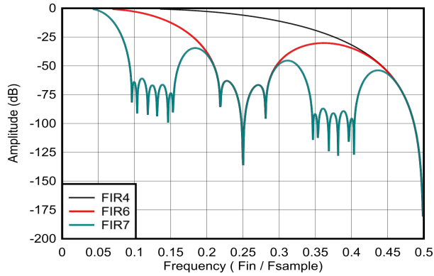
图 7-21. FIR4、FIR6 和 FIR7 滤波器频率响应
