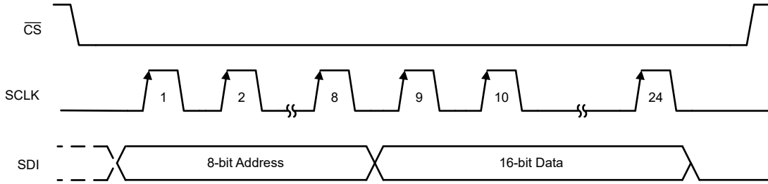
图 7-40. 寄存器写入帧
