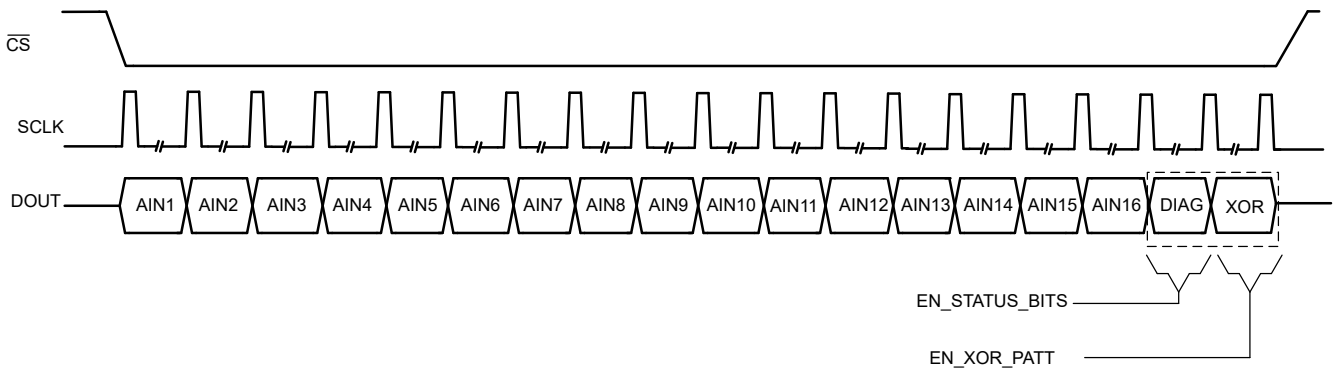
图 7-31. ADC 数据输出帧，已启用 DIAG_FLAG 和 XOR_PATT
