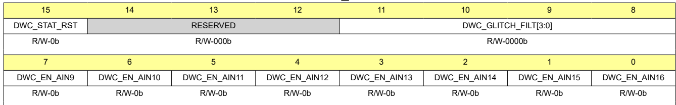
图 8-94. DWC_CFG 寄存器
