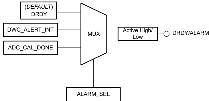
图 7-25. 警报功能框图
