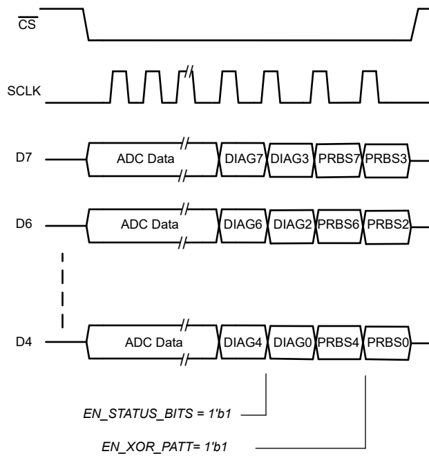
图 7-33. ADC 输出帧，4 通道模式
