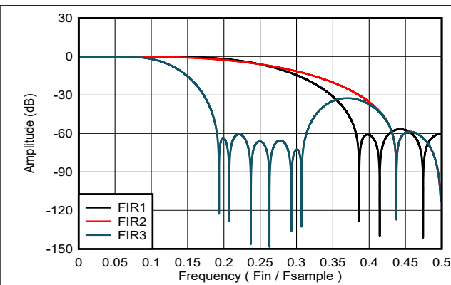
图 7-19. FIR1、FIR2 和 FIR3 滤波器频率响应
