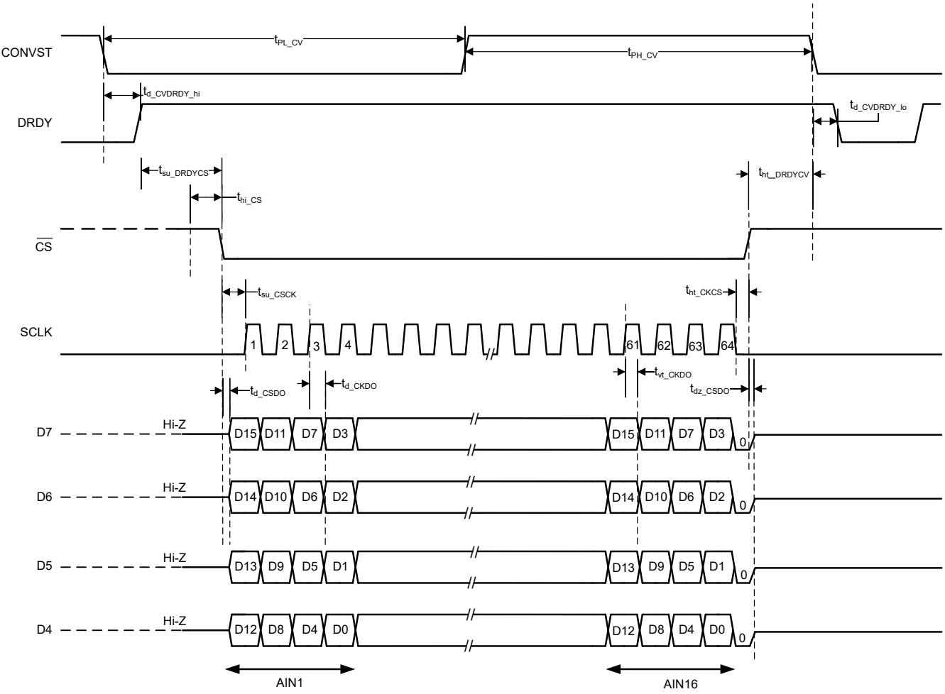
图 6-3. ADC 转换数据读取时序：4 通道
