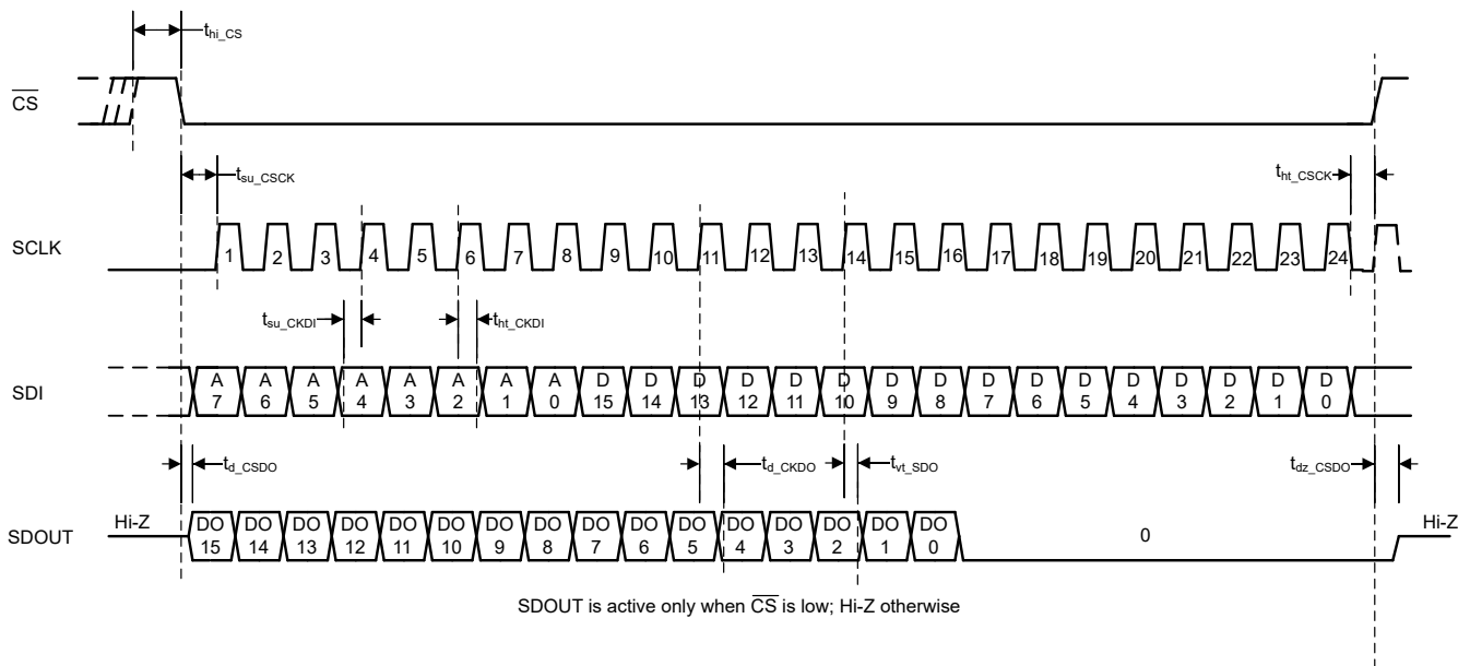
图 6-1. 寄存器读取和写入操作的时序
