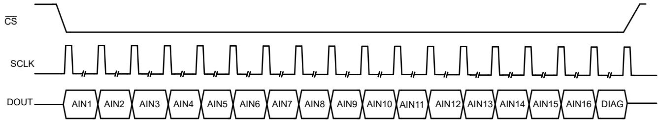
图 7-29. ADC 数据输出帧，DIAG_FLAG 已启用
