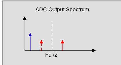
图 7-18. 使用低通数字滤波器实现抗混叠
