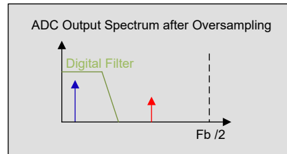
图 7-18. 使用低通数字滤波器实现抗混叠
