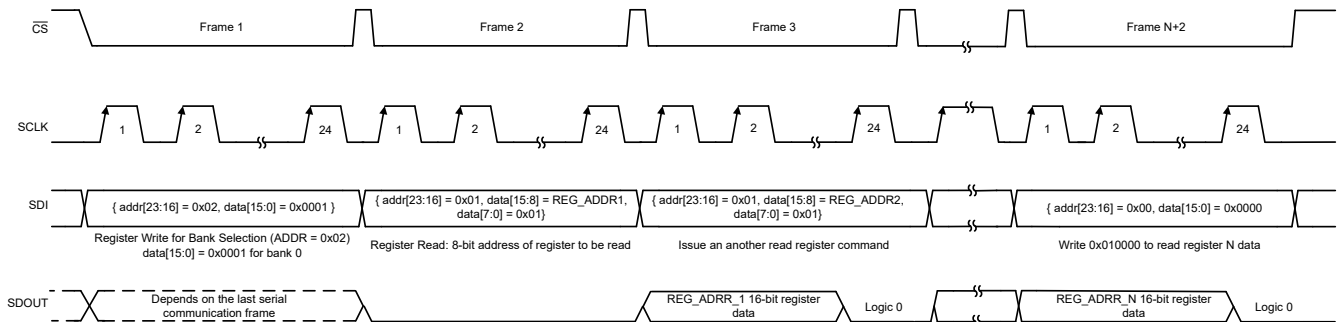
图 7-41. 寄存器读取
