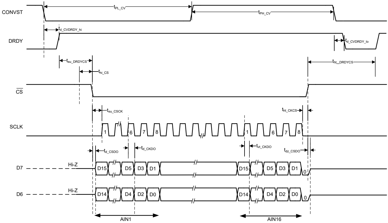
图 6-4. ADC 转换数据读取时序：2 通道
