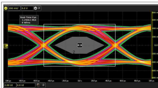
图 70. Eye 在 10-Gbps 位速率下具有默认输出摆幅
