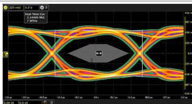
图 73. Eye 在 7.5-Gbps 位速率下具有增加输出摆幅
