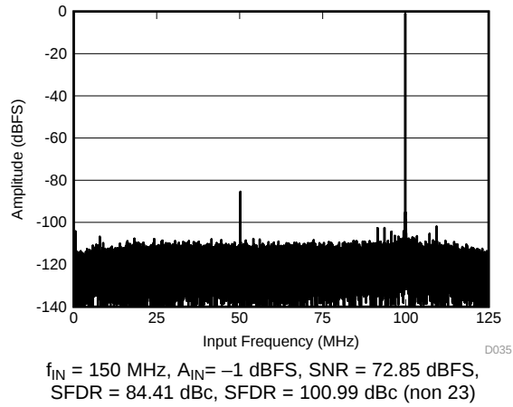
图 36. FFT for 150-MHz Input Signal
