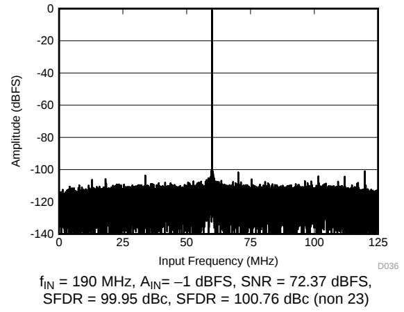
图 37. FFT for 190-MHz Input Signal
