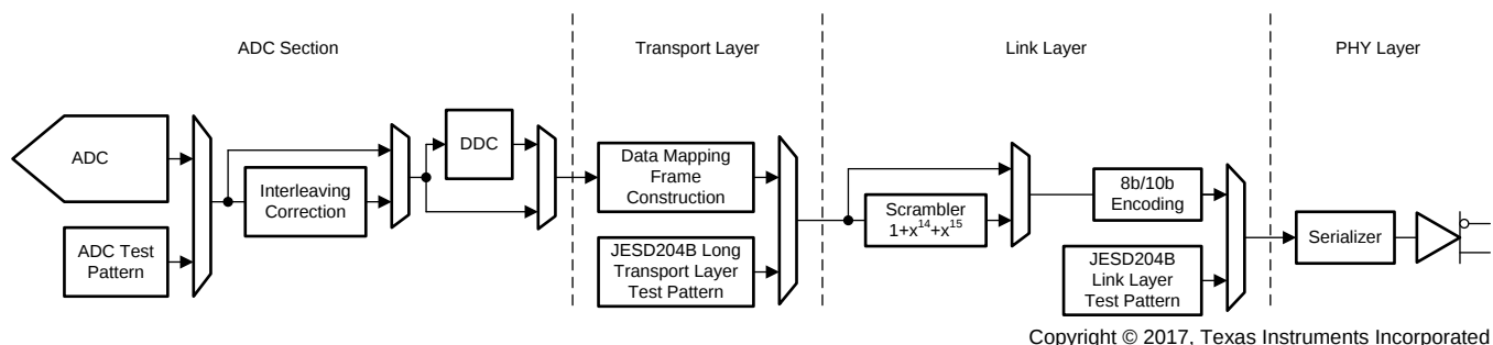
图 132. ADC Test Pattern
