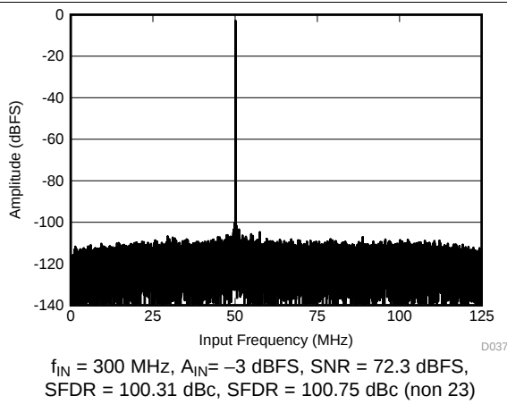
图 38. FFT for 300-MHz Input Signal
