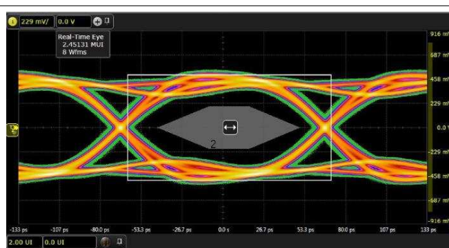
图 71. Eye 在 7.5-Gbps 位速率下具有默认输出摆幅
