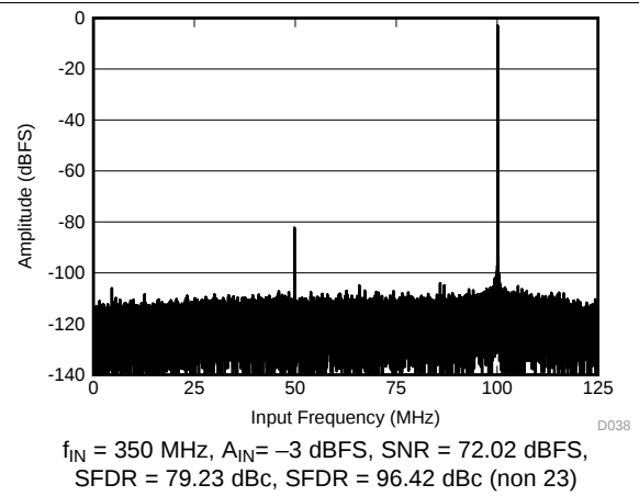
图 39. FFT for 350-MHz Input Signal
