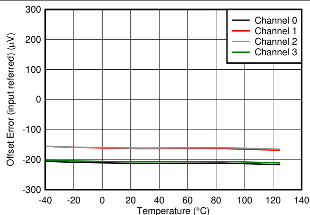
图 6-4. Offset Error vs Temperature
