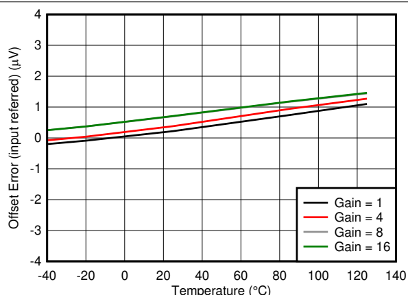
图 6-5. Offset Error vs Temperature
