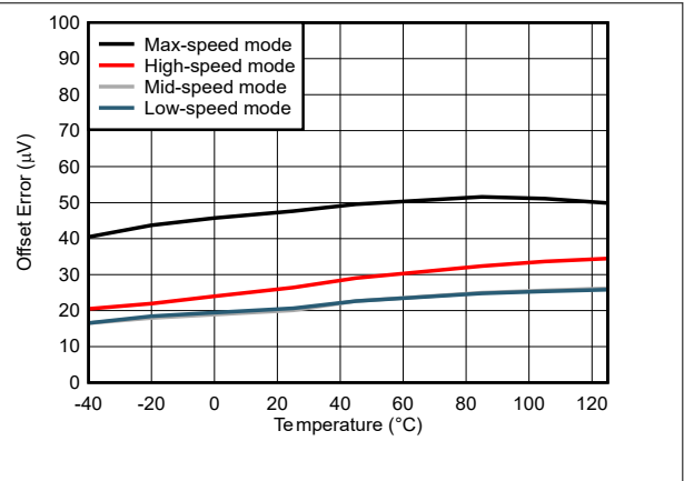
图 5-50. 偏移误差与温度间的关系
