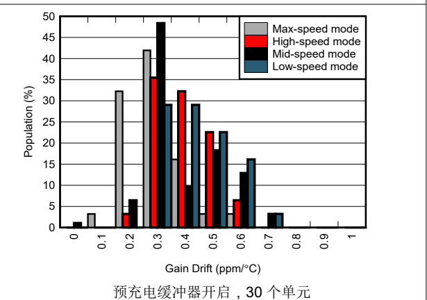
图 5-54. 增益漂移分布图
