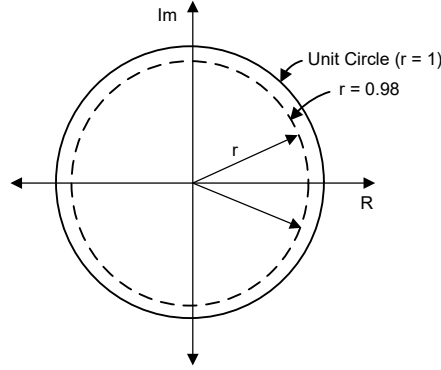
图 7-22. Z 平面
