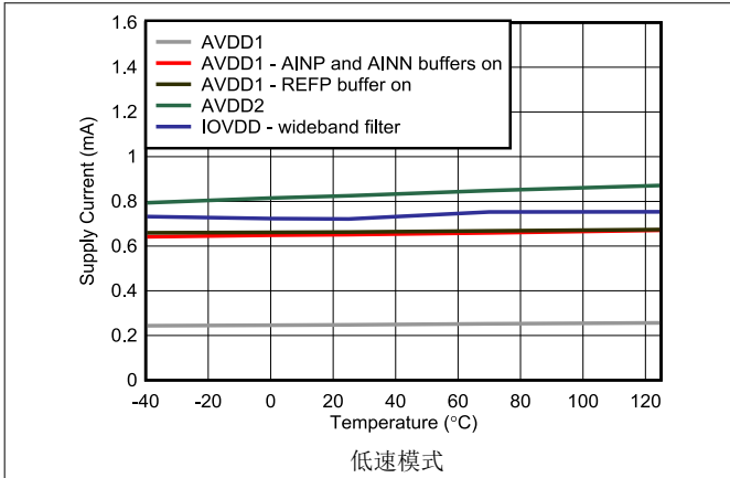
图 5-91. 电源电流与温度间的关系
