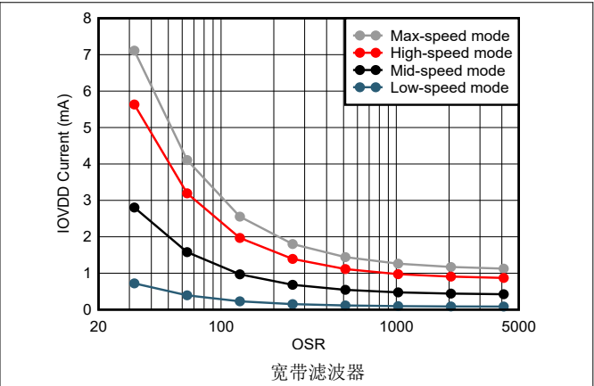
图 5-92. IOVDD 电流与过采样率间的关系
