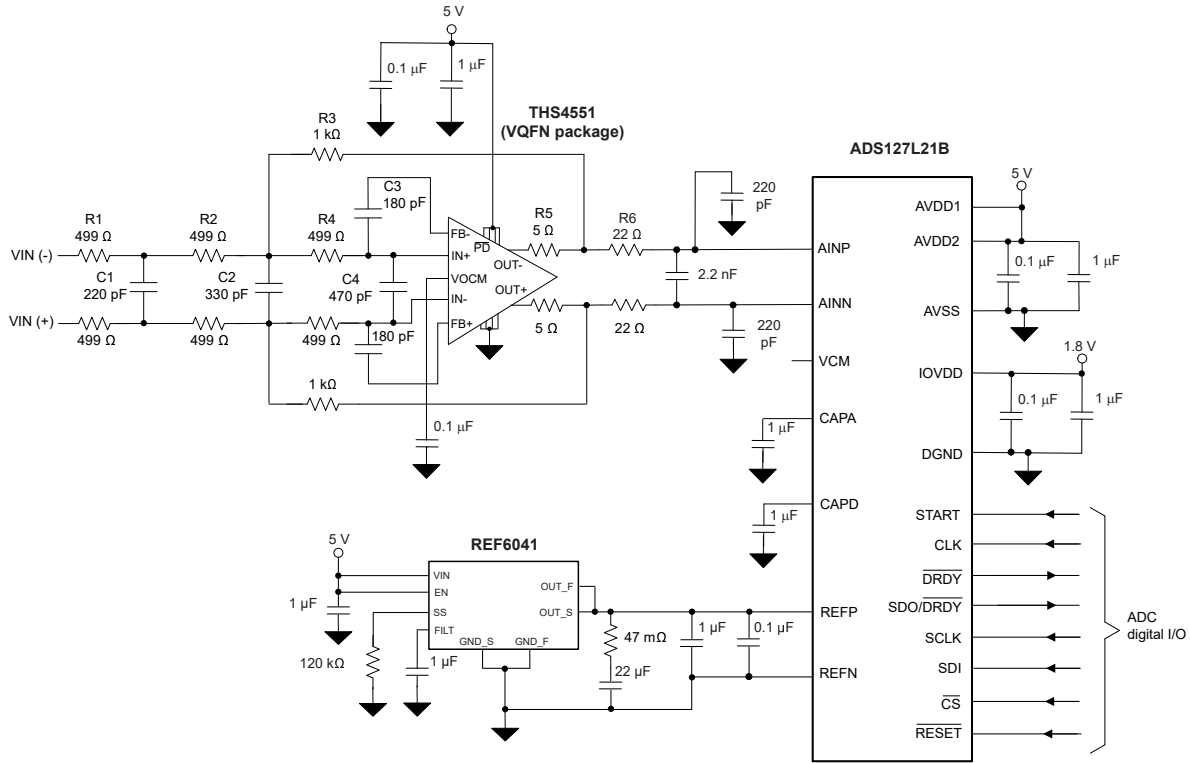
图 9-8. ADS127L21B 电路图
