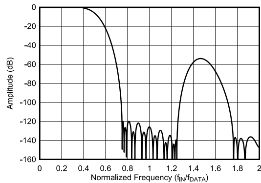
图 7-12. FIR2 滤波器频率响应 (OSR = 32)
