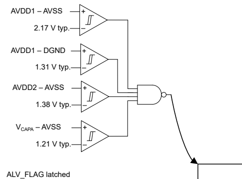
图 7-28. 模拟电源阈值
