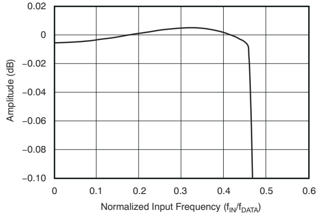
图 6-6. 高分辨率模式的通带响应
