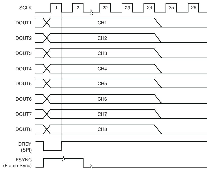
图 6-23. 离散数据输出模式
