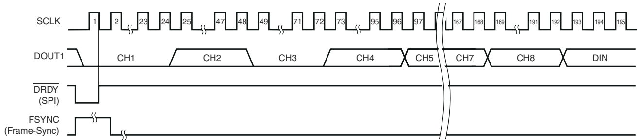
图 6-21. TDM 模式、固定位置数据 (显示通道 1 及 3 断电)
