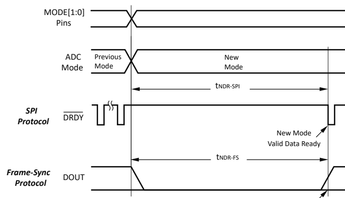
图 6-15. 模式更改时序
