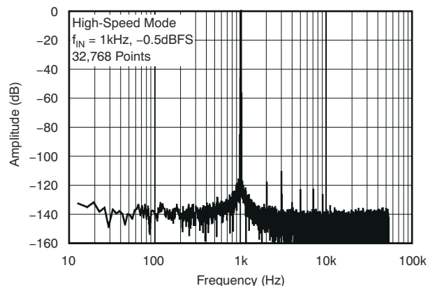
图 5-3. 输出频谱
