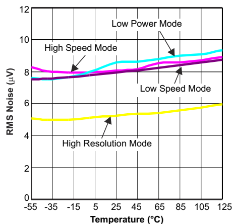
图 7-2. 噪声与温度间的关系
