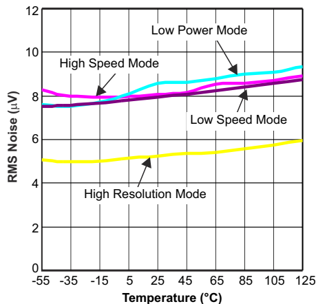
图 5-45. 噪声与温度间的关系
