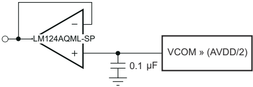
图 6-29. VCOM 输出
