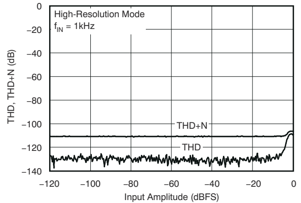
图 5-22. 总谐波失真与输入幅度间的关系
