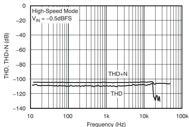
图 5-19. 总谐波失真与频率间的关系
