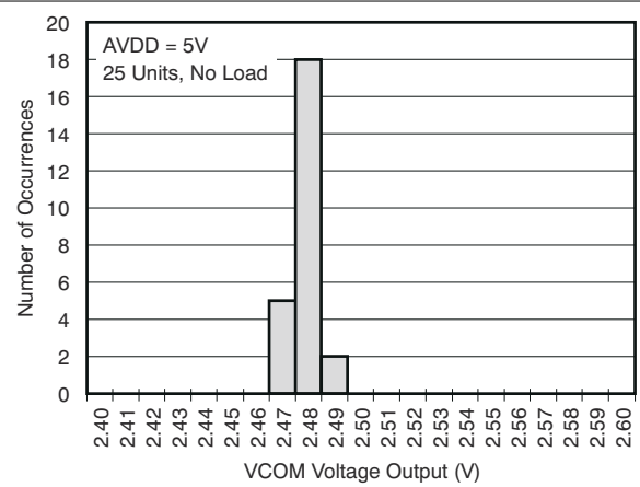
图 5-36. VCOM 电压输出直方图
