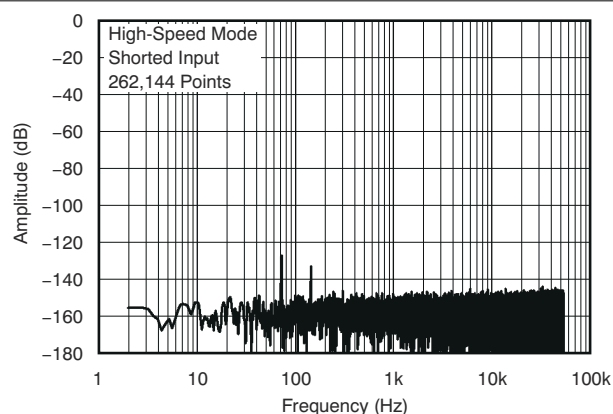
图 5-5. 输出频谱
