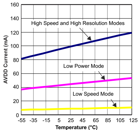
图 5-50. AVDD 电流与温度间的关系
