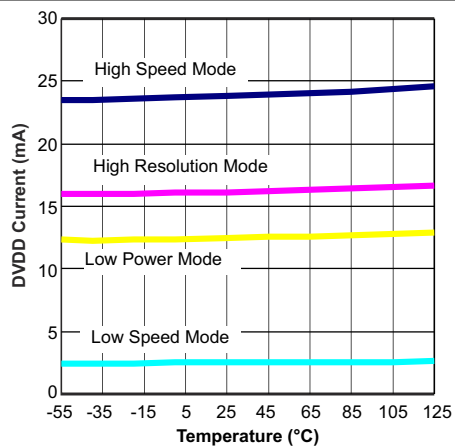
图 5-51. DVDD 电流与温度间的关系
