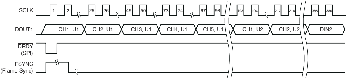
图 6-25. 图 6-24 的菊花链数据格式
