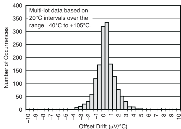
图 5-27. 温漂直方图
