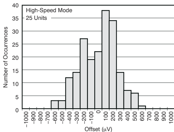
图 5-31. 失调电压误差直方图
