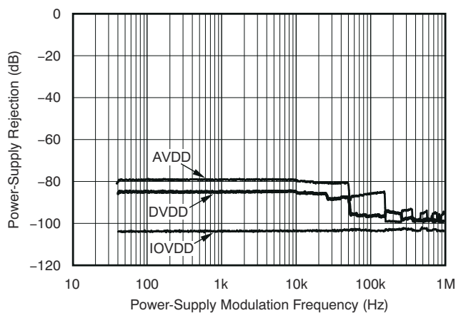
图 5-49. 电源抑制与电源频率间的关系
