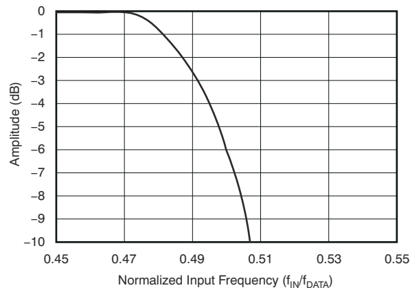
图 6-7. 高分辨率模式的过渡带响应
