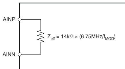
图 6-12. 有效输入阻抗
