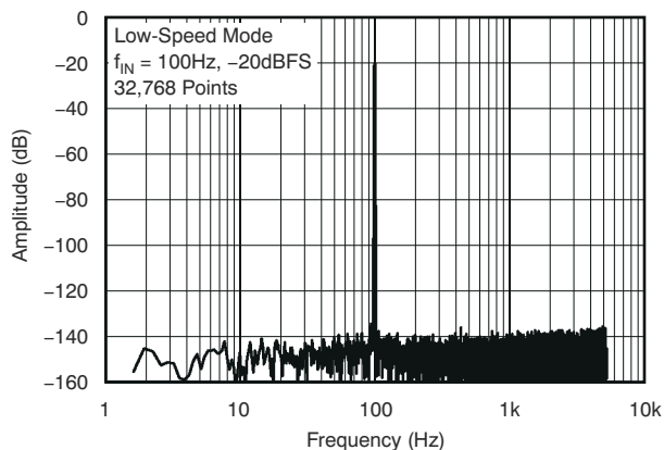
图 5-16. 输出频谱
