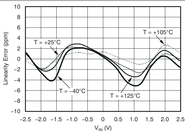
图 5-42. 线性误差与输入电平间的关系
