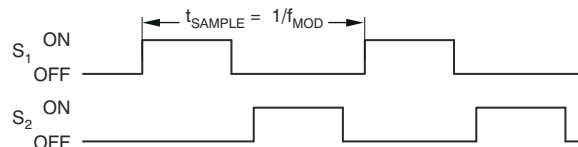
图 6-11. 图 6-10 的 S_1 和 S_2 开关时序
