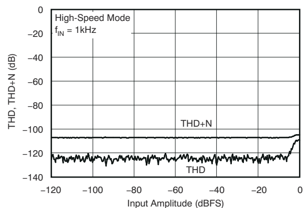
图 5-20. 总谐波失真与输入幅度间的关系
