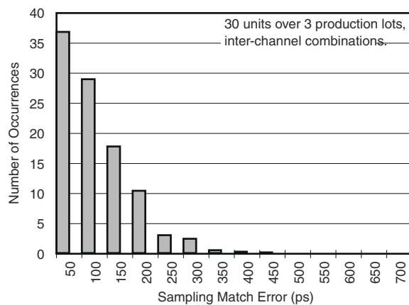
图 5-37. 采样匹配误差直方图
