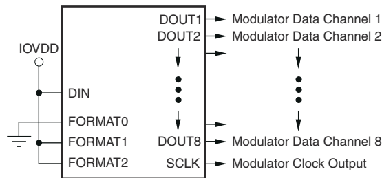
图 6-27. 调制器输出
