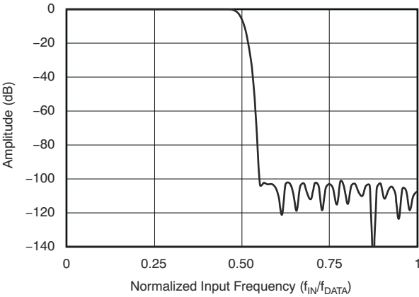
图 6-5. 高分辨率模式的频率响应
