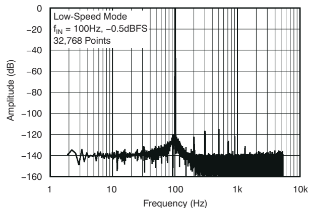
图 5-15. 输出频谱
