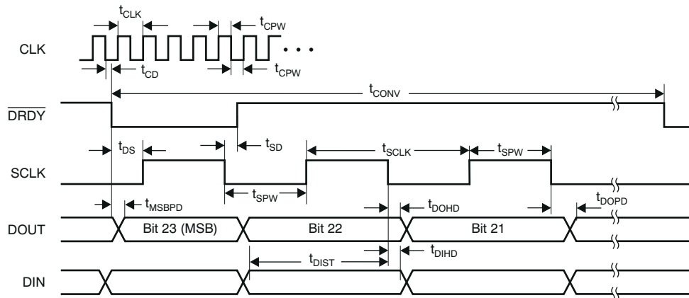
图 5-1. SPI 格式时序特点
