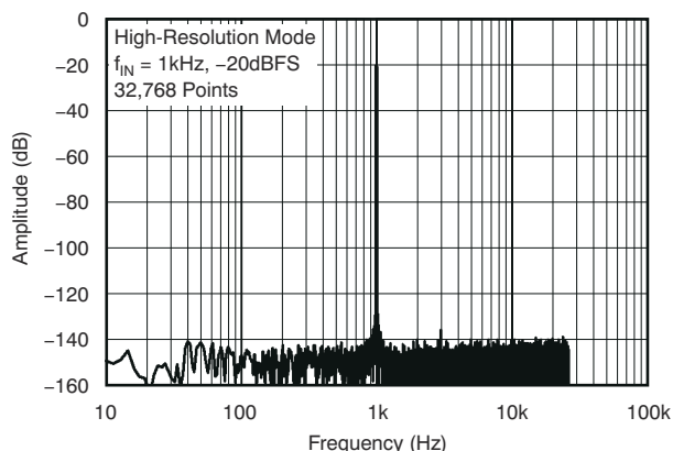
图 5-8. 输出频谱
