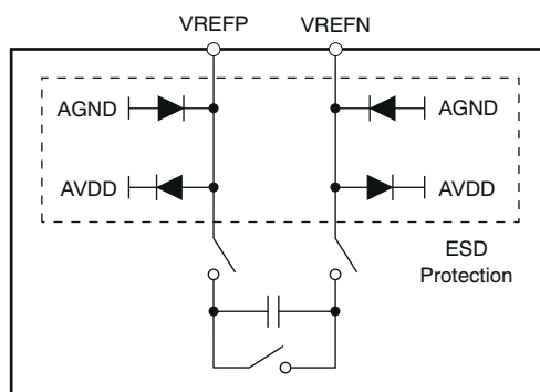
图 6-13. 等效基准输入电路
