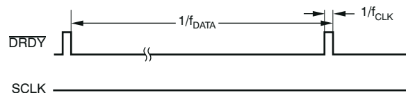
图 6-19. 无回读的 \overline{\text{DRDY}} 时序
