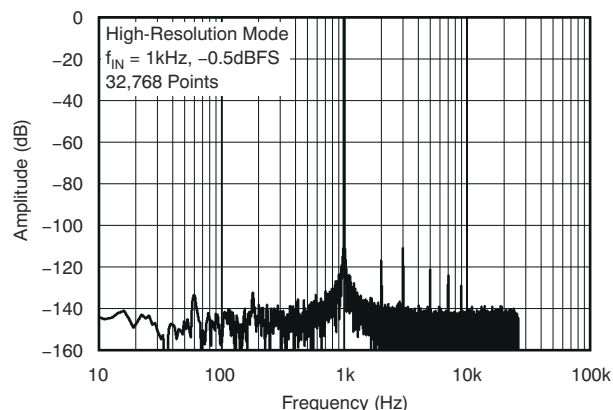
图 5-7. 输出频谱
