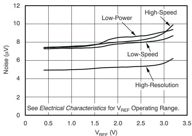
图 5-46. 噪声与基准电压间的关系
