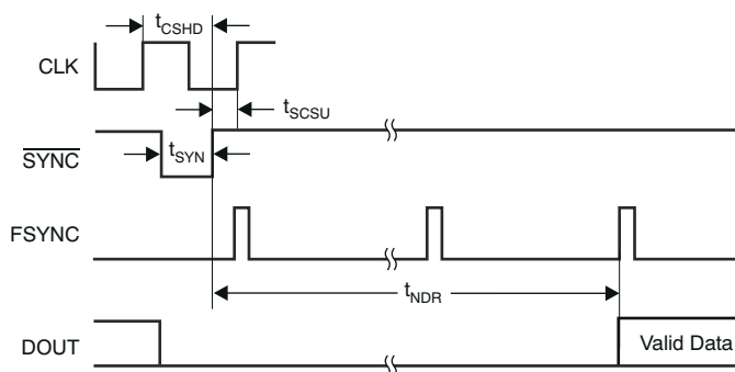
图 6-17. 同步时序 ( 帧同步协议 )
