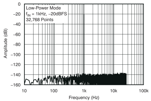
图 5-12. 输出频谱
