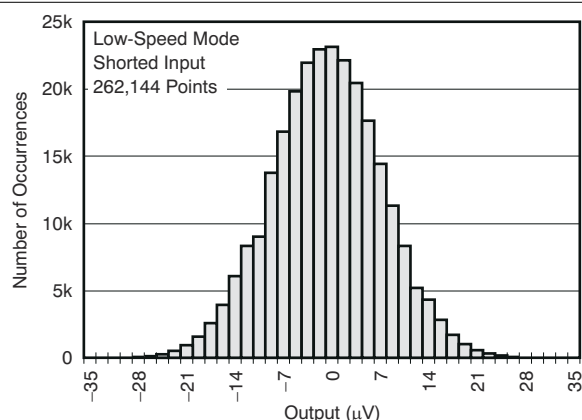
图 5-18. 噪声直方图
