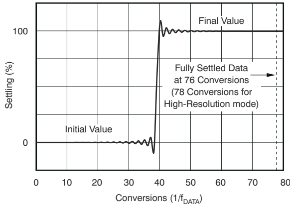
图 6-9. 阶跃响应
