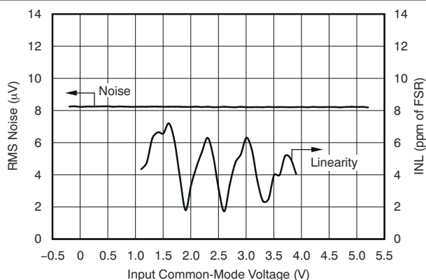
图 5-44. 噪声和线性与输入共模电压间的关系
