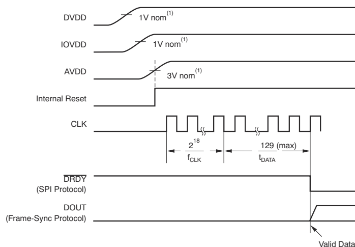
图 7-3. 启动序列
