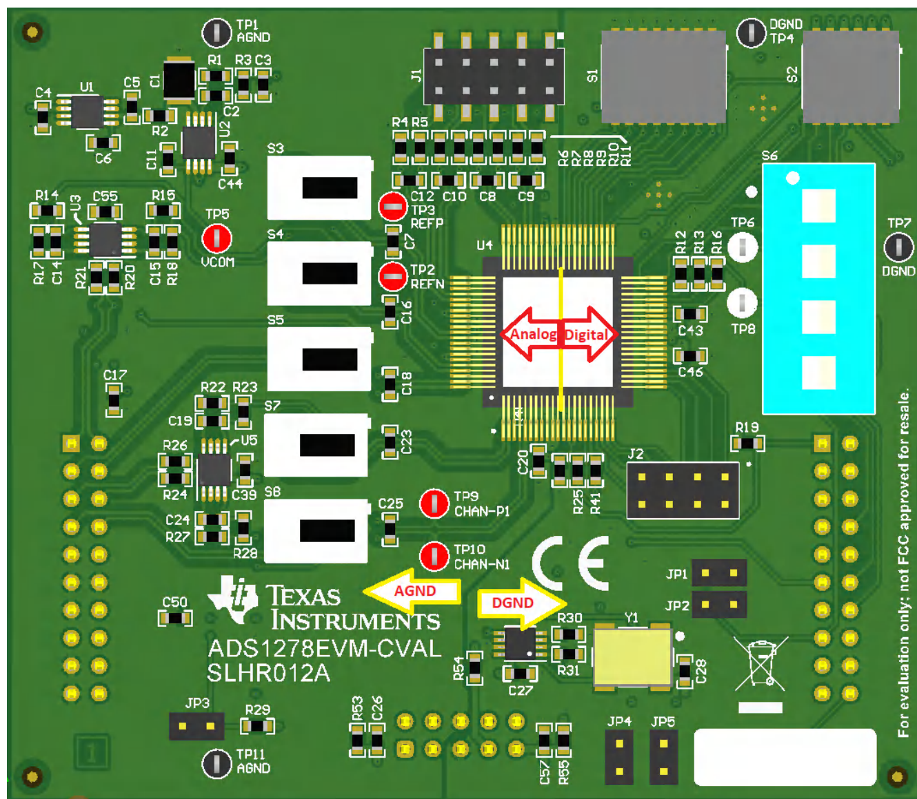
图 7-4. ADS1278QML-SP 布局示例
