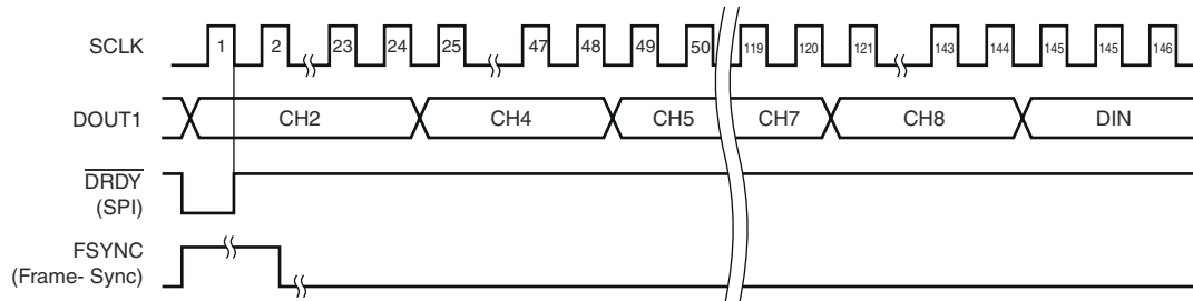
图 6-22. TDM 模式、动态位置数据 (显示通道 1 和 3 断电)
