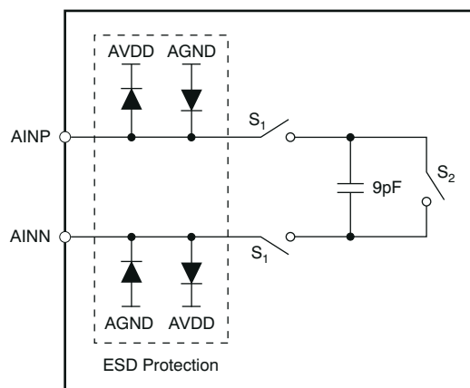
图 6-10. 等效模拟输入电路
