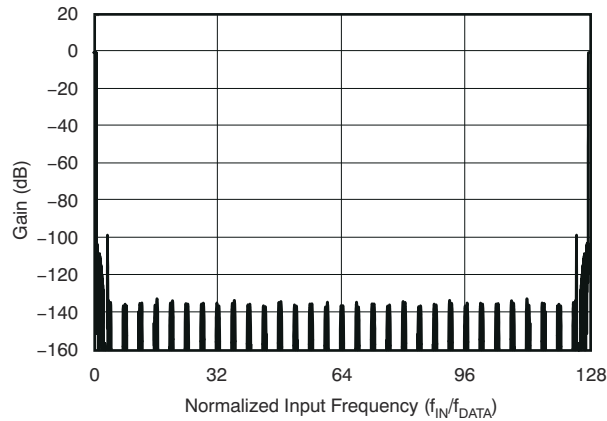
图 6-8. 高分辨率模式下 F_{MOD} 的频率响应
