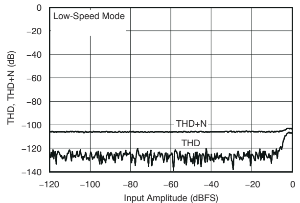
图 5-26. 总谐波失真与输入幅度间的关系
