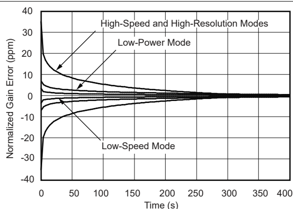
图 5-30. 增益预热漂移响应频带
