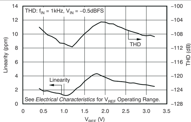
图 5-43. 线性和总谐波失真与基准电压间的关系
