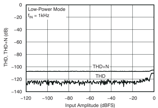
图 5-24. 总谐波失真与输入幅度间的关系
