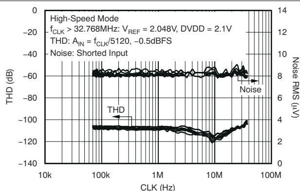
图 5-47. 总谐波失真和噪声与 CLK 间的关系
