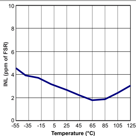
图 5-41. 积分非线性与温度间的关系
