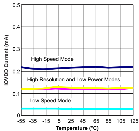
图 5-52. IOVDD 电流与温度间的关系
