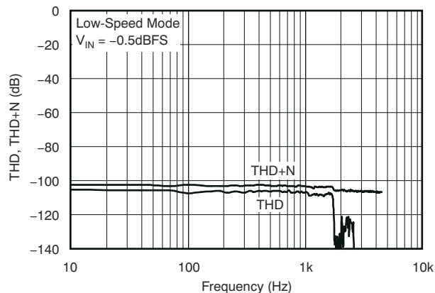
图 5-25. 总谐波失真与频率间的关系
