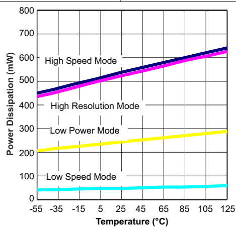
图 5-53. 功耗与温度间的关系
