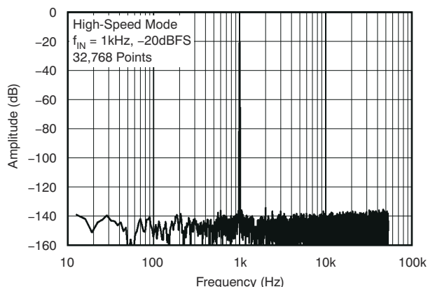
图 5-4. 输出频谱
