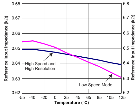
图 5-38. 基准输入差分阻抗与温度间的关系
