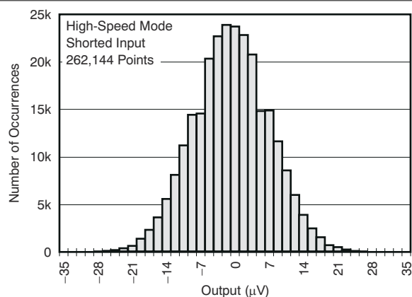
图 5-6. 噪声直方图
