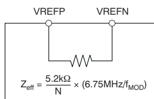
图 6-13. 等效基准输入电路
