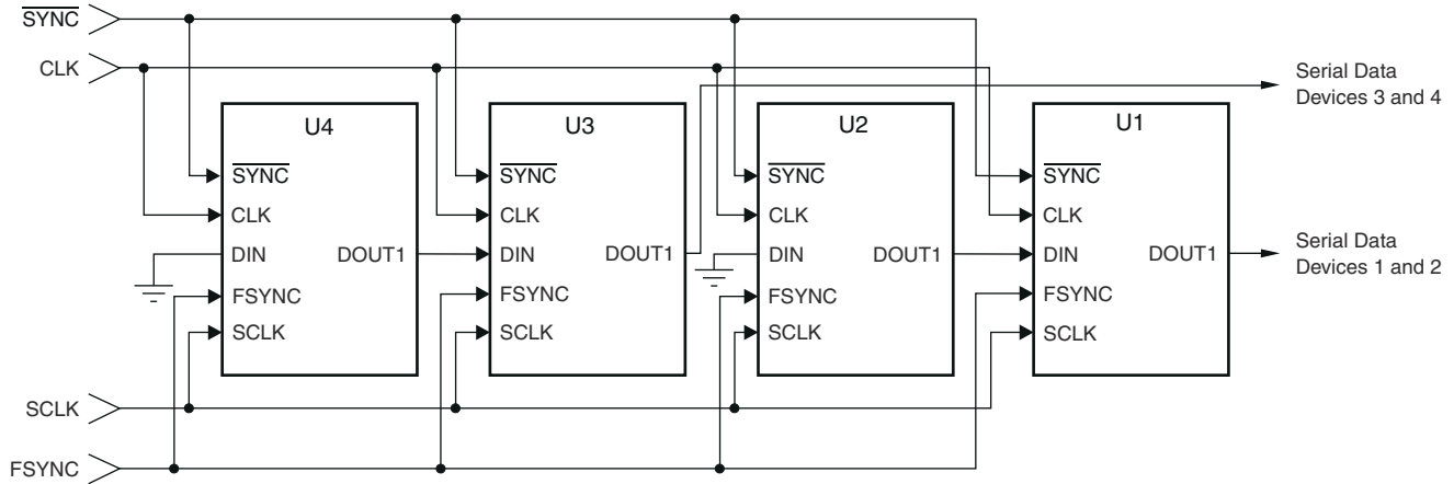
图 6-26. 分段式 DOUT 菊花链、帧同步协议 ( Format[2:0] = 011 或 100 )
