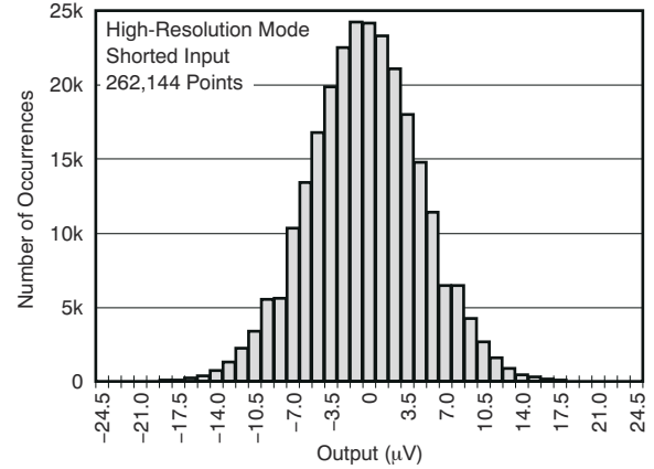
图 5-10. 噪声直方图
