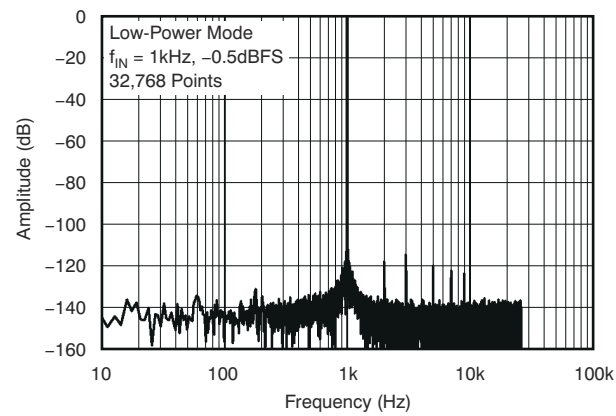
图 5-11. 输出频谱
