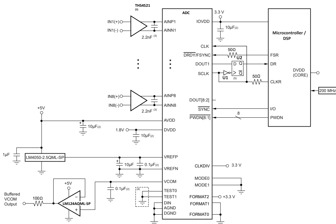
图 7-1. 典型应用原理图
