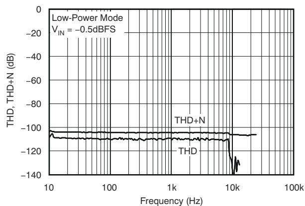
图 5-23. 总谐波失真与频率间的关系
