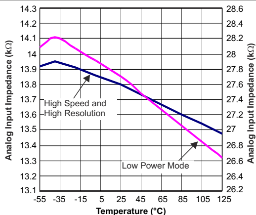
图 5-39. 模拟输入差分阻抗与温度间的关系
