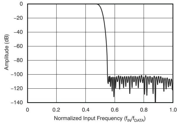
图 6-1. 高速、低功耗及低速模式的频率响应
