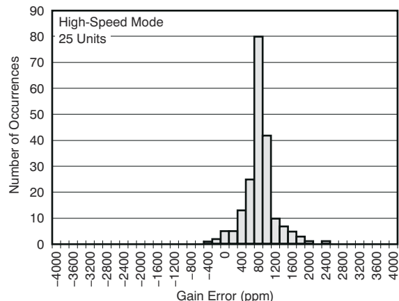
图 5-32. 增益误差直方图
