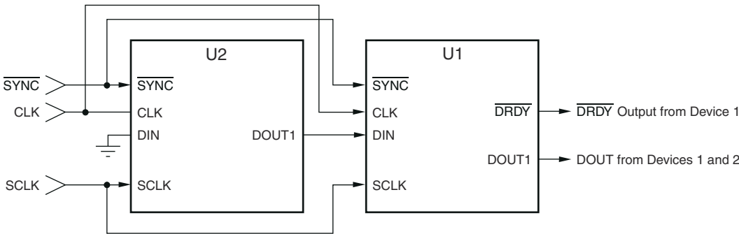
图 6-24. 两个器件的菊花链、SPI 协议 (Format[2:0] = 000 或 001)
