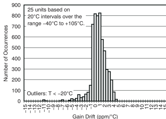
图 5-28. 增益漂移直方图
