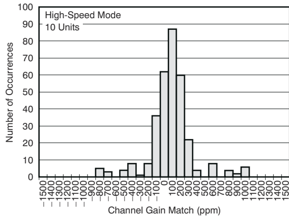
图 5-33. 通道增益匹配直方图
