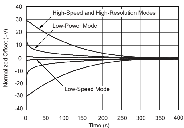
图 5-29. 偏移预热漂移响应带
