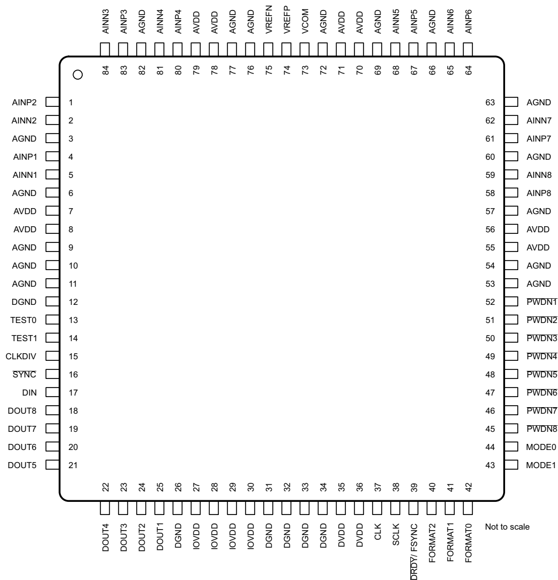
图 4-1. HFQ 封装 84 引脚 CFP 顶视图
