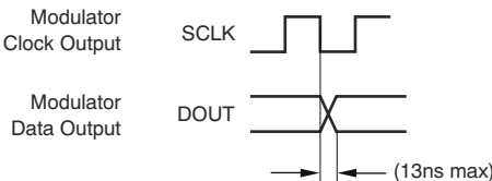
图 6-28. 调制器输出时序
