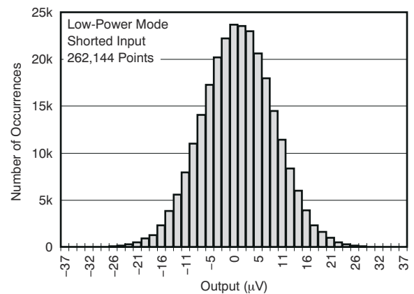
图 5-14. 噪声直方图
