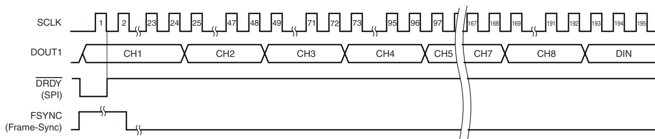
图 6-20. TDM 模式 (启用所有通道)
