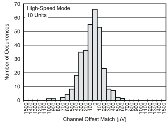
图 5-34. 通道失调电压匹配直方图
