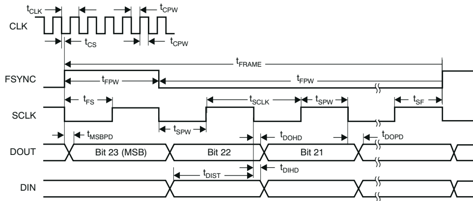
图 5-2. 帧同步格式计时特点
