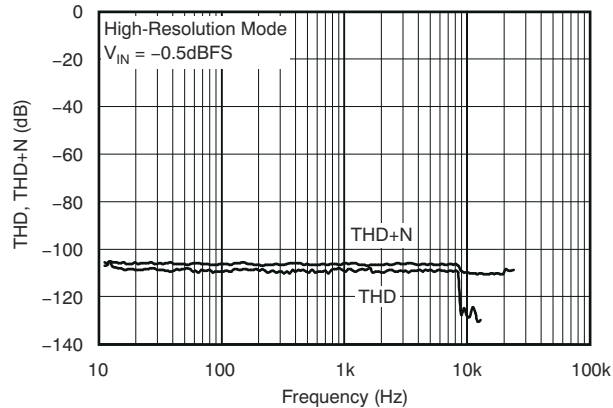
图 5-21. 总谐波失真与频率间的关系
