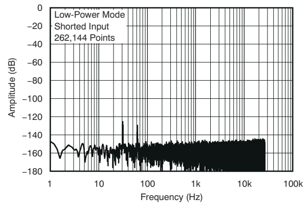
图 5-13. 输出频谱
