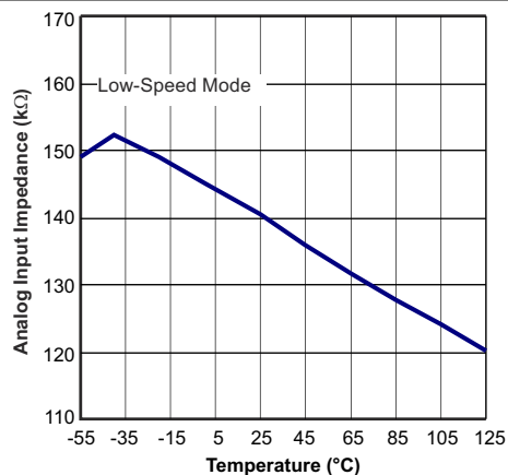
图 5-40. 模拟输入差分阻抗与温度间的关系
