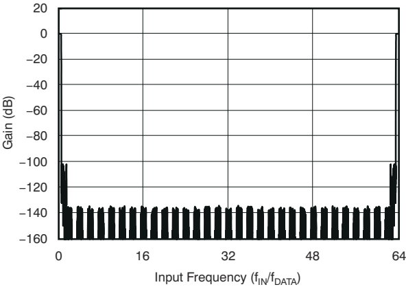
图 6-4. 高速、低功耗和低速模式下 F_{MOD} 的频率响应
