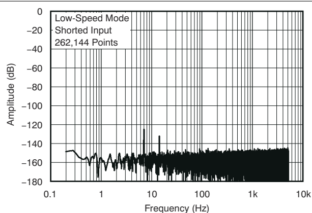
图 5-17. 输出频谱
