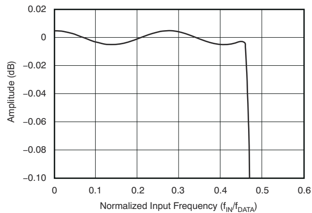
图 6-2. 高速、低功耗及低速模式的通带响应
