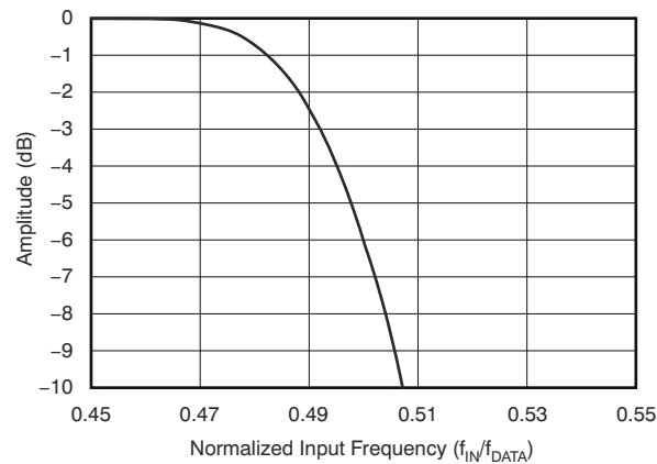
图 6-3. 高速、低功耗及低速模式的过渡带响应
