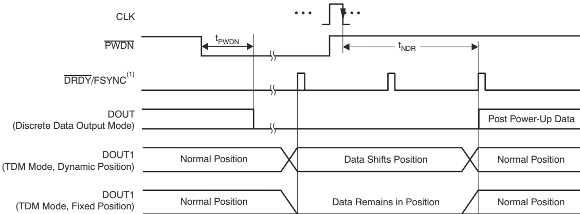
图 6-18. 断电时序
