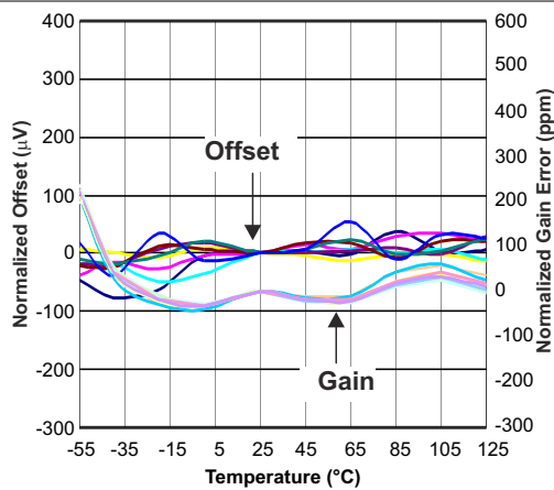
图 5-35. 偏移和增益与温度间的关系
