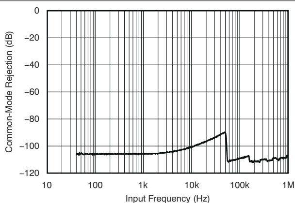
图 5-48. 共模抑制与输入频率间的关系
