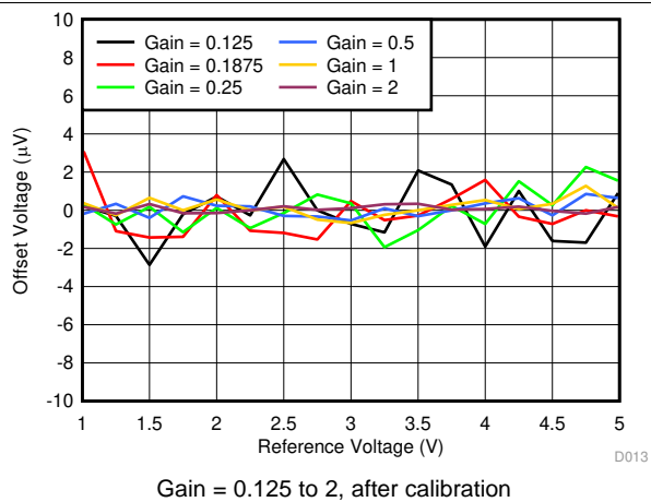
图 29. Offset Voltage vs Reference Voltage
