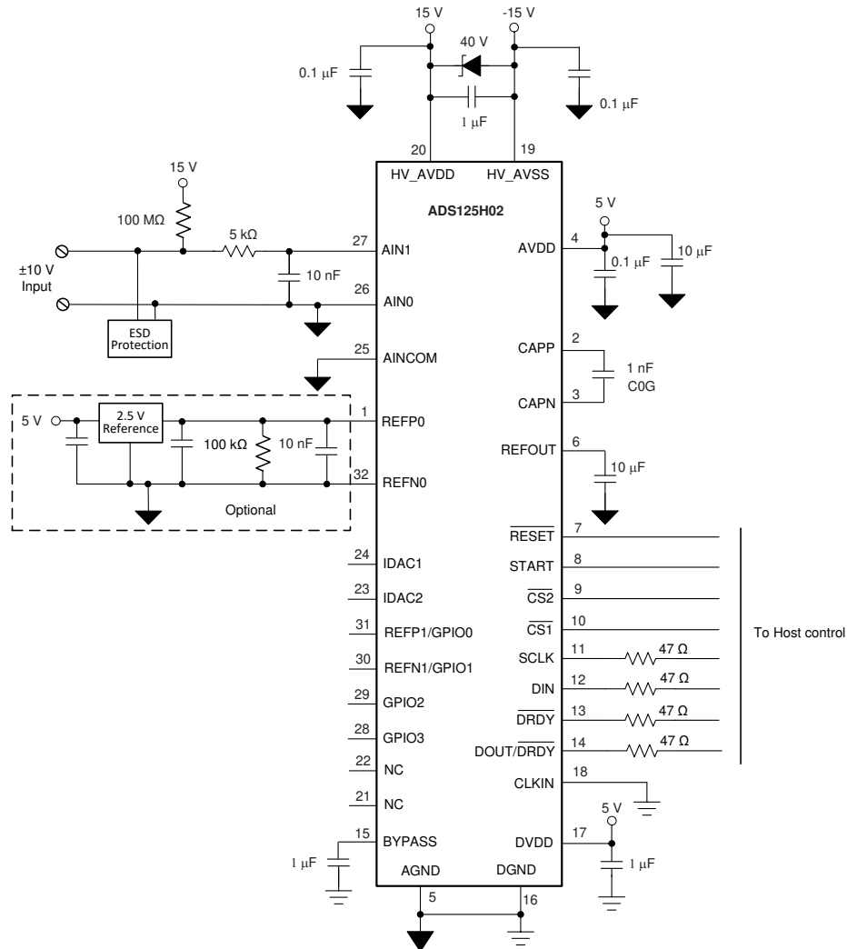
图 98. \pm 10 -V Analog Input PLC Module
