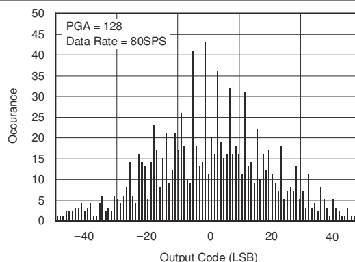
图 5-8. Noise Histogram
