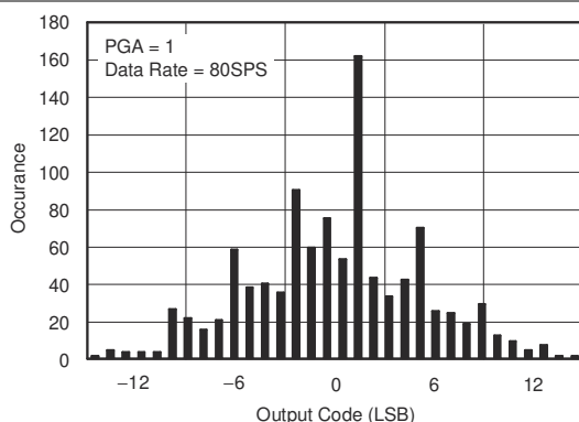
图 5-7. Noise Histogram
