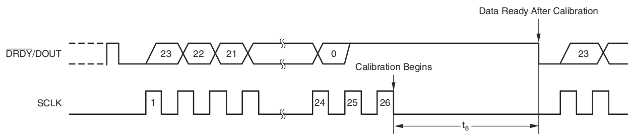
图 7-11. Offset-Calibration Timing
