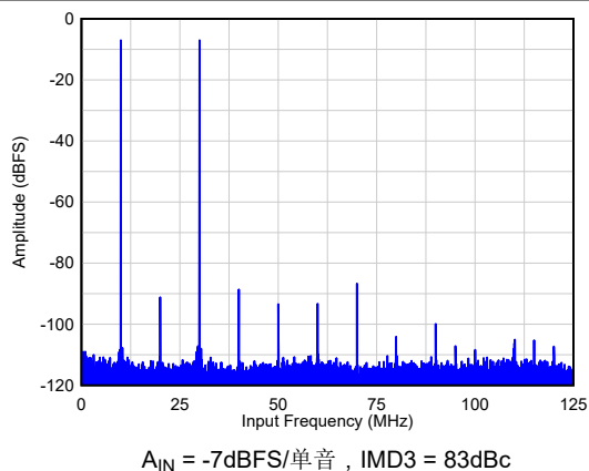
图 6-11. F_{IN} = 220\text{MHz}/240\text{MHz} 时的双音 FFT
