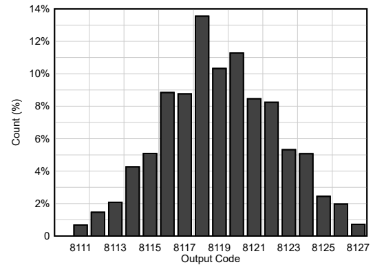
图 6-52. 直流偏移直方图
