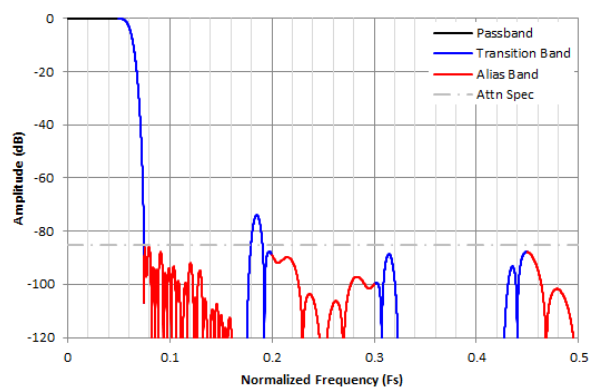
图 8-27. /8 复数抽取滤波器响应
