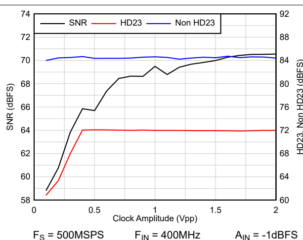
图 8-12. 交流与时钟振幅间的关系
