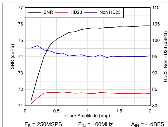
图 8-13. 交流与时钟振幅间的关系
