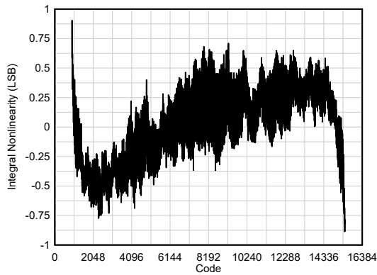
图 6-51. INL
