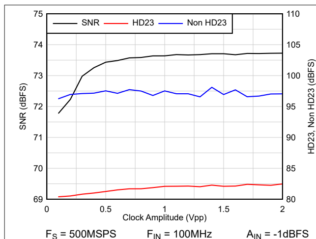
图 8-11. 交流与时钟振幅间的关系
