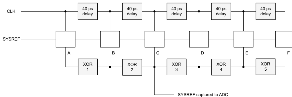
图 8-17. SYSREF 检测电路
