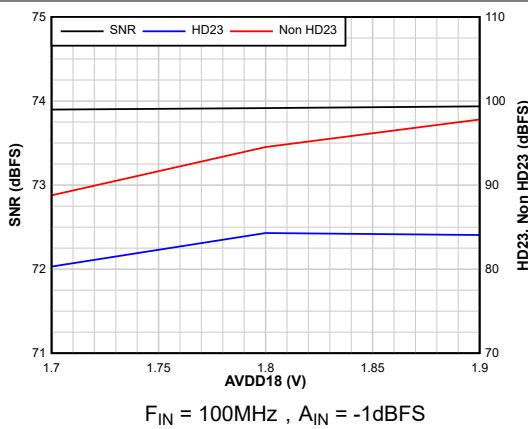
图 6-19. 交流性能与 AVDD18 间的关系
