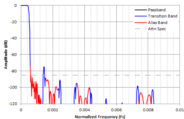
图 8-41. /1024 复数抽取滤波器响应
