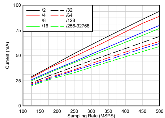
图 6-54. 电流与采样率间的关系
