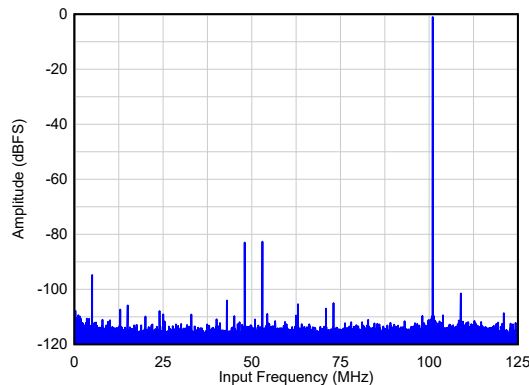
图 6-2. F_{IN} = 101\text{MHz} 时的单音 FFT
