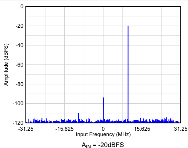
图 9-7. FFT4 : /8 抽取
