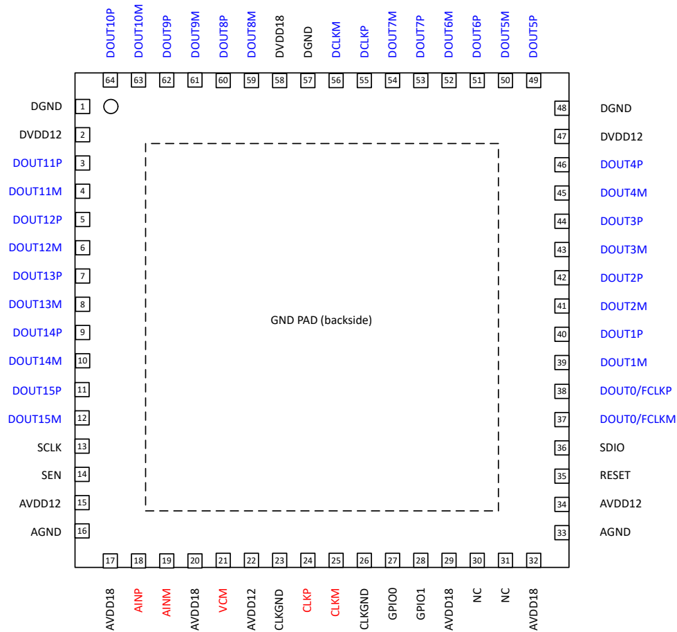
图 5-1. RTD 封装、64 引脚 VQFN (顶视图)
