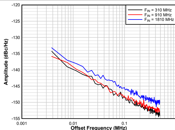
图 8-10. 振幅噪声示例
