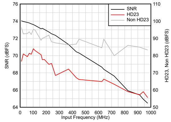
图 6-40. 交流性能与 F_{IN} 间的关系
