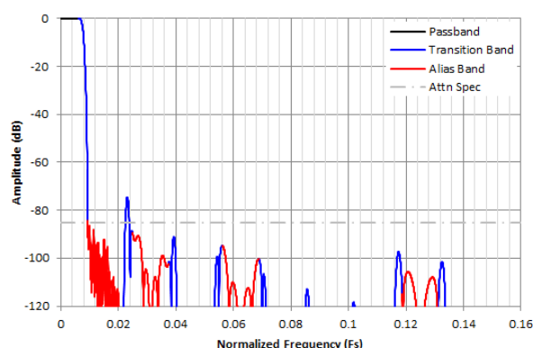
图 8-33. /64 复数抽取滤波器响应
