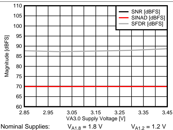
图 16. SNR, SINAD, SFDR vs VA3.0 Supply
