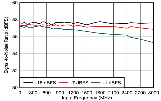
图 5-99. SNR vs Input Frequency
