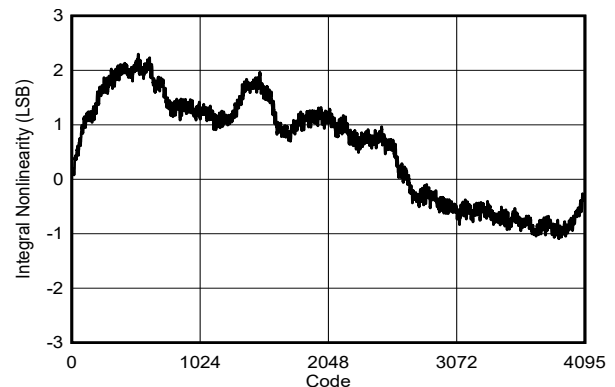
图 5-265. INL vs Code
