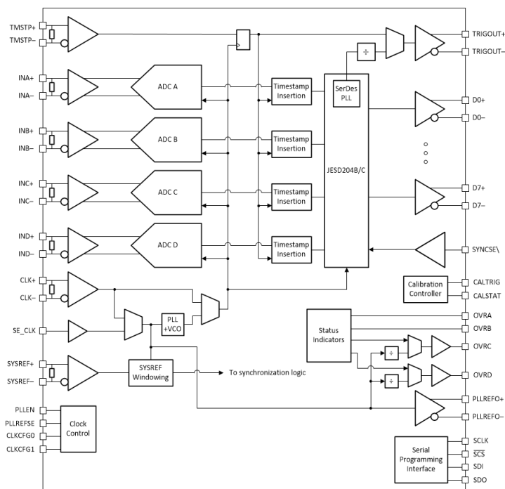
四通道器件方框图
