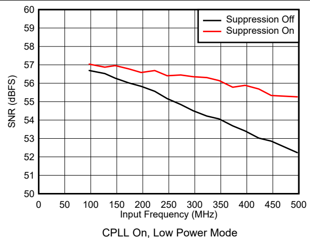
图 7-60. SNR vs Input Frequency
