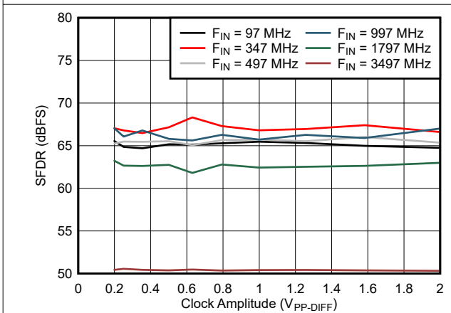
图 5-41. SFDR vs Clock Amplitude
