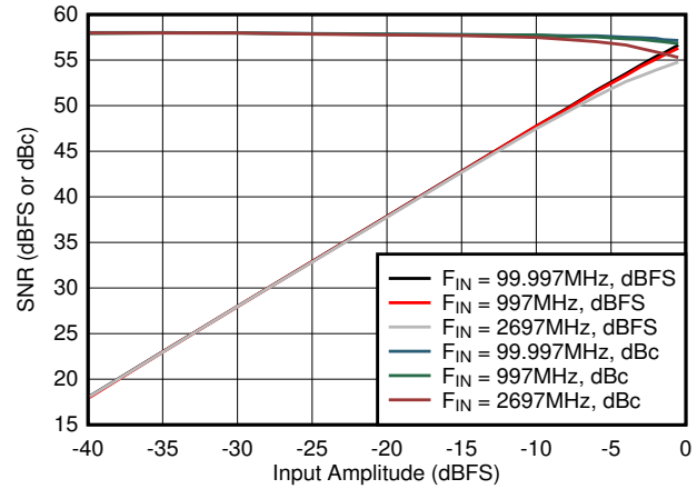
图 7-32. SNR vs Input Amplitude
