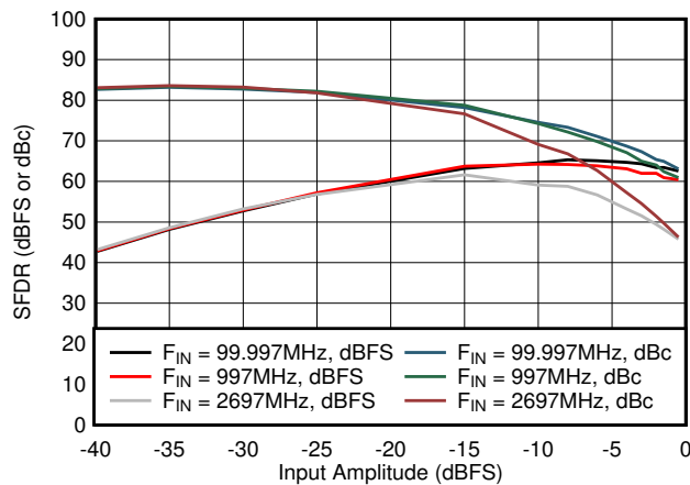
图 7-33. SFDR vs Input Amplitude
