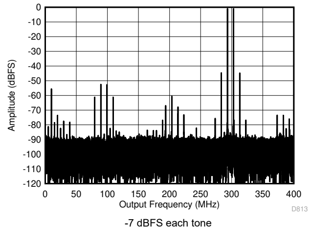
图 7-68. Two Tone FFT at 3498 MHz
