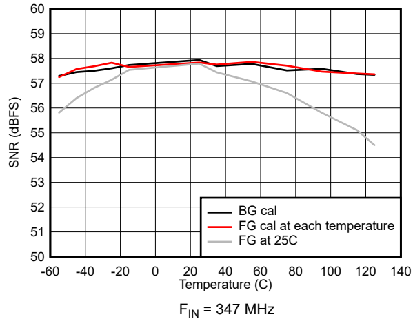
图 7-43. SNR vs Temperature
