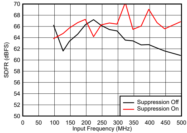
图 7-61. SFDR vs Input Frequency
