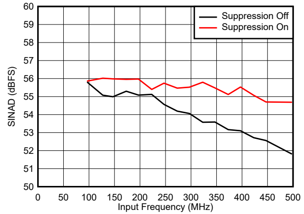
图 7-62. SINAD vs Input Frequency
