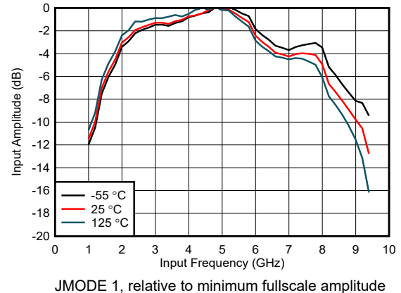
图 6-2. DES Mode: Input Amplitude vs Input Frequency
