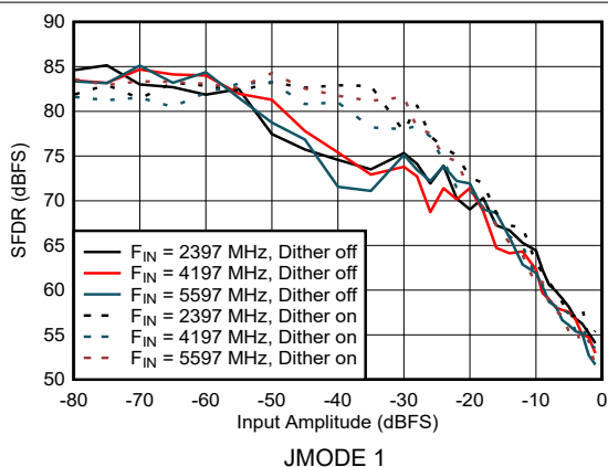
图 6-15. DES Mode: SFDR vs Input Amplitude
