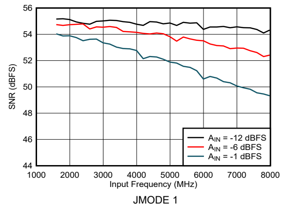
图 6-8. DES Mode: SNR vs Input Frequency
