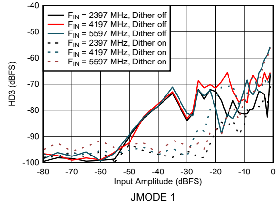
图 6-18. DES Mode: HD3 vs Input Amplitude
