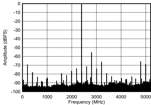
图 8-2. FFT for 2397 MHz Input Signal, 10.4 GSPS, JMODE1
