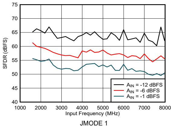
图 6-9. DES Mode: SFDR vs Input Frequency
