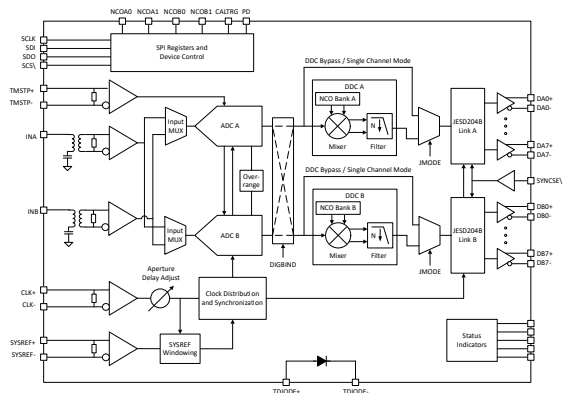
ADC12DJ5200SE 方框图
