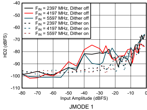
图 6-17. DES Mode: HD2 vs Input Amplitude
