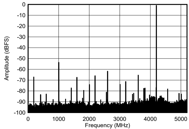
图 8-3. FFT for 4197 MHz Input Signal, 10.4 GSPS, JMODE1
