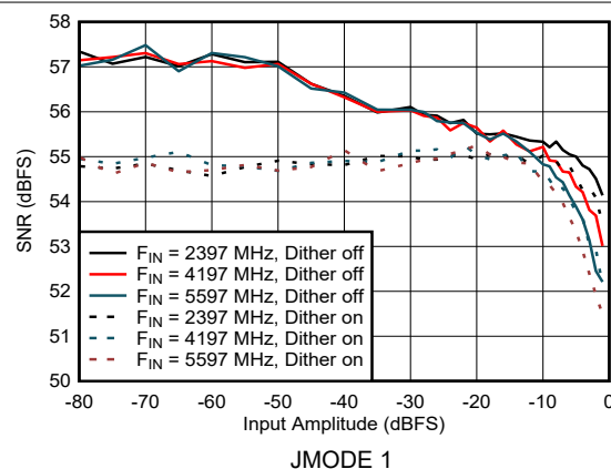
图 6-14. DES Mode: SNR vs Input Amplitude
