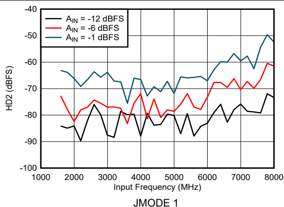
图 6-11. DES Mode: HD2 vs Input Frequency
