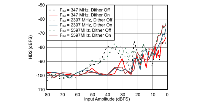
图 6-60. DES Mode: HD2 vs Input Amplitude and Dither
