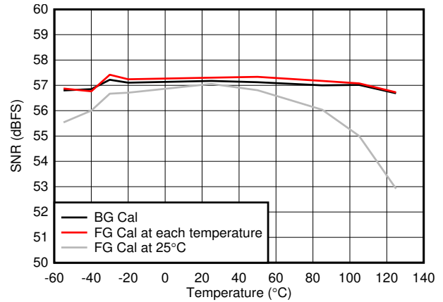
图 6-64. SNR vs Temperature
