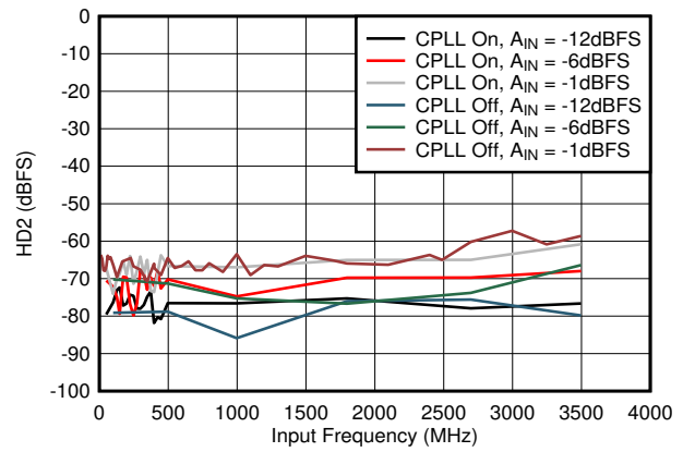
图 6-52. HD2 vs A_{IN} and C-PLL
