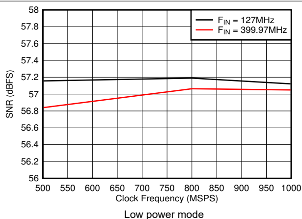
图 6-28. SNR vs Sample Rate
