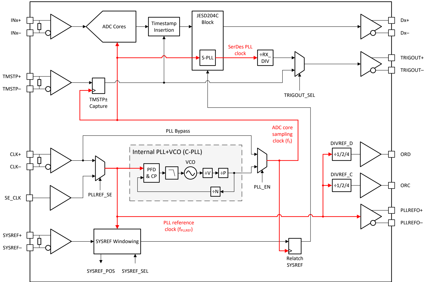
图 7-5. Clocking Subsystem
