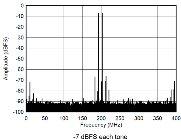
图 7-53. Dual Tone FFT at 1798 MHz
