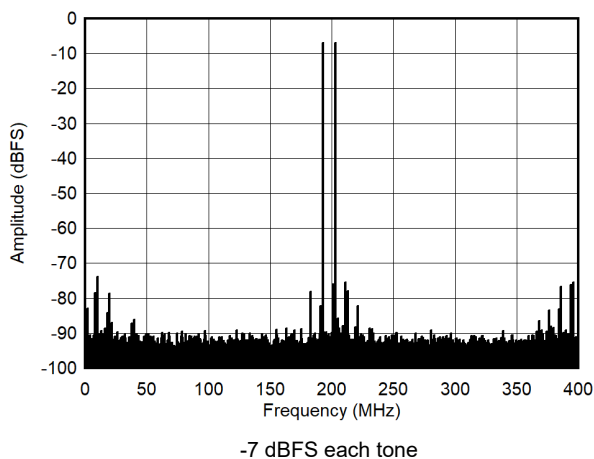
图 7-52. Dual Tone FFT at 998 MHz
