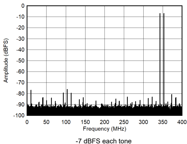
图 7-51. Dual Tone FFT at 348 MHz
