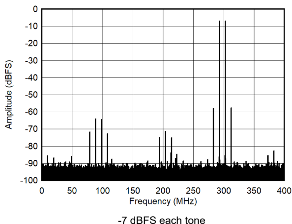
图 7-54. Dual Tone FFT at 2698 MHz
