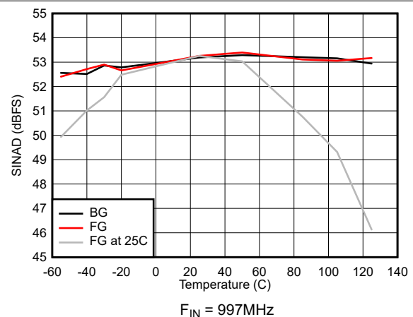
图 7-36. SINAD vs Temperature
