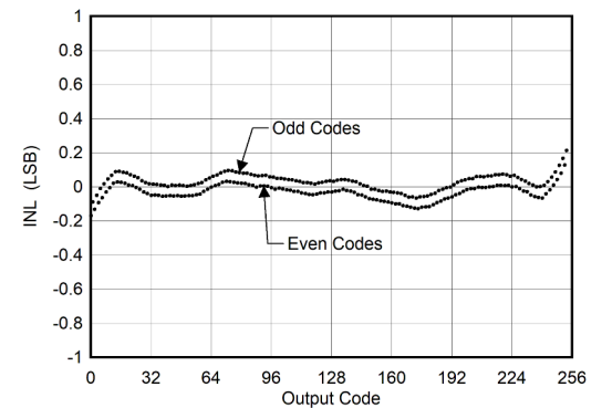
图 5-4. INL vs ADC Code
