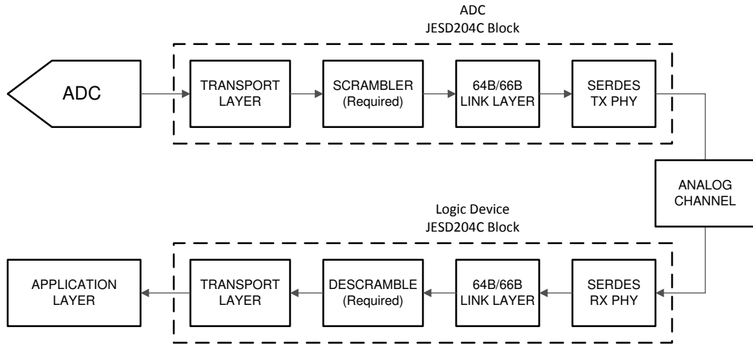
图 6-9. Simplified 64B/66B Encoded JESD204C Interface Diagram
