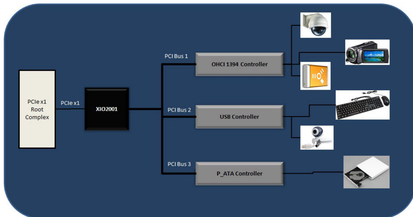
典型示意图
