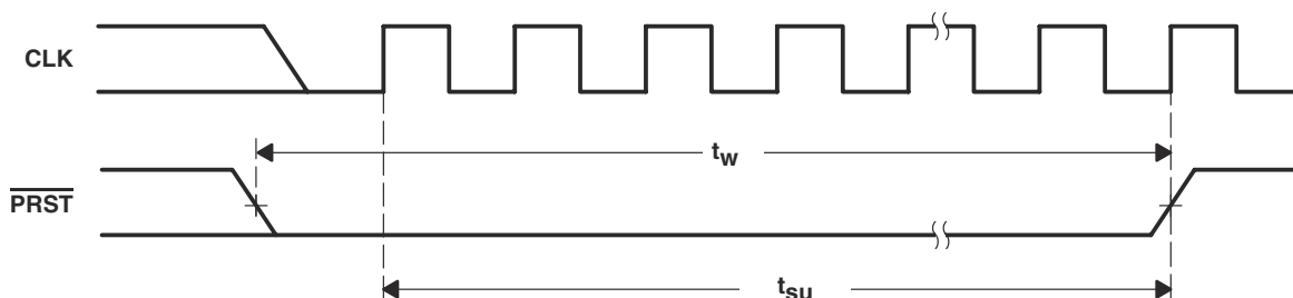
图 7-3. PRST Timing Waveforms
