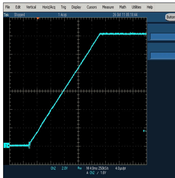
图 10-11. V OUT Soft Start
