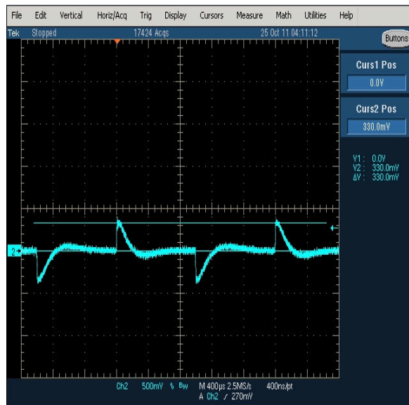
图 10-10. Load Transient
