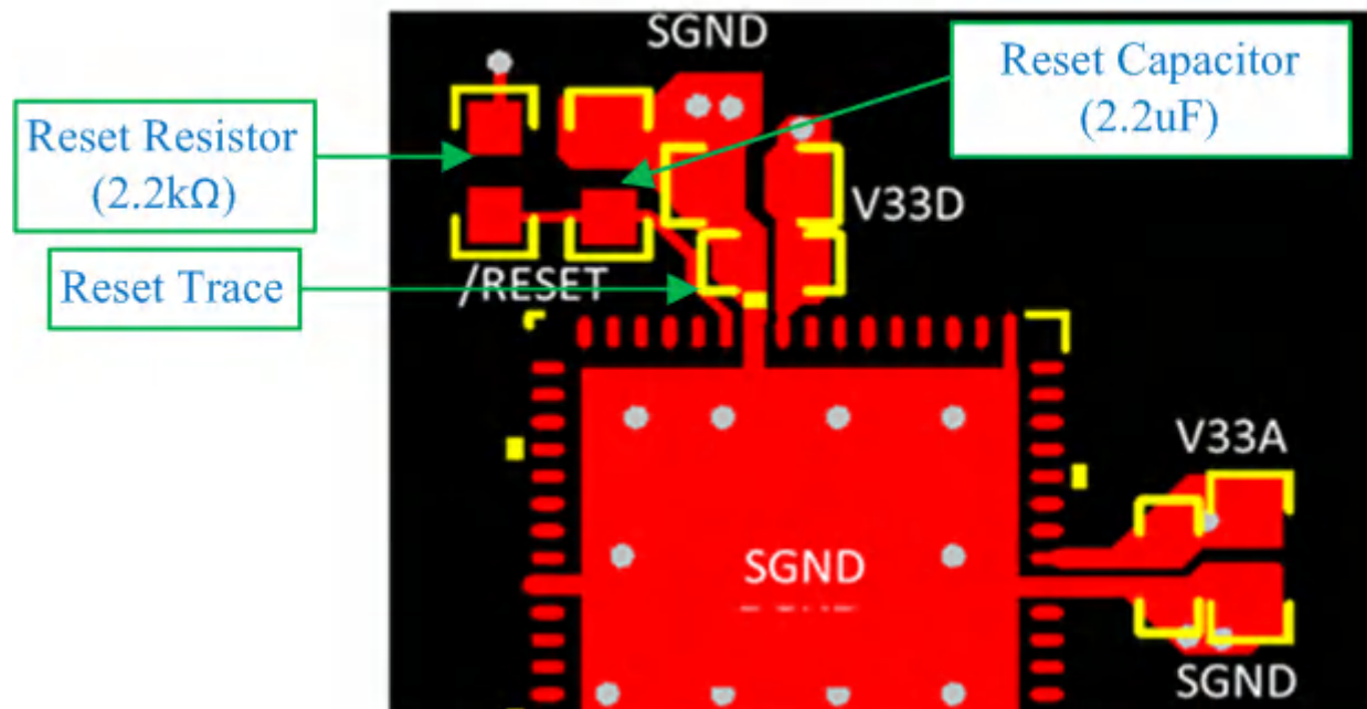
图 12-6. RESET Pin Connection
