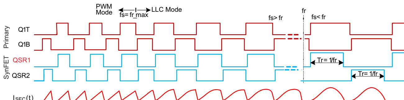
图 9-6. LLC Waveforms
