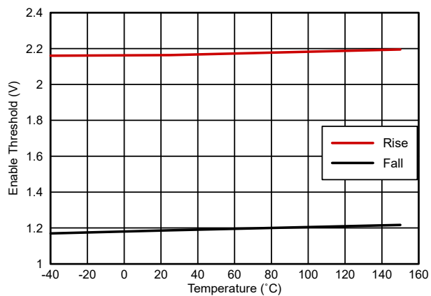
图 5-12. 使能阈值
