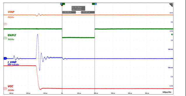
图 6-16. 输出短路运行 : VINP = 5.0V
