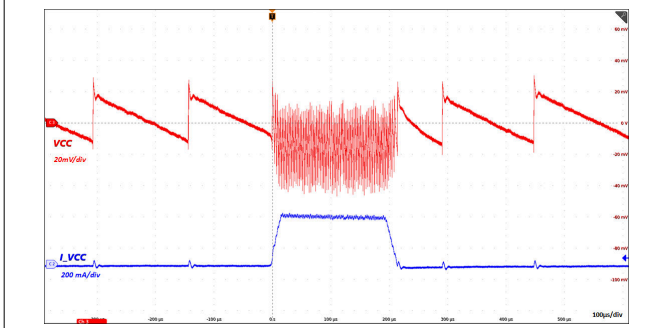
图 6-15. 负载瞬态 : VINP = 5.0V , VCC = 5.0V , C OUT2 = 22 μF , I VCC = 0mA - 300mA - 0mA
