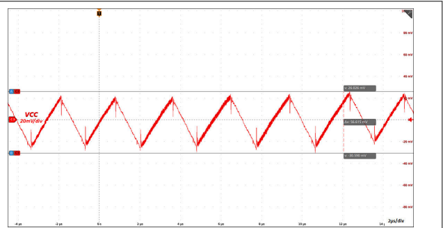
图 6-14. 稳态输出电压纹波 : VINP = 5.0V , VCC = 5.0V , 300mA 负载
