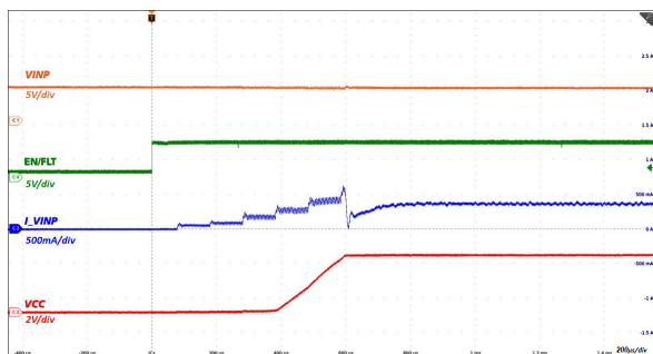
图 8-3. 通过 EN/FLT 从低电平到高电平启动 : VINP = 5.0V , VCC = 3.3V , 11Ω 负载
