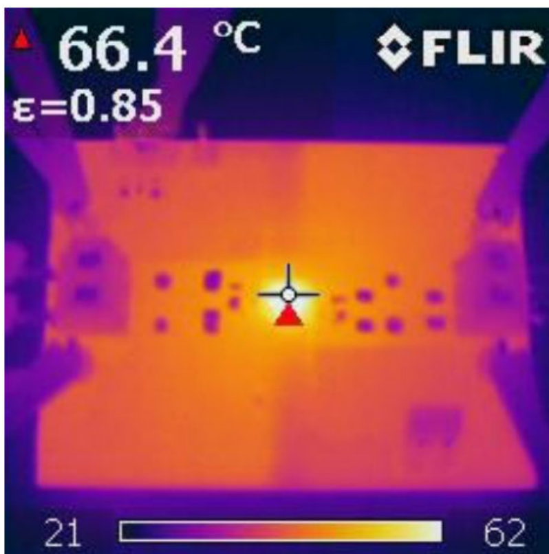
图 8-2. UCC33410 热像图 : VINP = 5.0V , VCC = 3.3V , P_{Out}=1.0W
