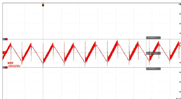
图 8-4. 稳态输出电压纹波 : VINP = 5.0V , VCC = 3.3V , C OUT2 = 22 μF , 300mA 负载
